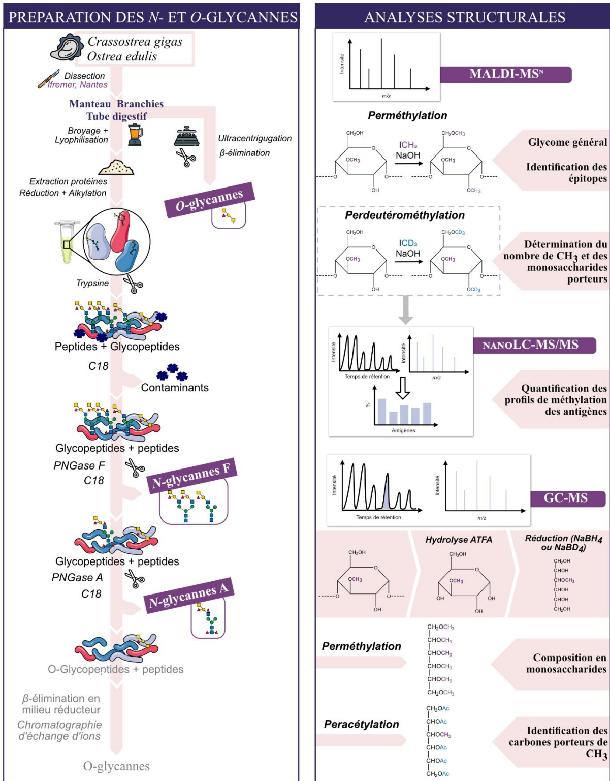
Figure 42 : Méthodologie employée pour les analyses structurales des N -et O -glycannes obtenus à partir des branchies, tubes digestif et manteaux des huîtres C. gigas et O. edulis . Crédits icones : Flaticon.com analyse par spectrométrie de masse MALDI-QIT-TOF. Après action de la PNGase A, les N -glycannes A ont été séparés des peptides et O -glycopeptides potentiels par SPE sur cartouche C 18 . En effet, dans le cas de la présence de O -glycosylprotéines dans les tissus testés, nous devons obtenir à l'issue de la SPE
