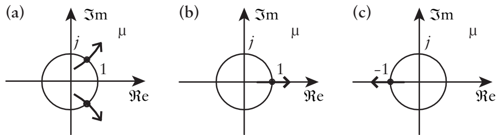
Figure 7 — Différents types d'instabilités identifiés
