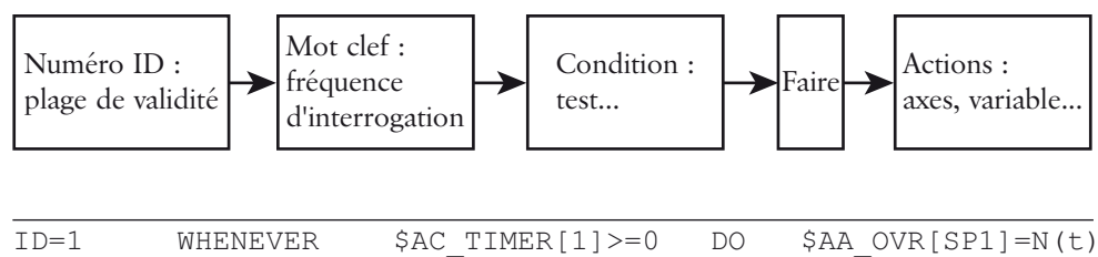
Figure 98 – Programmation d'une action synchrone sous la Siemens 840D
