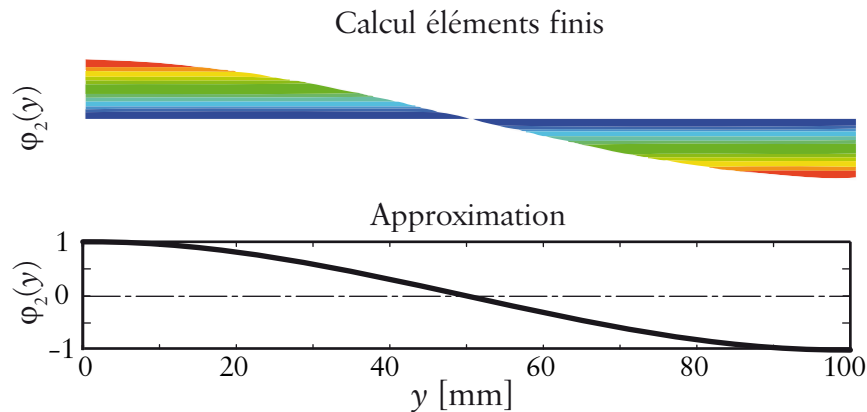
Figure 49 – Déformée modale du deuxième mode
