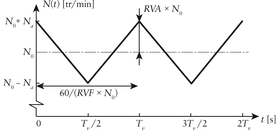
Figure 68 – Consigne de type triangulaire
