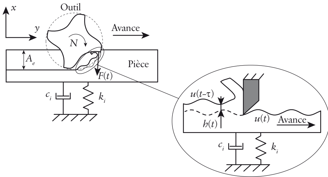
Figure 50 – Modélisation de la régénération de la surface
