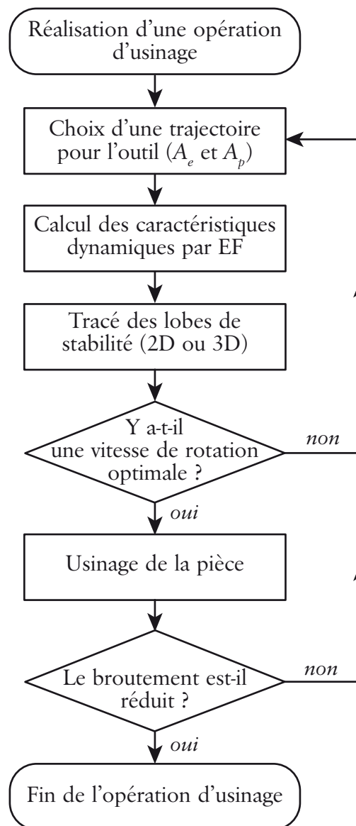
Figure 21 – Organigramme d'optimisation
