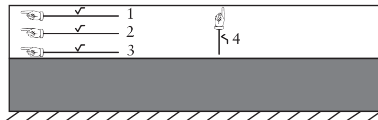
Figure 61 – Direction de mesure de la rugosité
