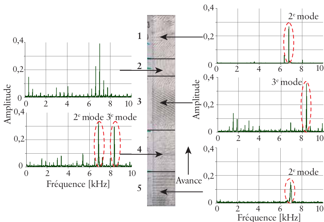
Figure 66 — Fréquences mesurées pour l'usinage à 20 500 tr/min
