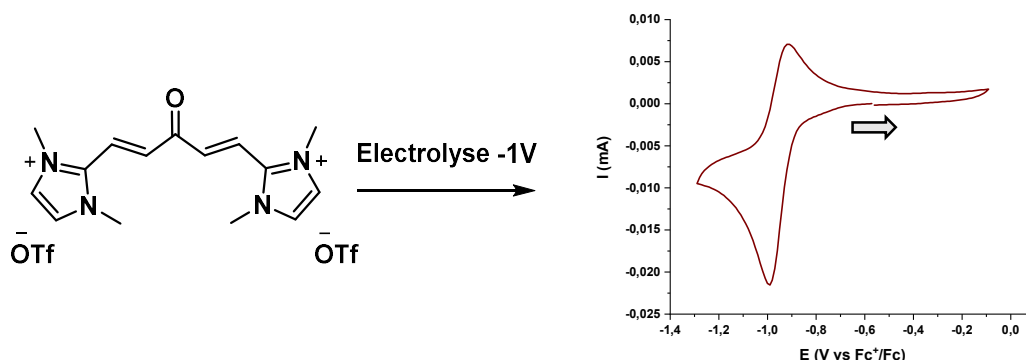
Schéma 2-11 : Courbe de voltampérométrie cyclique du composé 9a^{2+} enregistré après électrolyse à -1,0 V. Vitesse de balayage \nu = 100 mV \cdot s^{-1} . [C] = 1 mM avec TBAPF_6 à 0,1 M dans l'acétonitrile.
