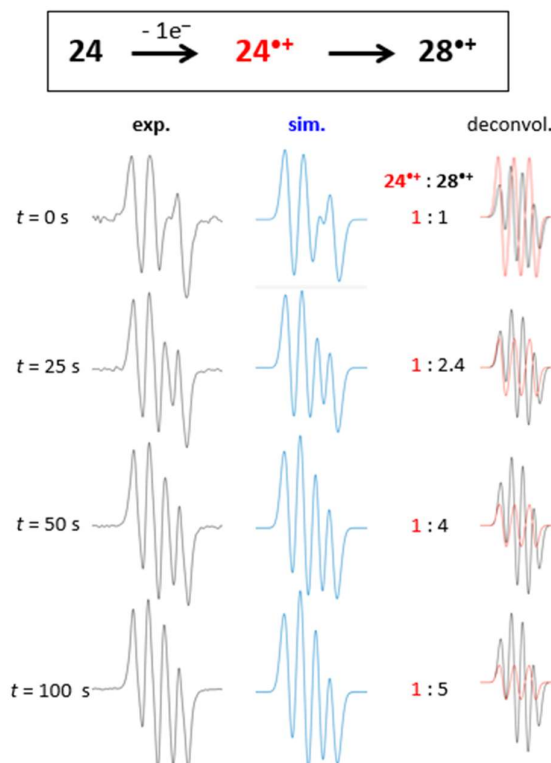
Figure 3-9 : Gauche, spectre RPE de l'électrolyse de 24 à 0,4 V dans l'acétonitrile ; milieu, le spectre simulé correspondant ; droite, déconvolution et respective contribution de 24 *+ en rouge et 28 *+ en noir.
