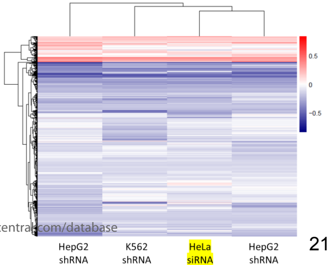
U2AF2
