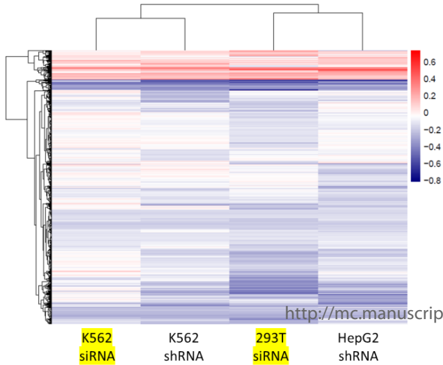
U2AF1
