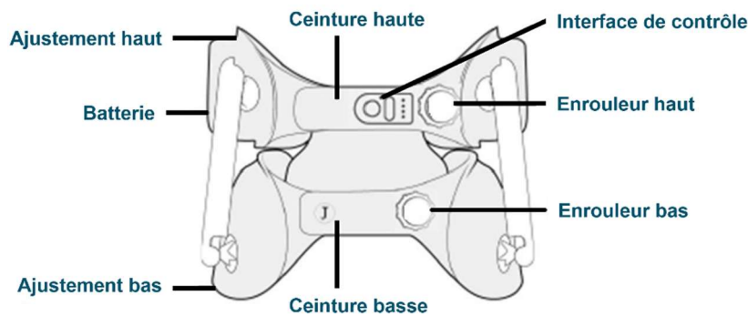
Figure 12. Schéma de l'exosquelette Japet.W.
