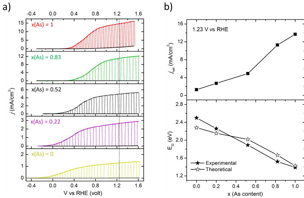
Figure III (a) Évaluation du photo-courant en fonction de la tension ( j - V ) pour les couches minces épitaxiales de 1 \mu m d'épaisseur d'alliages GaP_{1-x}As_x épitaxiées sur Si avec les différentes compositions x(As) données en insert. Le potentiel d'oxydation de l'eau (1,23 V vs RHE) est marqué par une ligne pointillée noire; (b) évolution de la densité nette de photo-courant ( j_{net} ) à 1,23 V et de la bande interdite ( E_g ) en fonction de x(As) de l'alliage GaP_{1-x}As_x
