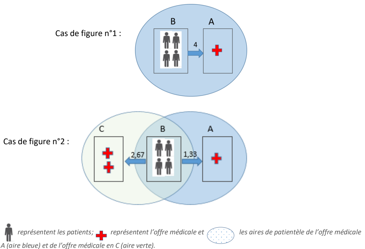
Figure 59 – Schéma explicatif de l'estimation de la demande de soins avec le 3SFCA de Luo 2014
