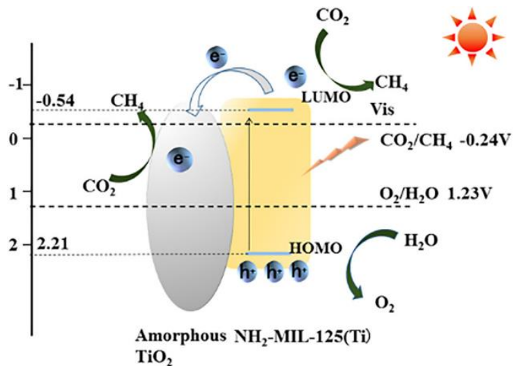
Figure 1. 22 : Représentation schématique du mécanisme proposé pour la photo-réduction du \text{CO}_2 en \text{CH}_4 en présence d' \text{H}_2\text{O} avec \text{NH}_2\text{-MIL-125(Ti)/TiO}_2 amorphe 76 .
