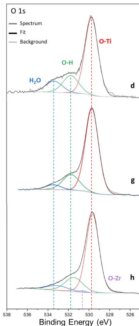
Figure III. 18 : Spectres XPS zoomés sur les orbitales O 1s (d) de TiO 2 (P25), (g) de TiO 2 /1% m. Au et (h) de [TiO 2 /1% m. Au]/5% m. NH 2 -UiO-66.
