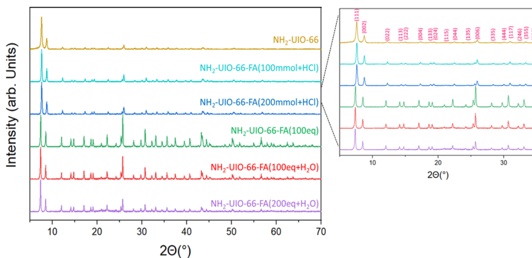
Figure IV. 2 : Diffractogrammes des rayons-X des différents MOF NH 2 -UiO-66 modifiés.
