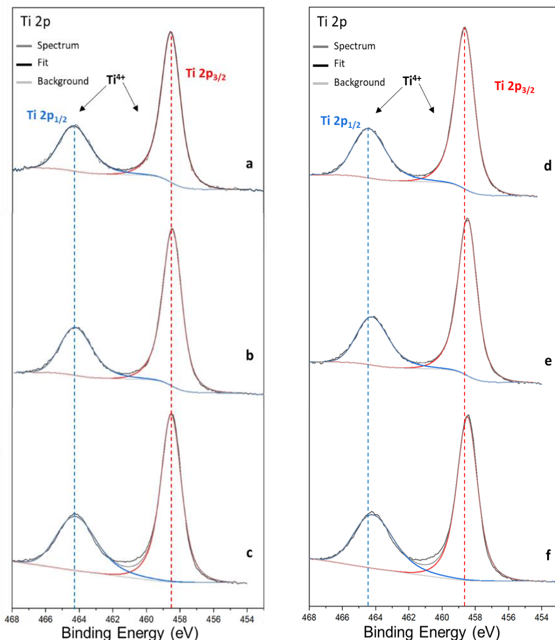
Figure III. 16 : Spectres XPS zoomés sur les orbitales Ti 2p (a) de TiO 2 (P25), (b) de TiO 2 /1% m. Au, (c) de [TiO 2 /1% m. Au]/5% m. NH 2 -UiO-66, (d) de 5% m. NH 2 -UiO-66/TiO 2 , (e) de [5% m. NH 2 -UiO-66/TiO 2 ]/1% m. Au et (f) de 20% m. [NH 2 -UiO-66/5% m. Au]/TiO 2 .
