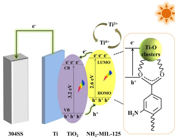
Figure 1. 23 : Représentation schématique proposée pour les transferts de charges au sein de \text{NH}_2\text{-MIL-125(Ti)/TiO}_2 , appliquée à la protection photo-cathodique contre la corrosion 94 .
