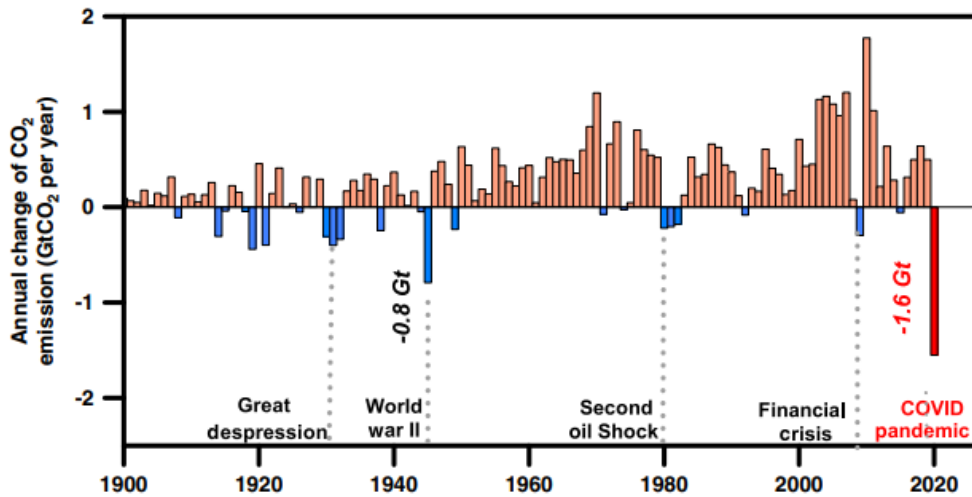
Figure 4 : Changements annuels des émissions de CO 2 depuis 1900 jusqu'en 2020 10 .
