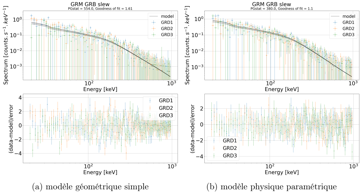
FIGURE 5.10 – Spectres en coups d'un sursaut gamma moyennement fluent vu par les trois GRDs du GRM, ajustés avec XSPEC, pour un modèle de fond géométrique simple (a), et un modèle physique paramétrique (b). Voir la figure 5.5 pour le détail des panneaux.
