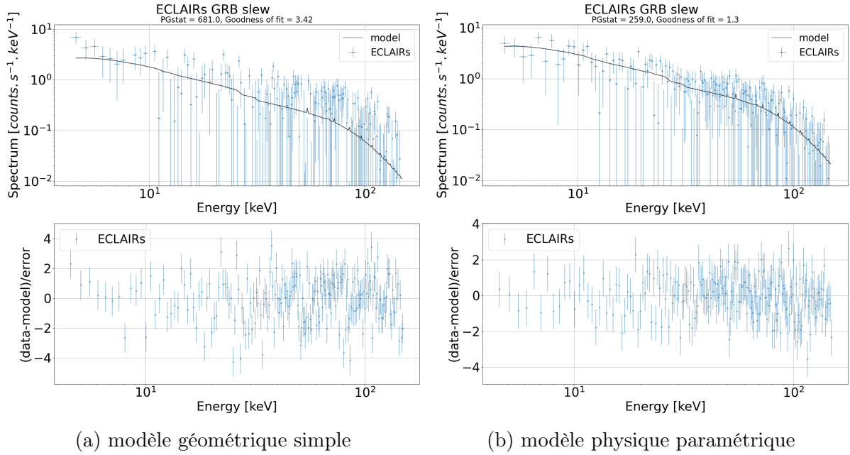
FIGURE 5.9 – Spectre en coups d'un sursaut gamma moyennement fluent vu par ECLAIRs et ajusté avec XSPEC, pour un modèle de fond géométrique simple (a), et un modèle physique paramétrique (b). Les panneaux du haut montrent le spectre en coups et le modèle du sursaut ajusté (courbe noire). Les panneaux du bas illustrent les résidus entre le modèle et les données où \chi = \frac{y-m}{\Delta y} , avec y les données simulées et m le résultat du modèle ajusté.
