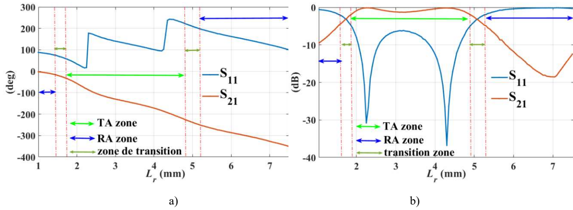
Fig.4.5 Les paramètres S simulés de la PC avec des guides d'ondes ouverts ( h=10 mm, \text{pas}=0,05 mm, f=20 GHz, polarisation x, \phi_{\text{inc}}=90^\circ , \theta_{\text{inc}}=25^\circ ). a) Phase. b) Amplitude.
