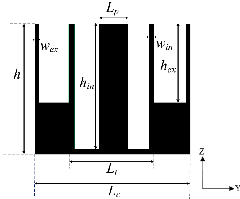
Fig.5.1 Cellule bi-bande proposée (vue en coupe).
