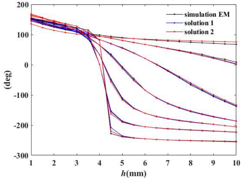
Fig.2.9 Phase réfléchie
