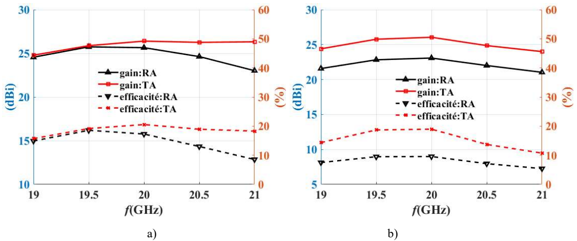
Fig.4.7 Gain et efficacité de surface. a) TRA1. b) TRA2.
