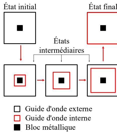
Fig.2.5 Le mécanisme de variation de la PC 3D (vue de dessus).
