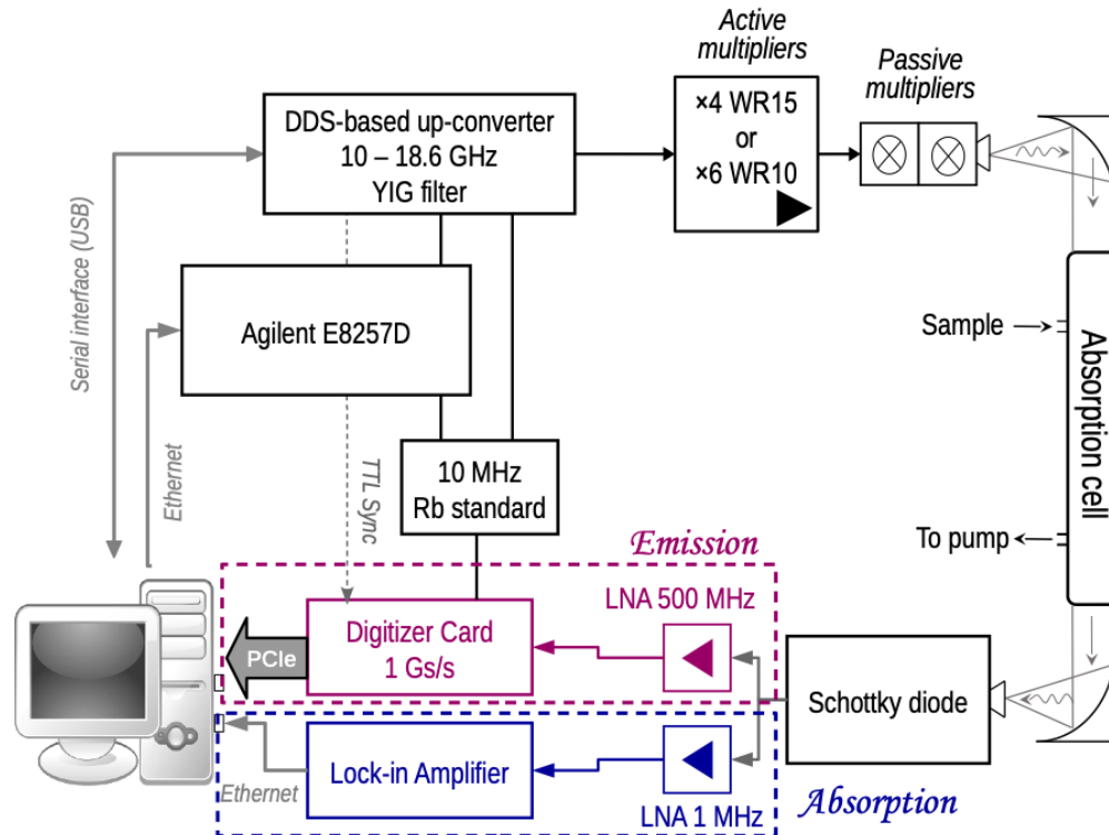
FIGURE 2.9 – Schéma du spectromètre millimétrique du PhLAM. Crédit : L. Zou.
