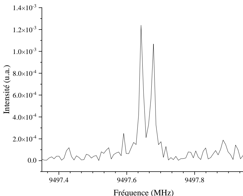
FIGURE 4.8 – Enregistrement de la transition 2_1 \leftarrow 1_0 ( N''_{j''} \leftarrow N'_{j'} ) du butadienyl à 9497,613 MHz réalisé sur le SIMO2 avec une résolution 16 kHz après moyennage sur 100 acquisitions. V_d = 1500 V, I_{lim} = 50 mA, délai = 15 \mu s, T_1 = 800 \mu s, T_2 = 400 \mu s, f = 1 Hz et T_7 = 1000 \mu s, P = 5 bar avec une sensibilité de 100 mV.
