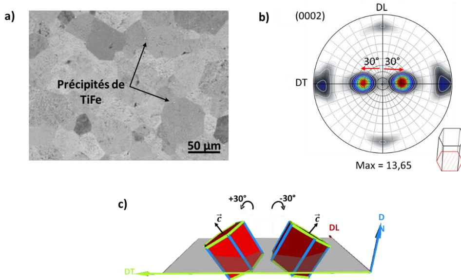
Figure 48: Micrographie MEB de la section transverse du feillard T40 (a), figure de pôle directe (0002), recalculée par la logicielle ATEX, obtenue par DRX à la surface du feillard T40 et schéma simplifié de l'orientation des grains \alpha en surface du feillard (c).
