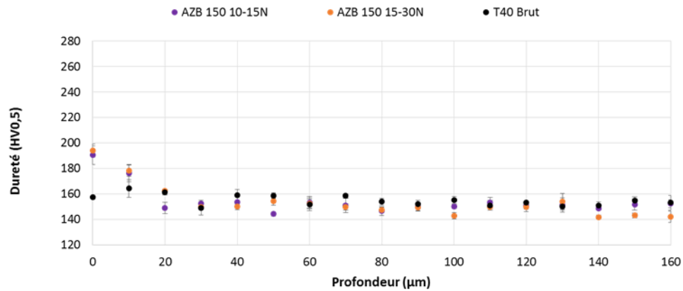
Figure 118: Profils de microdureté des échantillons grenailés avec le média AZB150 et une IA F10-15N et F15-30N ainsi que celui du T40 brut.
