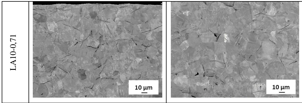
Figure 113: Micrographies MEB (contraste BSE) de la coupe transverse des feuillards LS10-1, LA10-0,9, LA10-0,77 et LA10-0,71 hydrurés à 250°C pendant 500 heures dans un autoclave contenant de l'eau déminéralisée et 1,5 bar de dihydrogène.
