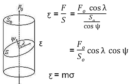
Figure 8: Loi de Schmid et Boas accompagnée d'un schéma [54]
