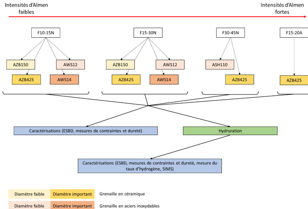
Figure 116: Plan d'expérience qui est réalisé pour le grenailage du feuillet T40
