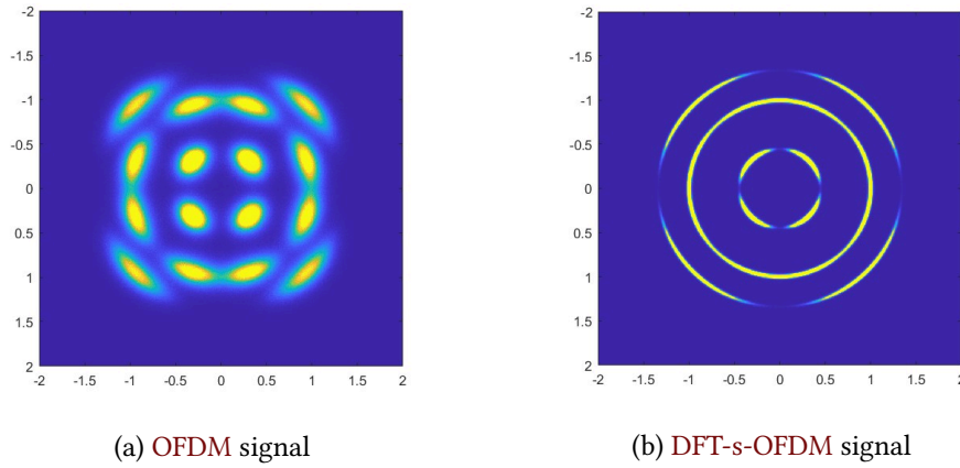
Figure A.4: Effets du PN sur les différents signaux reçus en considérant les paramètres dans le tableau 2.4 .
