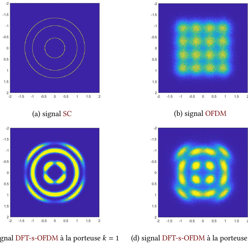
Figure A.8: Effets du PN Gaussien (GPN) sur divers signaux utilisant de la 16-QAM avec un SNR = 50 dB
