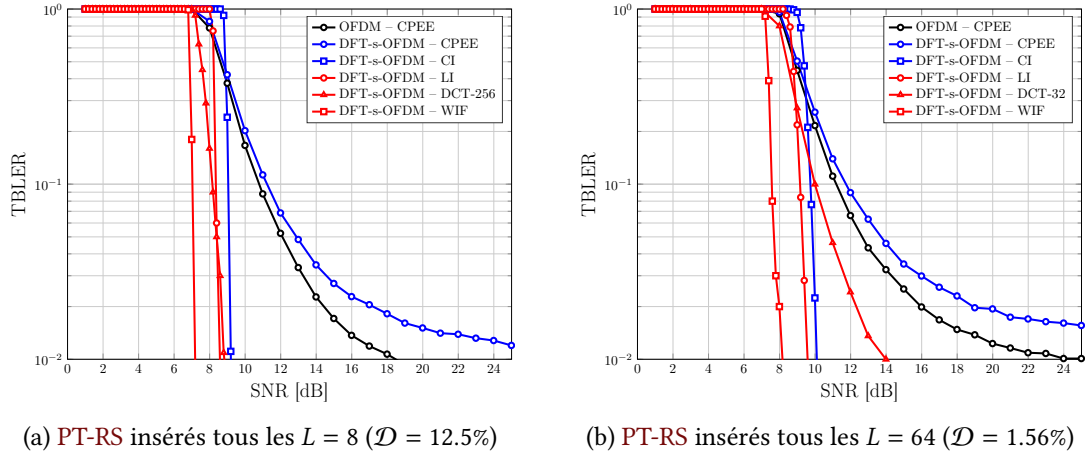
Figure A.5: Comparaison des performances entre l'OFDM et la DFT-s-OFDM en considérant le schéma de PT-RS distribué. Le modèle de PN considéré est celui du 3GPP dans figure A.3b.
