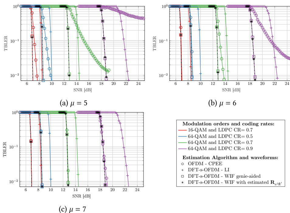
Figure A.6: Performances de la DFT-s-OFDM et de l'OFDM en terme de TBLER en fonction du SNR. Les numerologies \mu = \{5, 6, 7\} et le modèle de PN proposé par le CEA sont considérés.
