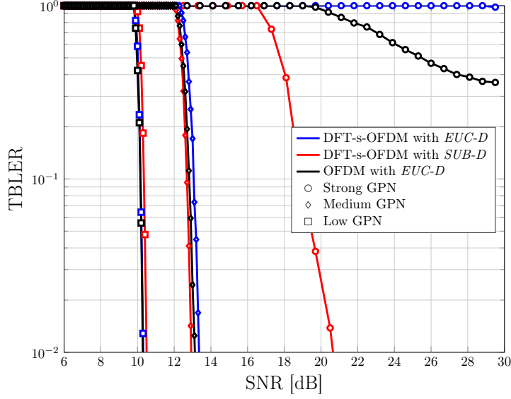
Figure A.9: Performance OFDM vs DFT-s-OFDM: TBLETR en fonction du SNR pour une modulation 16-QAM avec N_s = 480 , N_f = 512 et CR=0.7 .
