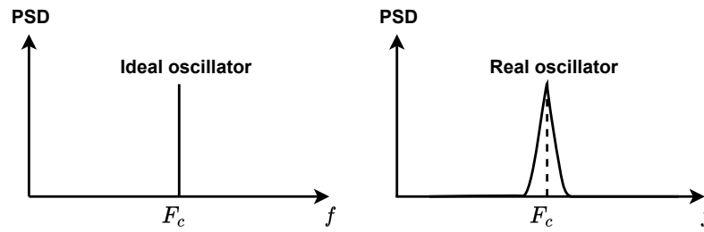
Figure A.2: Densité spectrale de puissance (PSD) de la réponse fréquentielle d'un oscillateur idéal (ideal) vs. oscillateur réel (real)
