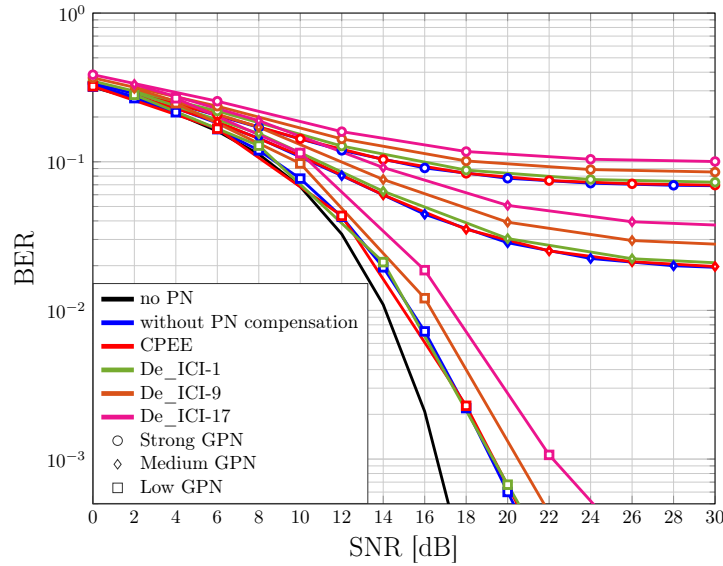
Figure A.10: Performance d'un système OFDM: le taux d'erreur binaire non codé (BER) en fonction du SNR pour une modulation 16-QAM, N_s=480 et N_f=512 .
