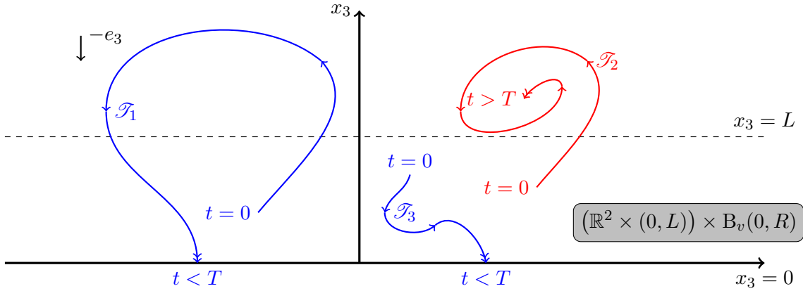
Figure 1.2: \text{EGC}_T(L, R) non satisfaite (trajectoire \mathcal{F}_2 non absorbée avant t = T )
