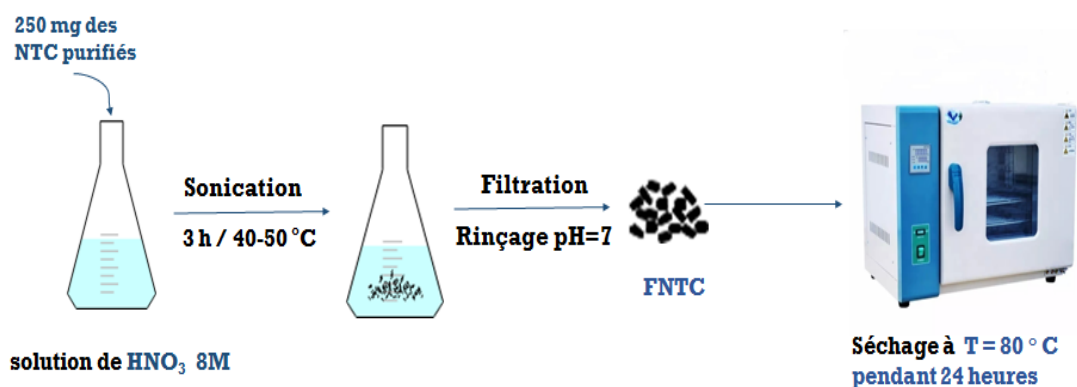
Figure 2-2: Représentation schématique de la fonctionnalisation des NTC.
