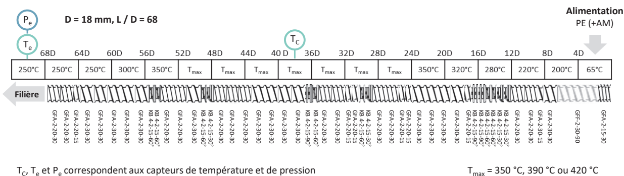
Figure II-8. Profils de vis et de températures utilisés pour la dégradation et la fonctionnalisation de polyéthylène par extrusion à très hautes températures
