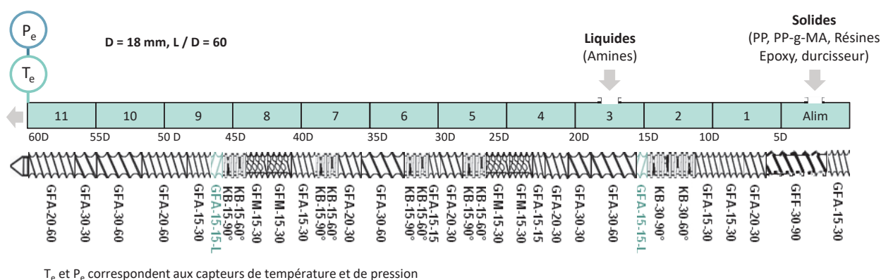
Figure II-6. Profil de vis utilisé pour la dispersion d'une phase thermdurcissable réticulée in situ dans une matrice polypropylène
