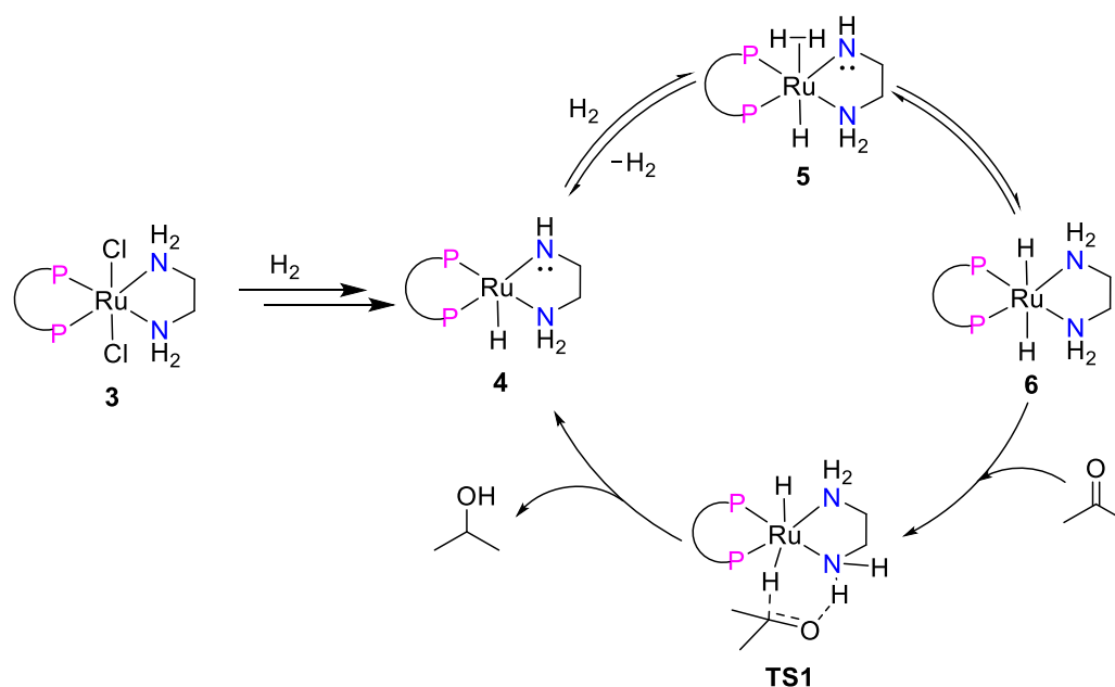
Schéma 4. Mécanisme proposé pour les complexes à base de Ru-NH dans l'hydrogénation catalysée des cétones. [47,48]
