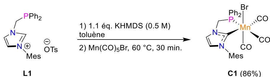
Schéma 11. Synthèse du complexe NHC-phosphine de Mn C1 à partir du pré-ligand L1 .
