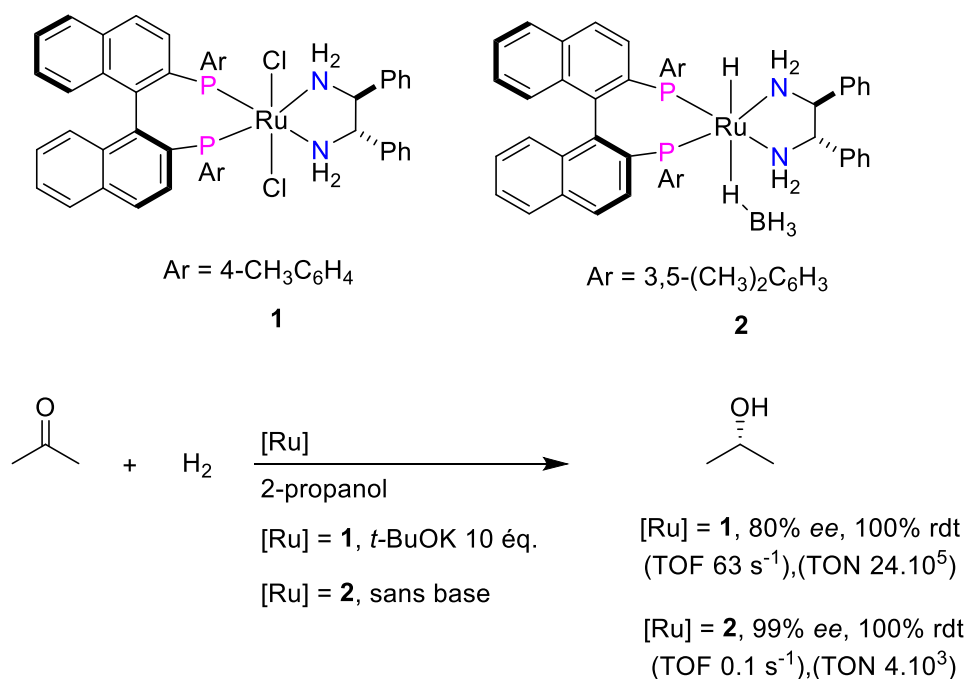
Schéma 3. Complexes de Ru-NH chiraux hautement actifs pour l'hydrogénation asymétrique des cétones. [44,46]
