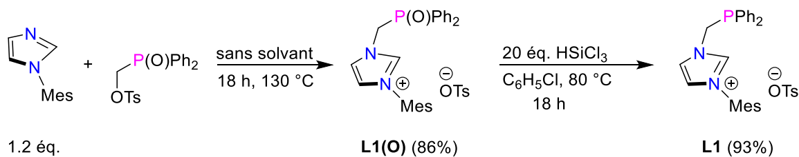
Schéma 10. Synthèse du sel de N-phosphino-imidazolium L1 à partir du 1-mésityl-imidazole.
