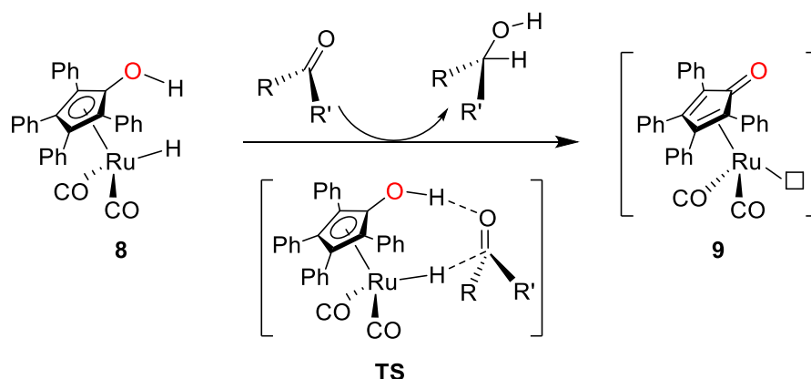
Schéma 6. Mécanisme proposé pour l'hydrogénation des dérivés carbonylés par le catalyseur de Shvo. [57]
