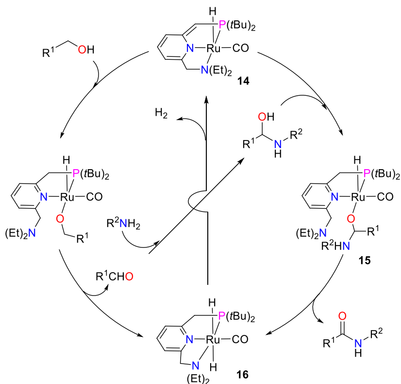
Schéma 8. Mécanisme proposé pour l'acylation déshydrogénante d'amines avec des alcools en utilisant le complexe pince PNN-Ru 14 comme catalyseur. [62]
