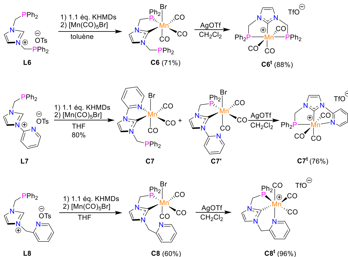
Schéma 18. Synthèses des complexes de Mn(I) cationiques tridentés à coeur NHC C6t , C7t et C8t à partir des précurseurs correspondants L6 , L7 et L8 .
