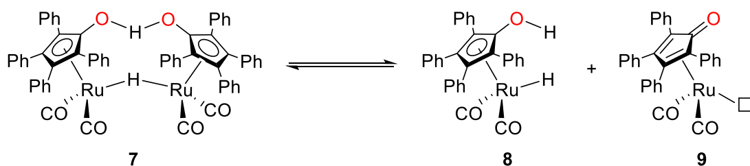
Schéma 5. Catalyseur de Shvo 7 en équilibre avec ses monomères actifs 8 et 9 . [56]
