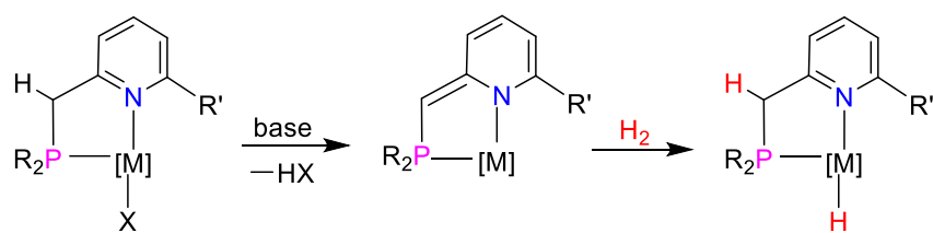
Schéma 7. Processus d'aromatisation/d'aromatisation dans les complexes de pinces de Milstein.
