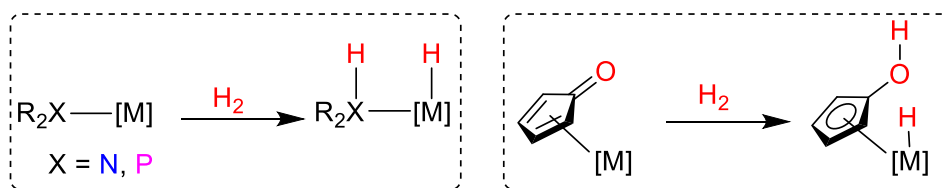
Schéma 2. Activation de H 2 par des ligands non innocents via une coopération métal-ligand.
