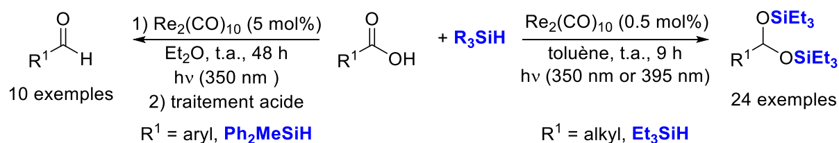
Schéma 19. Hydrosilylation des acides carboxyliques catalysée par le rhénium.
