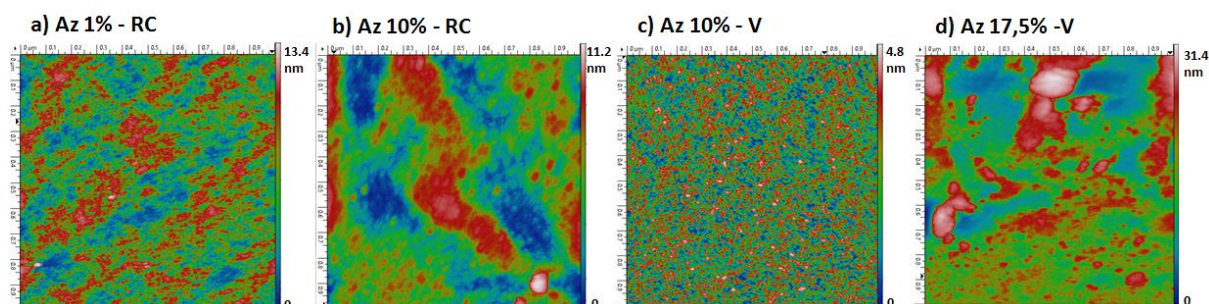
Figure 102 – Scans AFM ( 1 \times 1 \mu\text{m} ) de la surface d'échantillons greffés de protéines pour différents taux d'azotures et différentes structururations : 1% RC (a), 10% RC (b), 10% V (c) ou 17,5% V (d)
