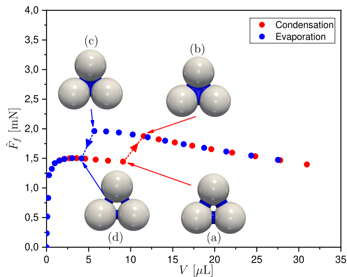
Figure A.1: L'évolution de la force capillaire \hat{F}_f [mN] en fonction du volume d'eau [ \mu\text{L} ].
