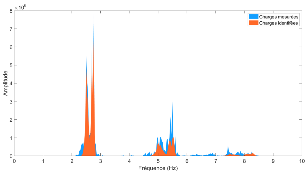
Figure 7: Comparaison des forces mesurées et des modèles de charge identifiés (cas du « skipping » sur la plante de pied)
