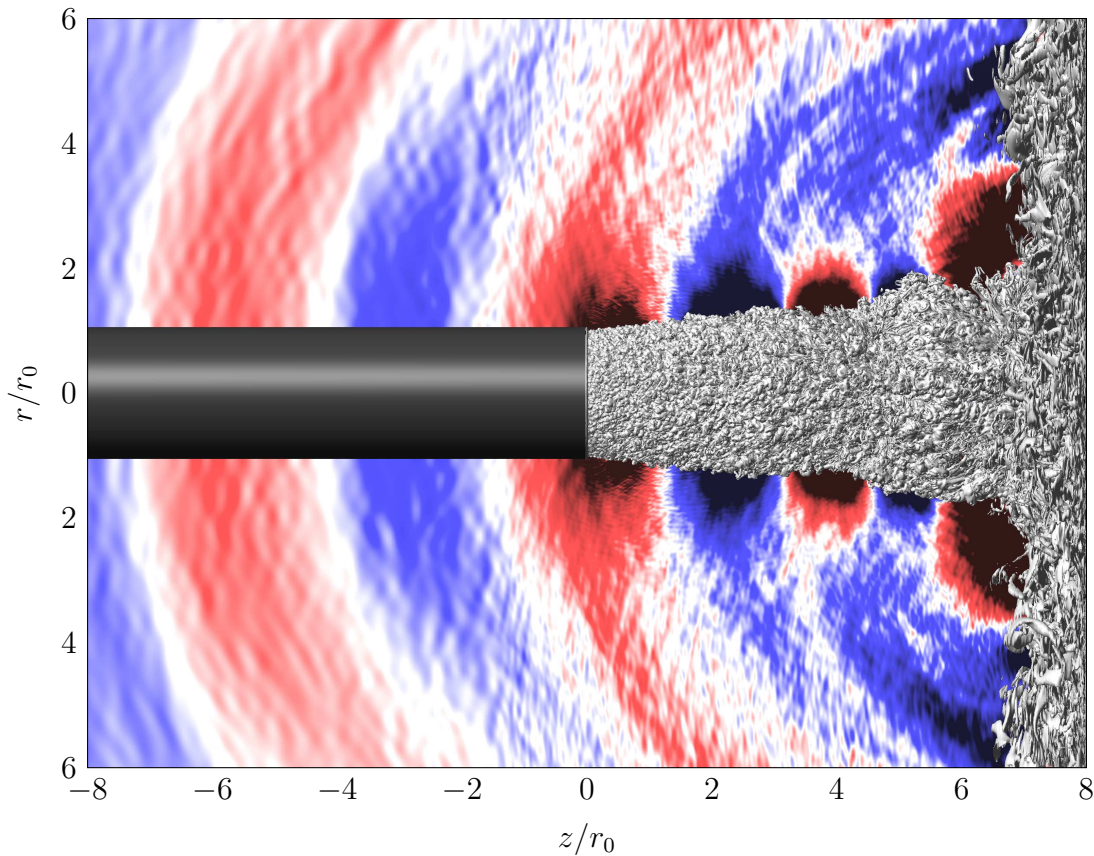
FIGURE 1.8 – Vue instantan e de l' coulement et du rayonnement acoustique d'un jet impactant   nombre de Mach de 0.9 ; (gris) isosurfaces de la norme de la vorticit  et (bleu/rouge) fluctuations de pression dans une coupe azimutale.
