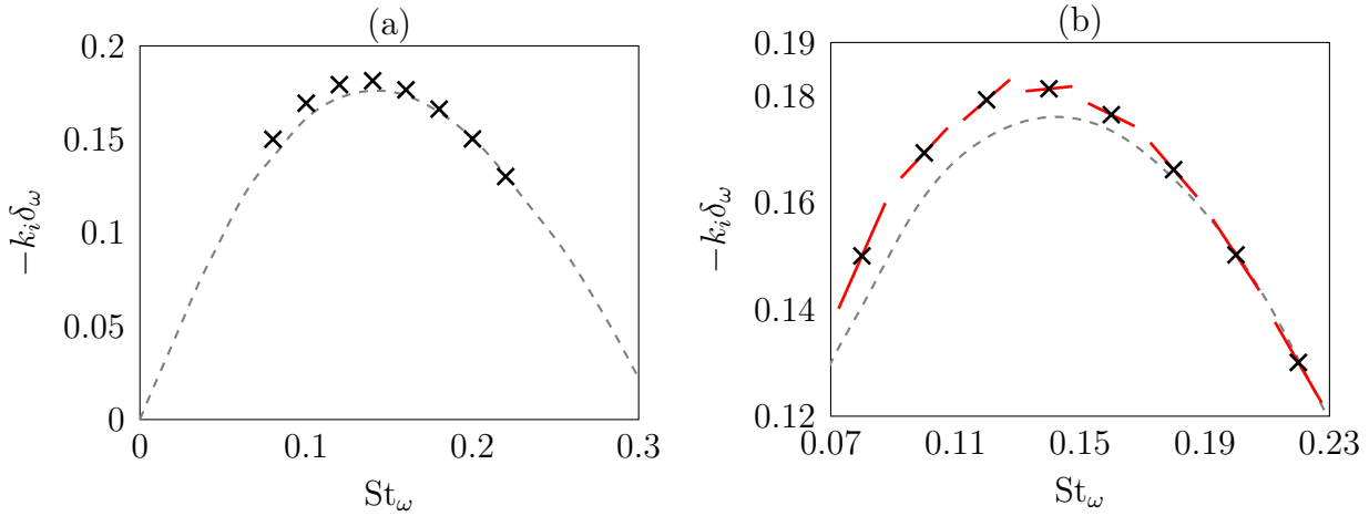
FIGURE 3.11 – Variations du taux d'amplification des ondes d'instabilité en fonction du nombre de Strouhal de l'excitation obtenues par \times les simulations et ----- l'analyse de stabilité linéaire de Monkewitz & Huerre [205]; — dérivées des taux d'amplification par rapport au nombre de Strouhal de l'excitation.
