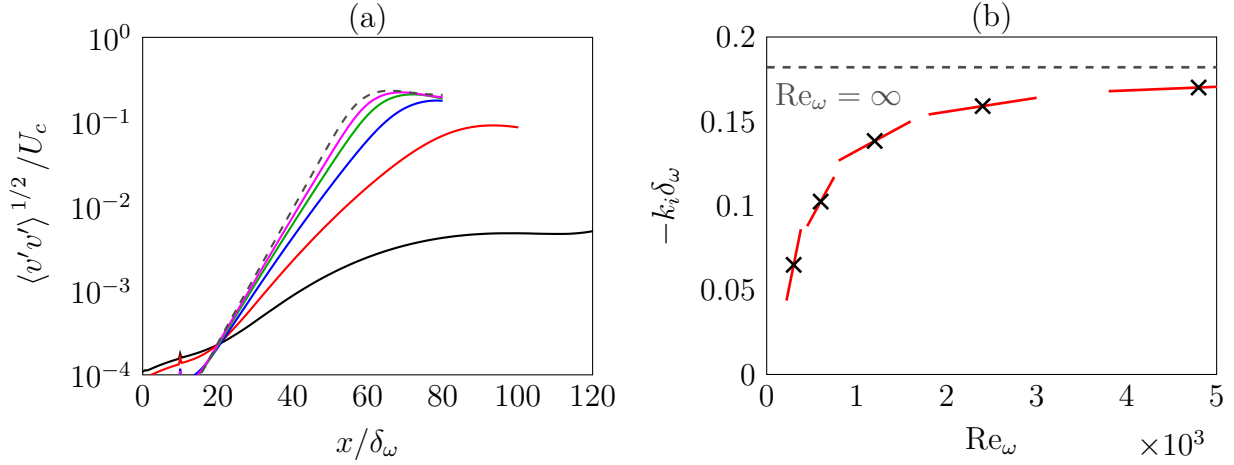
FIGURE 3.9 – Variations (a) des valeurs quadratiques moyennes des fluctuations de vitesse transverse en y = 0 pour \text{Re}_\omega = 300 , \text{Re}_\omega = 600 , \text{Re}_\omega = 1200 , \text{Re}_\omega = 2400 , \text{Re}_\omega = 4800 et \text{Re}_\omega = \infty et (b) du taux d’amplification des ondes d’instabilité et de ses dérivées en fonction du nombre de Reynolds.
