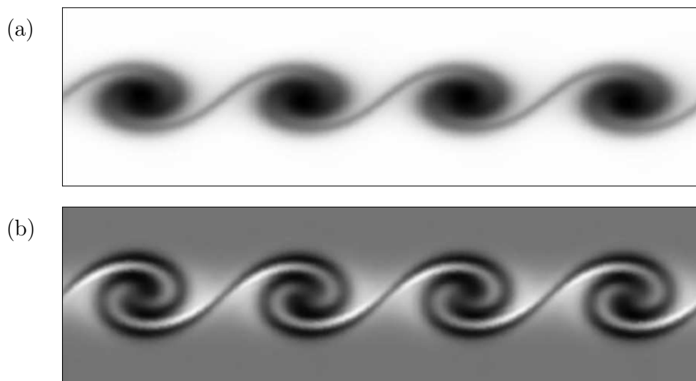
FIGURE 1.20 – Repr sentations (a) d'un champ instantan  de vorticit  et (b) de sa d riv e par rapport au nombre de Reynolds obtenus par Zayernouri & Metzger [337] en appliquant la m thode de l' quation aux sensibilit s   un  coulement de couche de m lange bidimensionnel.
