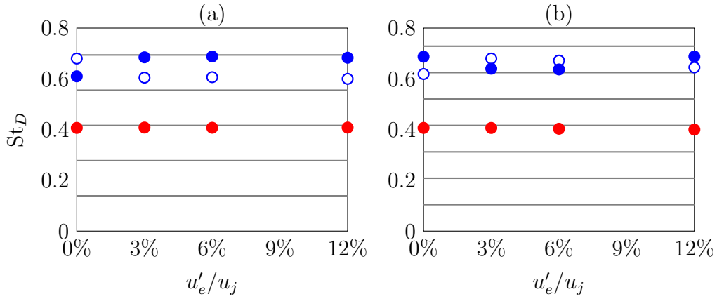
FIGURE 4.7 – Variations des nombres de Strouhal des pics \bullet dominants pour n_\theta = 0 et \circ dominants et \bullet secondaires pour n_\theta = 1 pour (a) L = 6r_0 et (b) L = 8r_0 avec le pic d'intensité des fluctuations de vitesse pour les jets libres équivalents; — nombres de Strouhal obtenus à partir du modèle (4.1).
