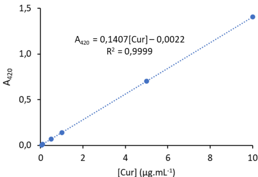
Figure III-1. Absorbance à \lambda = 420\ \text{nm} ( A_{420} ) en fonction de concentration de curcumine [\text{Cur}] dans eau/HCl 1M/EtOH 10/1/55 v/v ( n = 1 )
