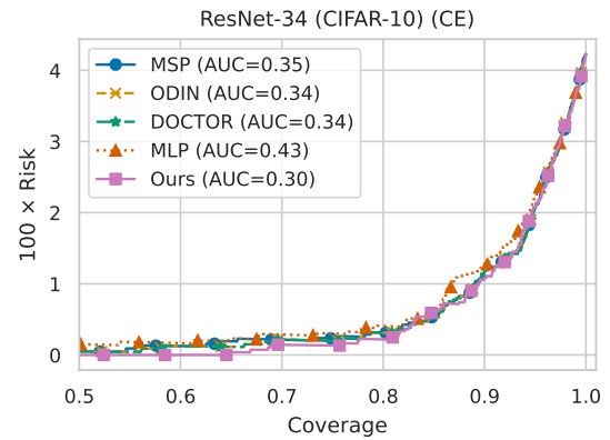
(d) ResNet-34 RC curve.
