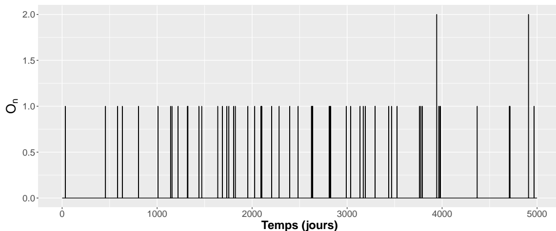
FIGURE 3.4 – Le cumul des nouveaux déclarés O_n correspondant au processus I pour une valeur de \Delta t = 1 jour.
