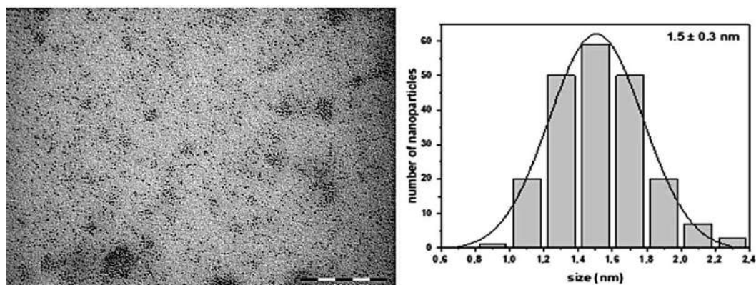
Figure 4: Image TEM des NPs de Ru 1 Ni 1 /PVP synthétisées à 85 °C (barre d'échelle 100 nm) et l'histogramme de taille respectif.
