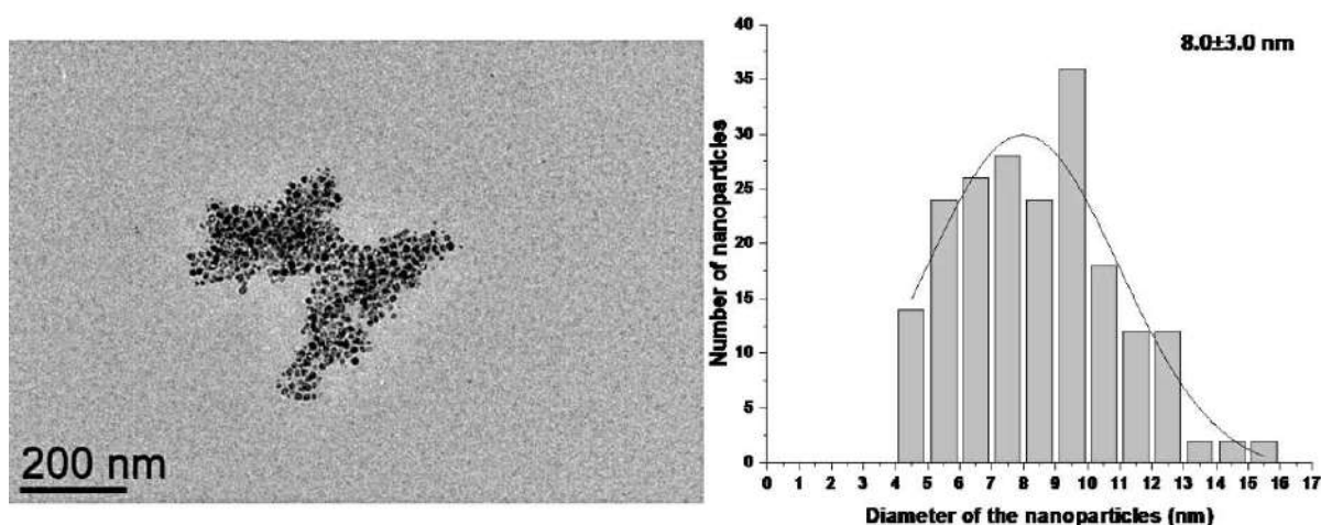
Figure 12: Image TEM de NPs de Cu/0.4 eq. HDA synthétisées à 100 °C (barre d'échelle 200 nm) et l'histogramme de taille respectif.
