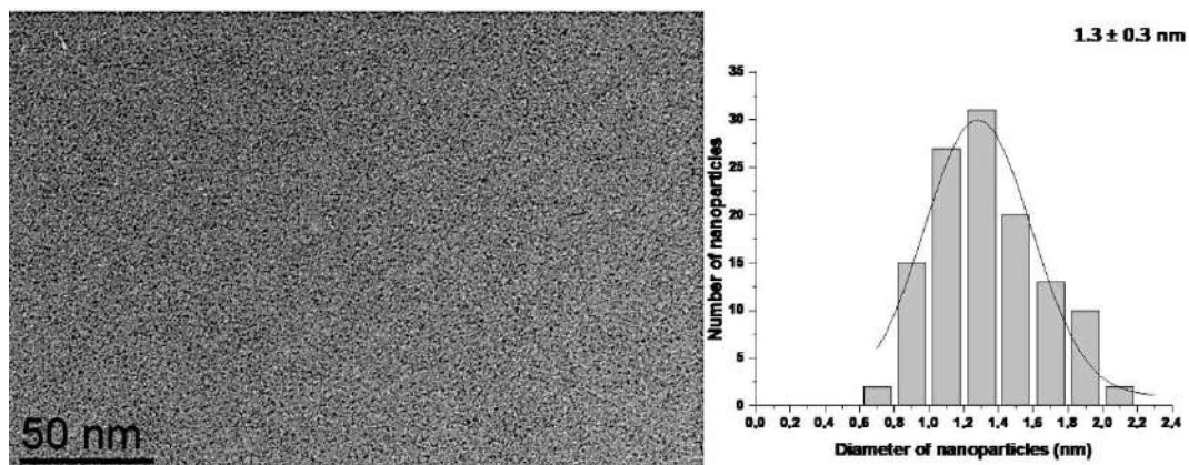
Figure 6: Image TEM de NPs de RuPNi/ \text{PPh}_2\text{Py} (barre d'échelle 50 nm) synthétisées à partir de [\text{Ru}(\eta^4\text{-C}_8\text{H}_{12})(\text{PPh}_2\text{Py})_2] et l'histogramme de taille correspondant.
