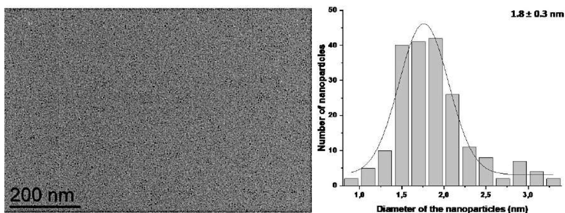
Figure 8: Image TEM de NPs de RuNi/AdCOOH (barre d'échelle 200 nm) et l'histogramme de taille respectif.
