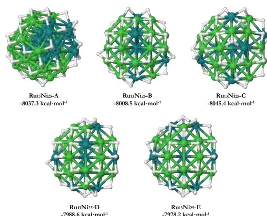
Figure 21: Modèles de Ru 13 Ni 25 avec un cœur de Ru (A à C) et avec une structure d'alliage (D et E) avec leurs énergies associées en kcal·mol -1 .
