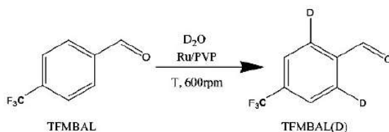
Schéma 13: Schéma réactionnel simplifié de la deutération catalytique de TFMBAL en TFMBAL(D).
