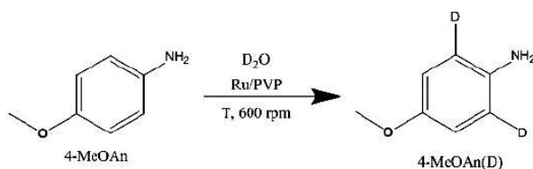
Schéma 12: Schéma réactionnel simplifié de la deutération catalytique de 4-MeOAn en 4-MeOAn(D).
