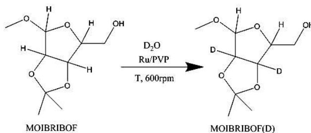
Schéma 14: Schéma réactionnel simplifié de la deutération catalytique du MOIBRIBOF en MOIBRIBOF(D).
