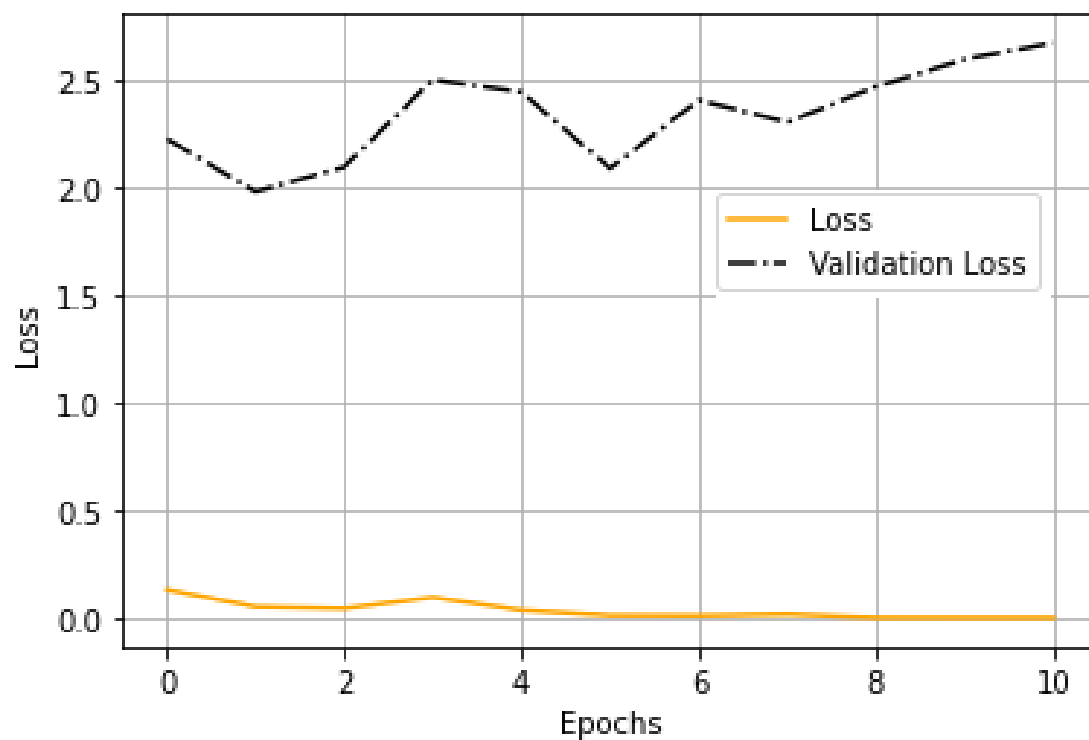
Figura 12: Característica de Calidad Verificable con BERT.
