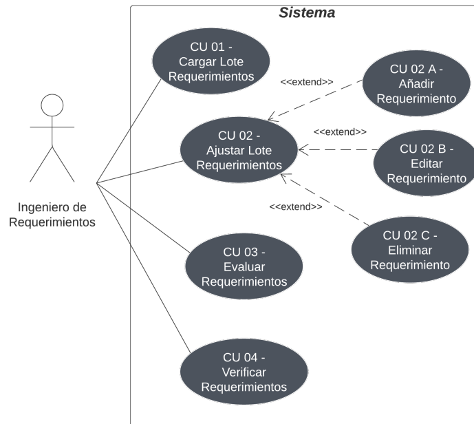
Figura 4.1: Diagrama de caso de uso.
