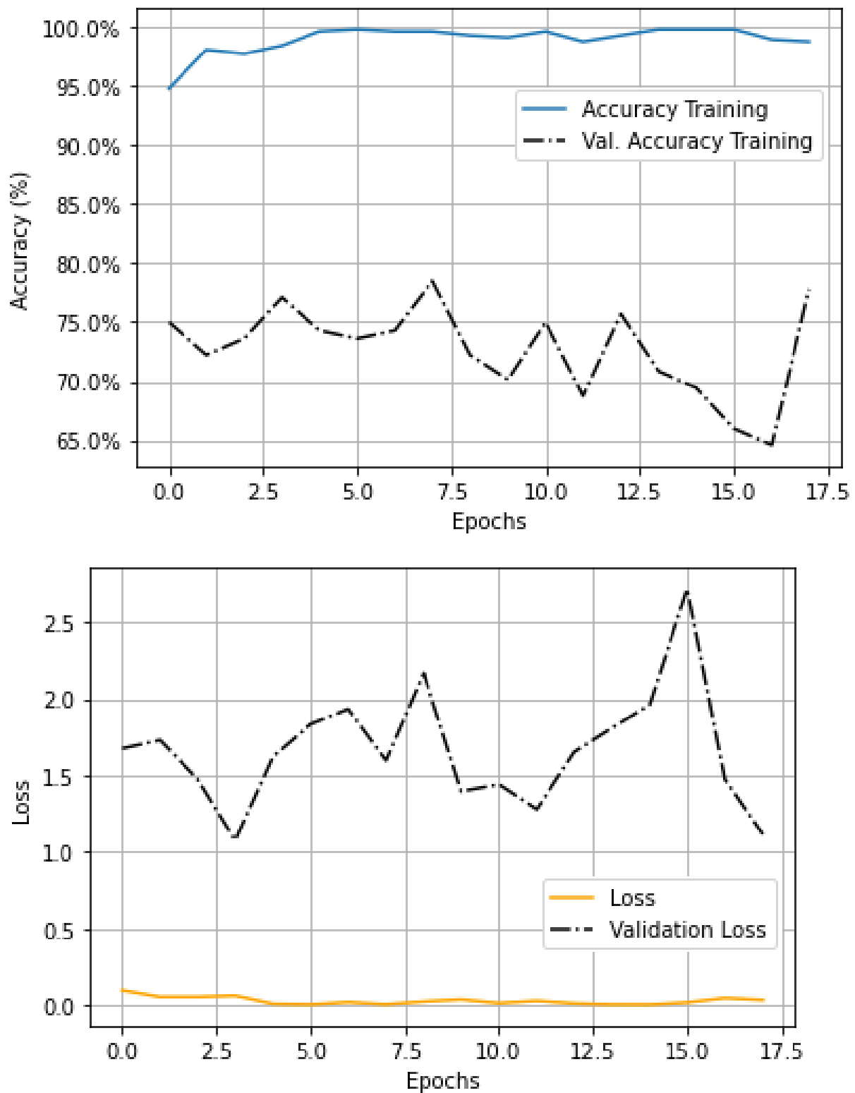
Figura 7: Característica de Calidad Ambiguo con BERT.
