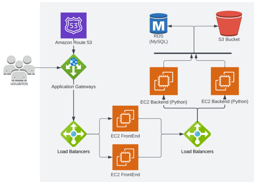
Figura 4.13: Diseño de infraestructura.
