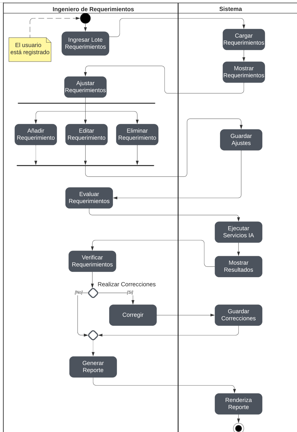
Figura 4.2: Diagrama de actividad.
