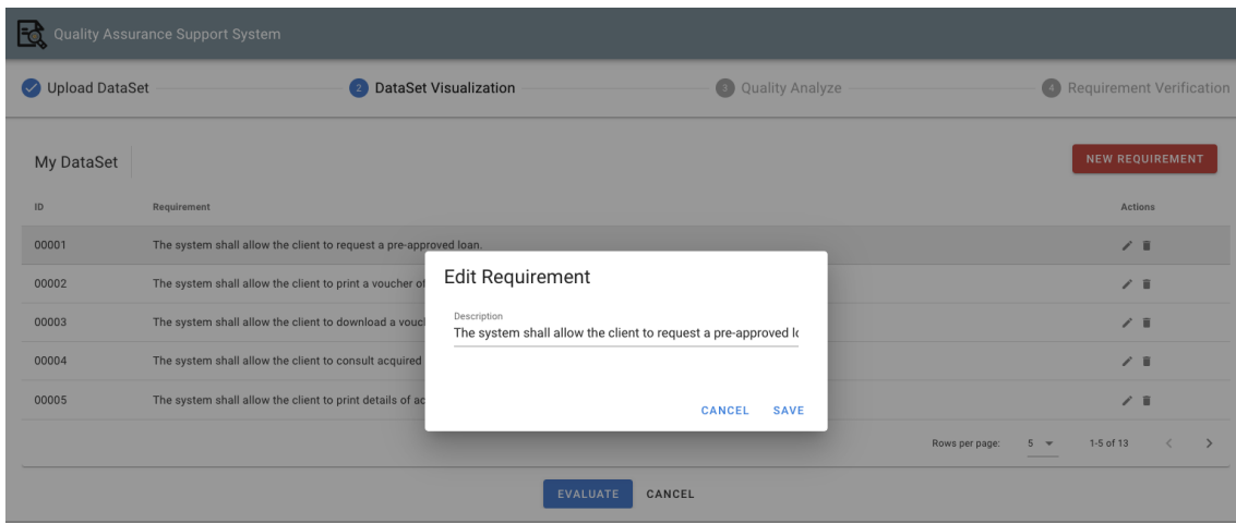
Figura 4.7: Interfaz Editar Requerimiento.
