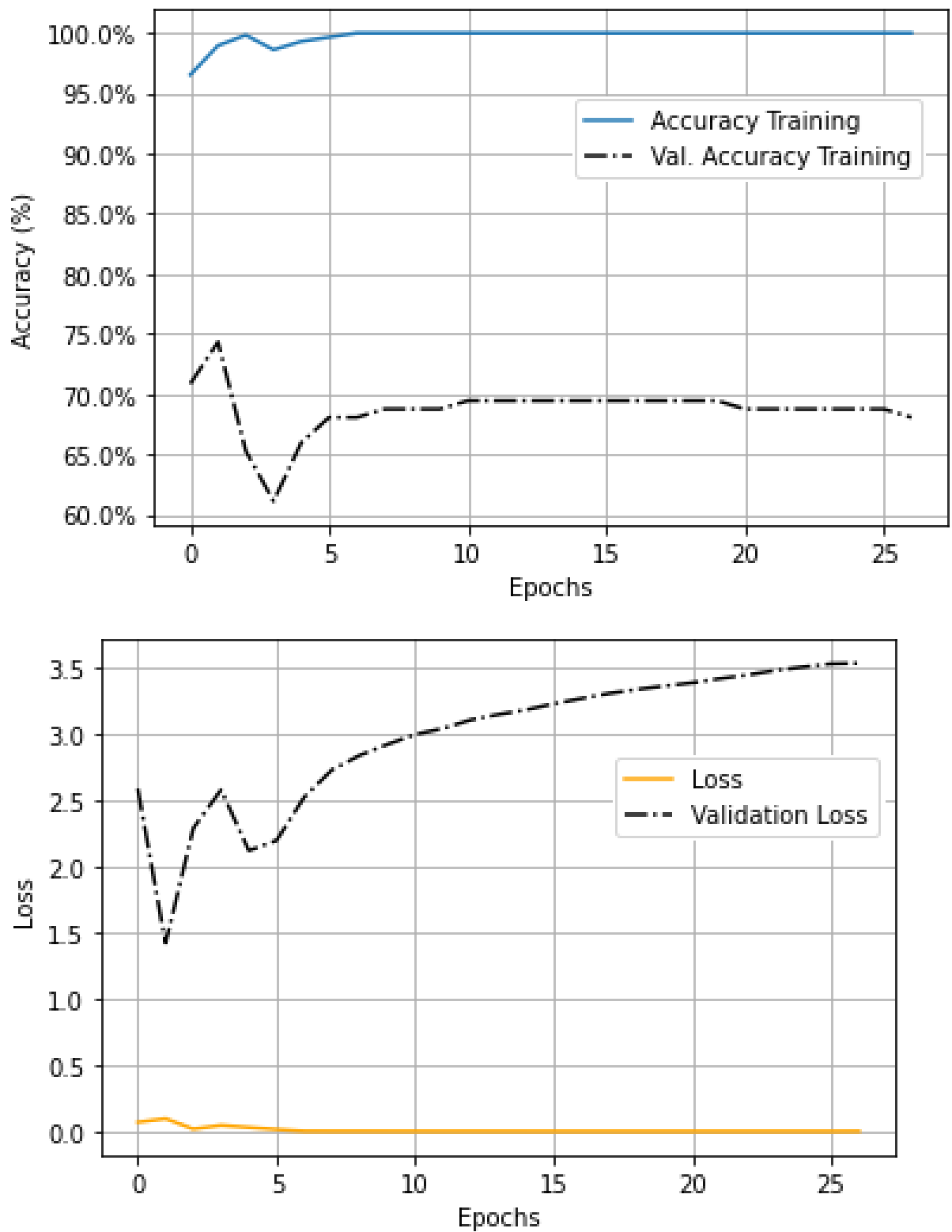
Figura 8: Característica de Calidad Conforme con BERT.
