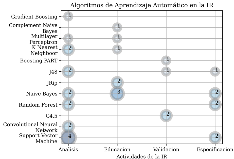
Figura 2.13: Algoritmos de aprendizaje automático aplicados en la IR.
