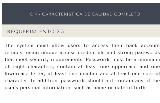
Figura 2.4: Característica de calidad Completo.
