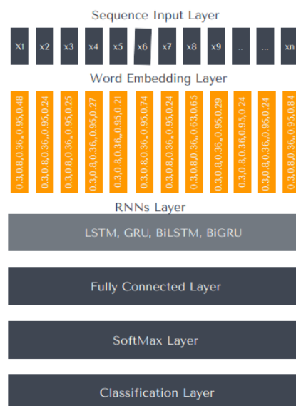
Figura 3.3: Arquitectura de red neuronal recurrente.
