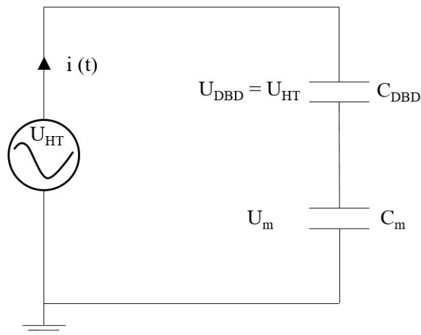
Figure II-10 : Schéma du circuit électrique équivalent du montage expérimental pour la mesure de la puissance par la méthode de Lissajous.
