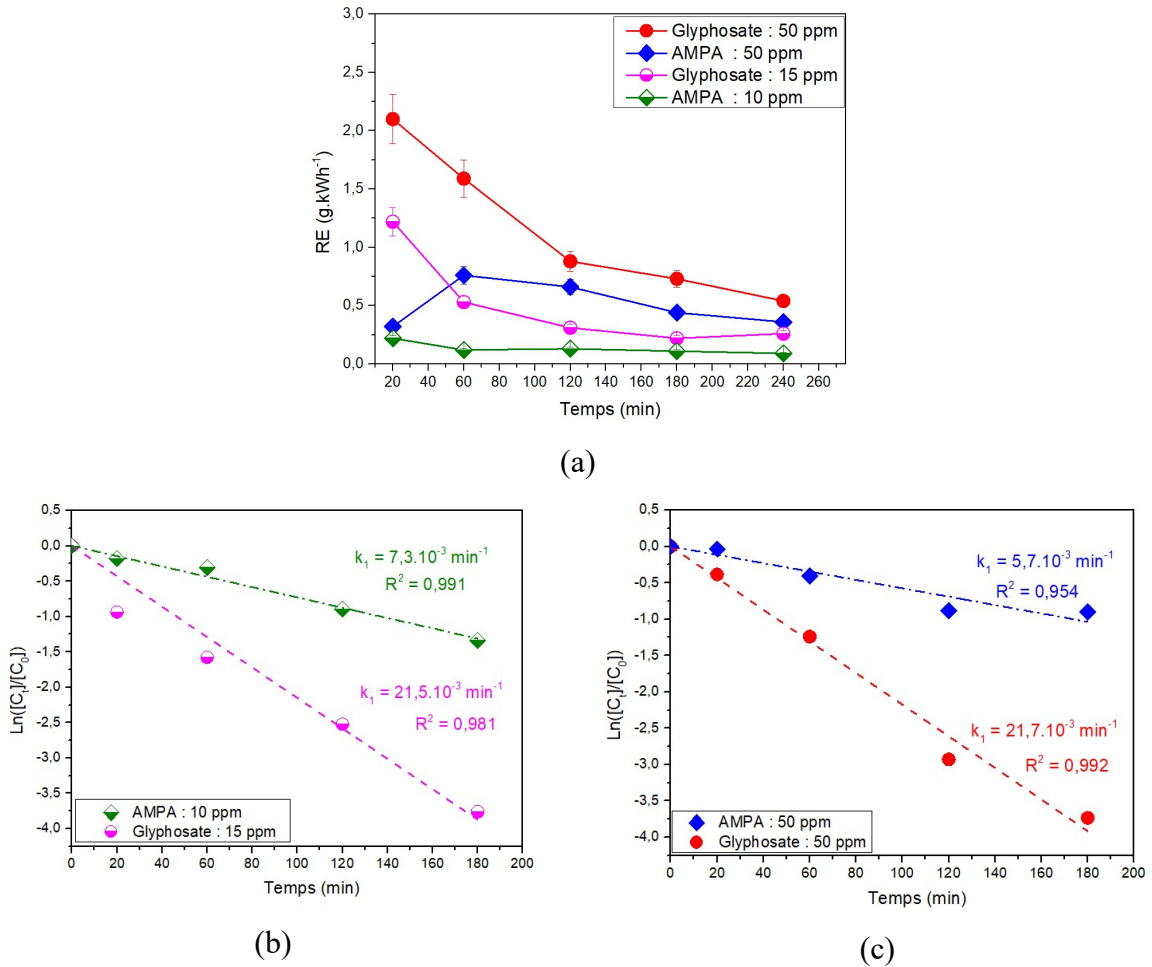
Figure IV-18: a) Rendement énergétique, a) modèle de pseudo-premier ordre pour les plus faibles concentrations initiales, et c) modèle de pseudo-premier ordre pour les concentrations de 50 ppm pour la dégradation de solutions de glyphosate seul et d'AMPA seul par PNT/L27-Fe ( [\text{glyphosate}]_0 = 50 et 15 ppm, [\text{AMPA}]_0 = 50 et 10 ppm, P = 1 W, V = 40 mL, m_{CA}/V = 0,75 mg.mL -1 , d_{\text{électrode-liquide}} = 5 mm, Q_{\text{air}} = 25 sccm).
