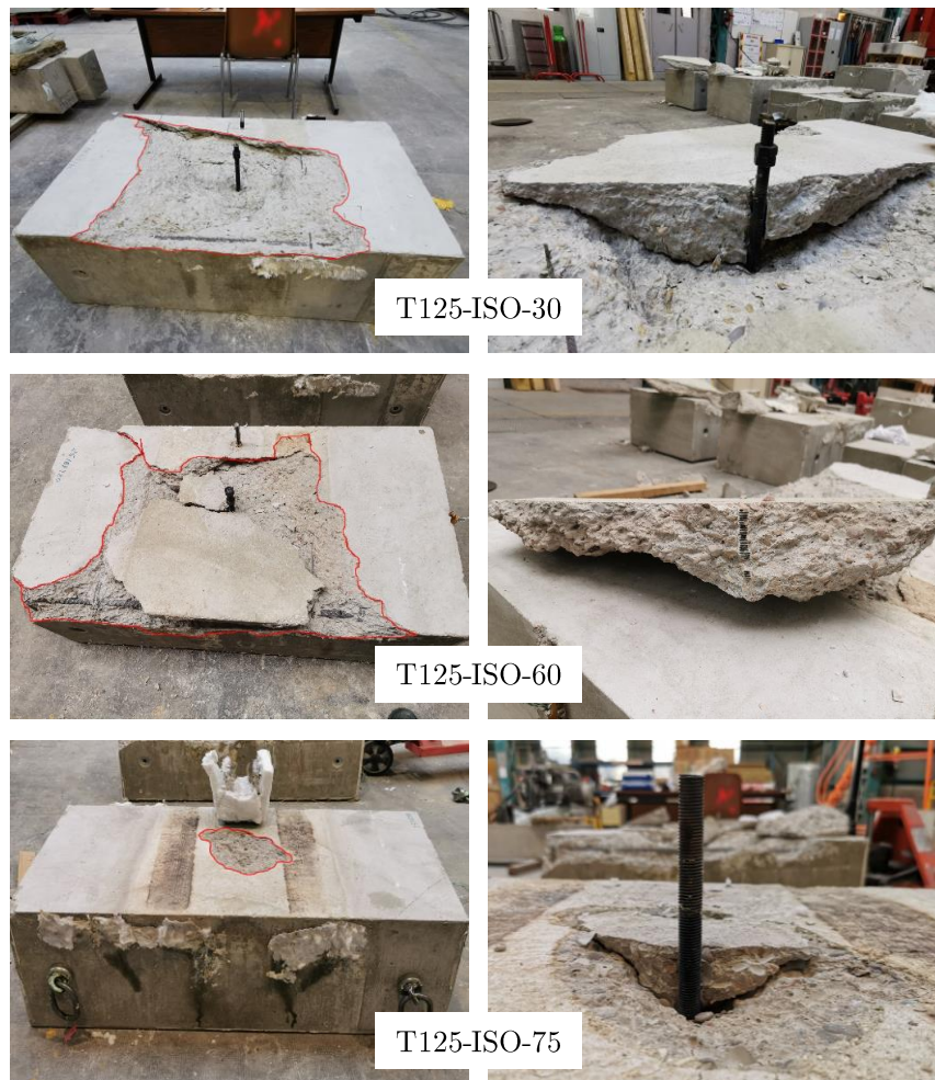
Figure 95 : Profils de rupture des chevilles chimiques sous conditions de feu standard
