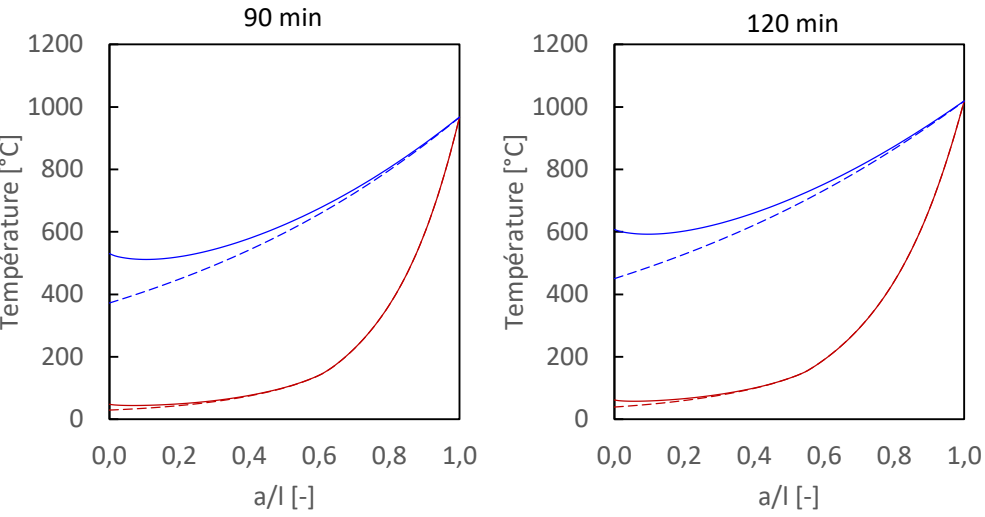
Figure 50 : Températures le long de la trajectoire de la fissure conique
