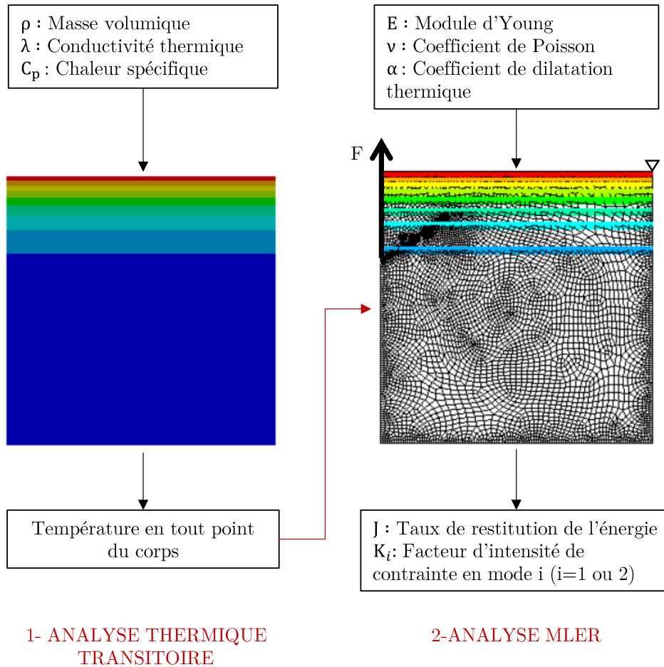
Figure 65 : Modèle thermomécanique en deux étapes
