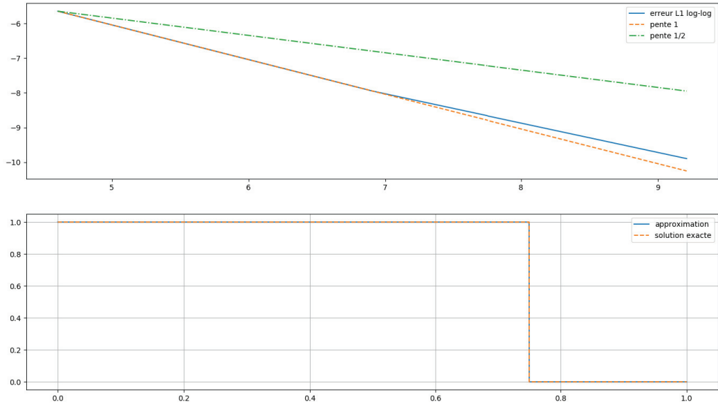
FIGURE 2.5 – Erreur numérique en échelle log-log pour le schéma de Rusanov pour l'équation de Burgers après compression de la donnée en un seul choc.
