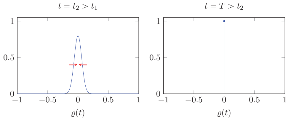
FIGURE 1.3 – Comportement de la solution de (3.11) pour W(x) = |x| en temps long, donnée initiale composée de deux gaussiennes (fusion puis concentration).
