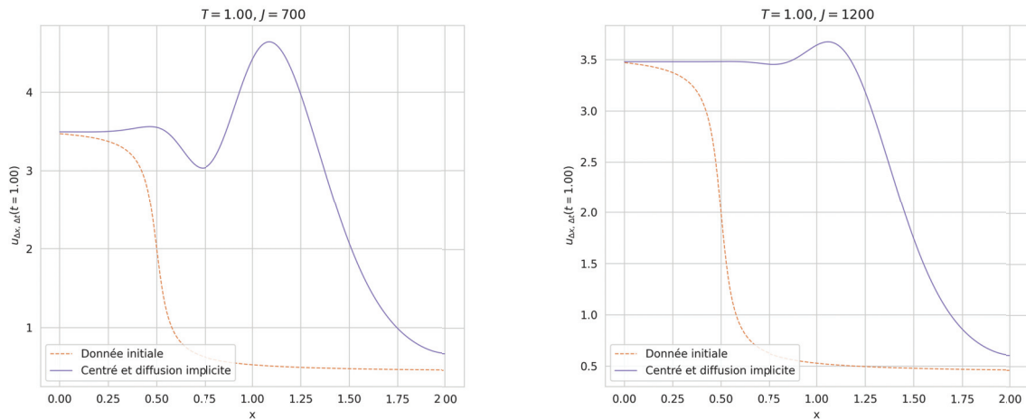
FIGURE 2.7 – Les mêmes paramètres qu’à la figure 2.6, mais avec 700 et 1200 mailles permettent de faire ressortir l’existence d’oscillations, qui ne sont toutefois pas aussi violentes que ce que l’on connaît en l’absence de diffusion, ainsi que le fait que l’amplitude de celles-ci tend vers 0 lorsque l’on raffine le maillage. Il est donc probable que le schéma converge \ell^\infty . On constate qu’il est en fait stable \ell^\infty au sens où \|u^n\|_{\ell^\infty} reste bornée. Le schéma downwind donne exactement le même type de graphe.
