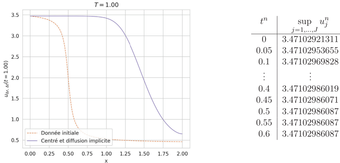
FIGURE 2.6 – Schéma centré avec diffusion implicite, pour le transport-diffusion linéaire à vitesse a = 1 et coefficient de diffusion \varepsilon = 0.05 , à T = 1 , J = 2000 mailles, avec a \frac{\Delta t}{\Delta x} = 50 et \frac{a^2 \Delta t}{2\varepsilon} = 0.5 . Le schéma global semble stable, même en norme \ell^\infty : il ne présente visiblement pas d'oscillations même en temps petit. Mais à y regarder de plus près, le principe du maximum n'est pas respecté : le schéma n'est pas stable \ell^\infty au sens usuel. On constate néanmoins, numériquement, qu'il est stable \ell_{\Delta x}^2 , ce que l'on retrouvera avec une analyse Von Neumann.
