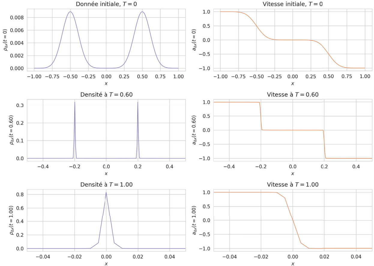
FIGURE 2.1 – Exemple de comportement du schéma upwind (2.1) pour donnée régulière, W(x) = |x| , 401 mailles, CFL= 0.9. On constate un peu de diffusion numérique qui fait « baver » la masse de Dirac sur 3 mailles.
