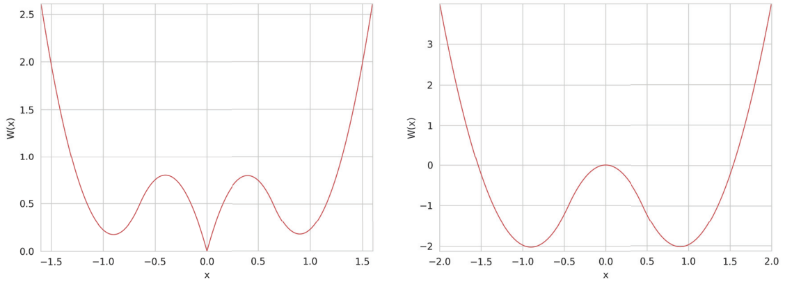
FIGURE 1.9 – Un potentiel admissible (gauche) et un potentiel non admissible (droite)
