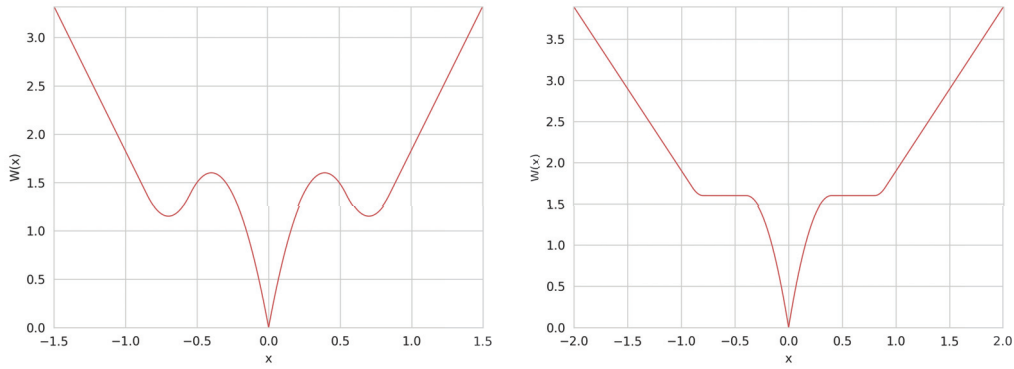
FIGURE 1.8 – Potentiels vérifiant W(x) \geq C|x| mais pas (A4-1)
