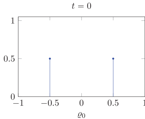
FIGURE 1.5 – Donnée initiale pour x_1 = -0.5 et x_2 = 0.5
