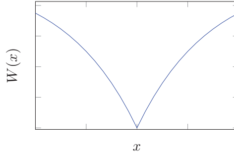
FIGURE 1.7 – Un potentiel pointu
