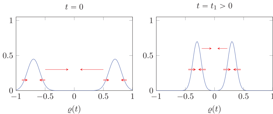
FIGURE 1.2 – Comportement de la solution de (3.11) pour W(x) = |x| , donnée initiale composée de deux gaussiennes, avant l'apparition de singularité ou la fusion des deux gaussiennes.
