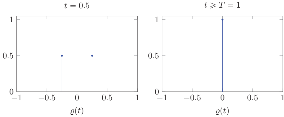
FIGURE 1.6 – Solution de (3.11) pour W(x) = |x| , donnée initiale deux masses de Dirac
