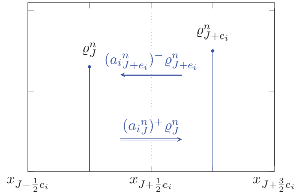
FIGURE 2.2 – Flux numérique F_{J+\frac{1}{2}e_i}^n (dans la direction i ) pour le schéma (2.1)
