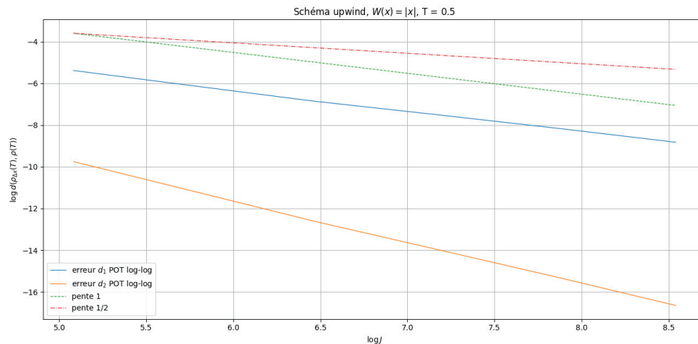
FIGURE 2.4 – Erreur numérique en échelle log-log pour le schéma (2.1), avec le potentiel W(x) = |x| en dimension d = 1 et pour donnée initiale \varrho^{ini} = \frac{1}{2}\delta_{-0.5} + \frac{1}{2}\delta_{0.5} . La distance W_1 (notée d_1 en légende) est calculée grâce à la représentation de la proposition 2.1, et la distance W_2 (notée d_2 ) est calculée avec le package Python POT. L'ordre de convergence observé est 1 au lieu de 1/2.
