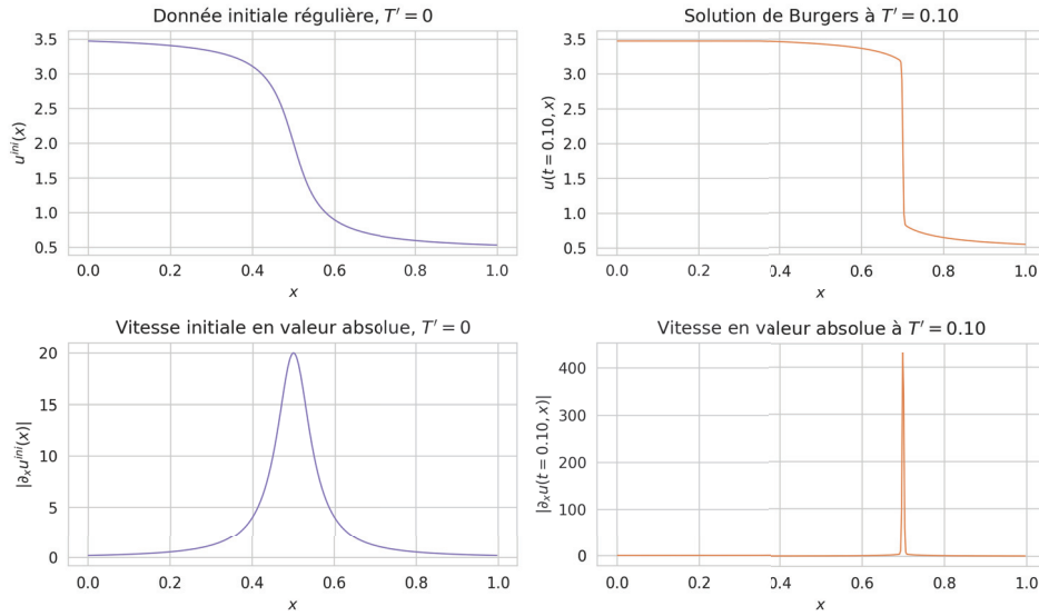
FIGURE 2.3 – Solution de l'équation de Burgers pour donnée décroissante, donc de temps de vie fini : |\partial_x u(T', x)| tend vers +\infty lorsque T' tend vers le temps d'apparition du choc.
