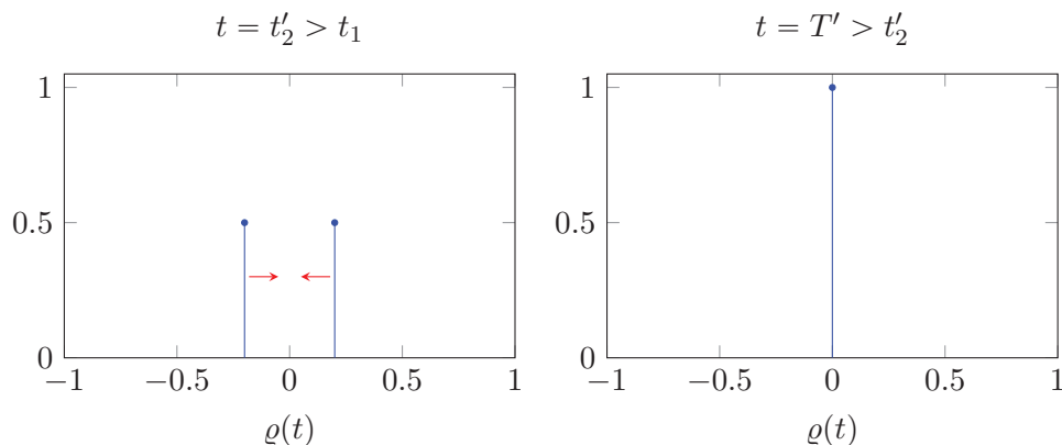
FIGURE 1.4 – Solution de (3.11) pour W(x) = 1 - e^{-|x|} en temps long, donnée initiale composée de deux gaussiennes (concentration puis fusion).
