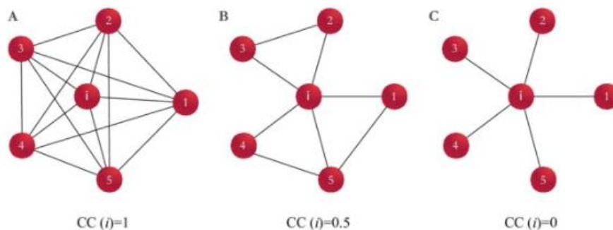
Figure 1. Exemples de coefficients de clustering d'un nœud dans trois graphes différents. Guiherme Ferraz de Aruda, Francisco A Rodrigues, Yamir Moreno, « Fundamentals of spreading processes in single and multilayer complex networks », Physics Reports , 756(4), 2018.
