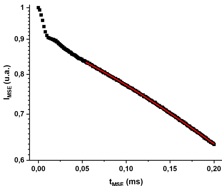
FIGURE V.26 – Signal de relaxation obtenu par MSE ^1H mesuré à T = 373 K du nanocomposite (80/20) à base de PEG3000. L'ajustement de la composante I_{mobile} est représenté en rouge.
