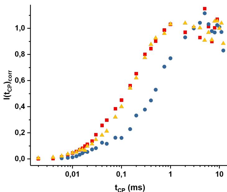
FIGURE V.59 – Montées de polarisation croisée ^1\text{H} \rightarrow ^{13}\text{C} des carbones des groupes CH et -CH 2 - des chaînes de RAN2500 (en rouge) et de RAN3900 (en jaune) au sein des nanocomposites (80/20), mesurées à T = 343\text{ K} et corrigées par les effets de relaxation en T_{1,\rho}(^1\text{H}) . Les résultats déterminés pour les carbones des groupes -CH 2 - du PEG3000 sont rappelés (en bleu) pour comparaison.
