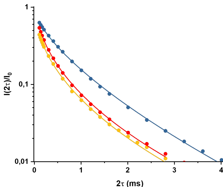
FIGURE V.49 – Signal de relaxation transverse ^1\text{H} déterminé par des expériences d'écho de Hahn effectuées pour les nanocomposites (80/20) à base de PEG3000 (en bleu), RAN2500 (en rouge) et RAN3900 (en jaune), à T = 343 \text{ K} .
