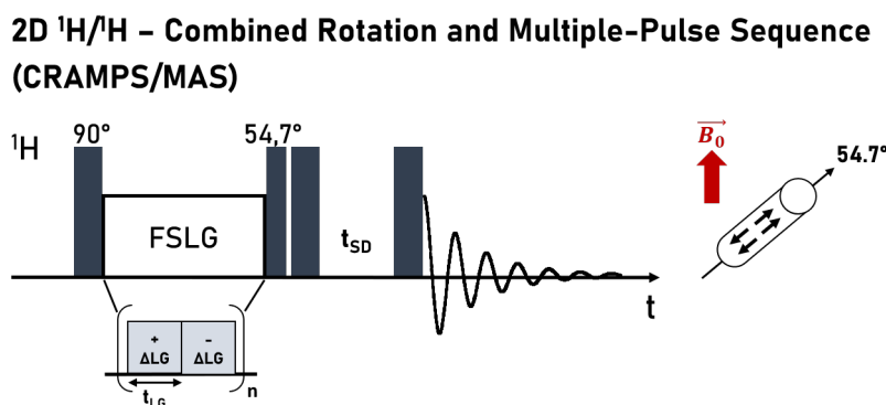
FIGURE II.17 – Séquence d'impulsions des expériences de corrélation 2D ^1\text{H} - ^1\text{H} de type FSLG/MAS.
