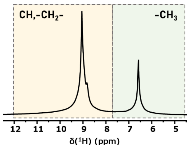
FIGURE IV.10 – Spectre mesuré à T = 343\text{ K} par la séquence T1irES ^1\text{H} , t_{evol} = 24\text{ s} , pour le nanocomposite (80/20) à base de RAN3900.
