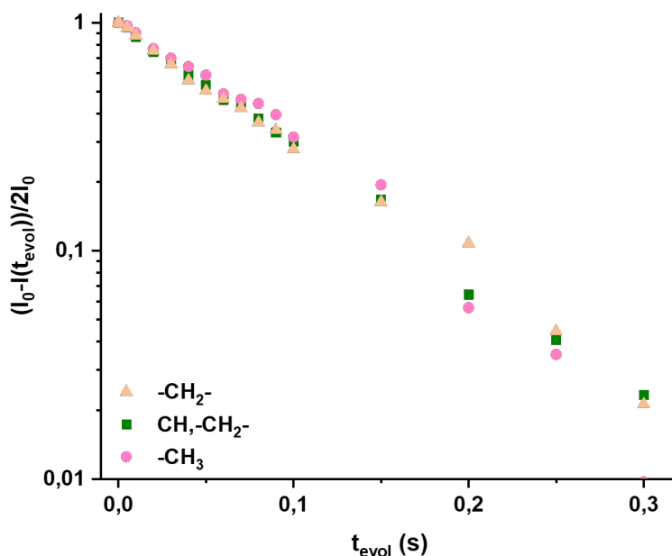
FIGURE IV.27 – RMN ^{13}C : évolution des pics correspondant aux groupements CH, -CH_2- et -CH_3 en fonction de t_{evol} du nanocomposite (80/20) à base de RAN3900 à \nu_r = 4 kHz et T = 343 K pour un temps de contact t_{CP} = 1 ms.
