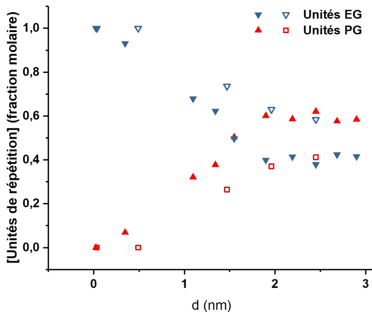
FIGURE VII.13 – Profil de la fraction molaire des unités de répétition en fonction de la distance obtenu pour le nanocomposite (80/20) à base de RAN3900 (carrés et triangles vides) pour comparaison avec celui obtenu pour le nanocomposite (80/20) à base de TB2900 (carrés et triangles pleins).
