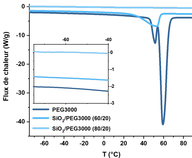
FIGURE V.6 – Thermogramme des NCs à base de PEG3000. Le balayage se fait de -80\text{ }^{\circ}\text{C} à 100\text{ }^{\circ}\text{C} à la vitesse de 10\text{ }^{\circ}\text{C}/\text{min} . Exo up.
