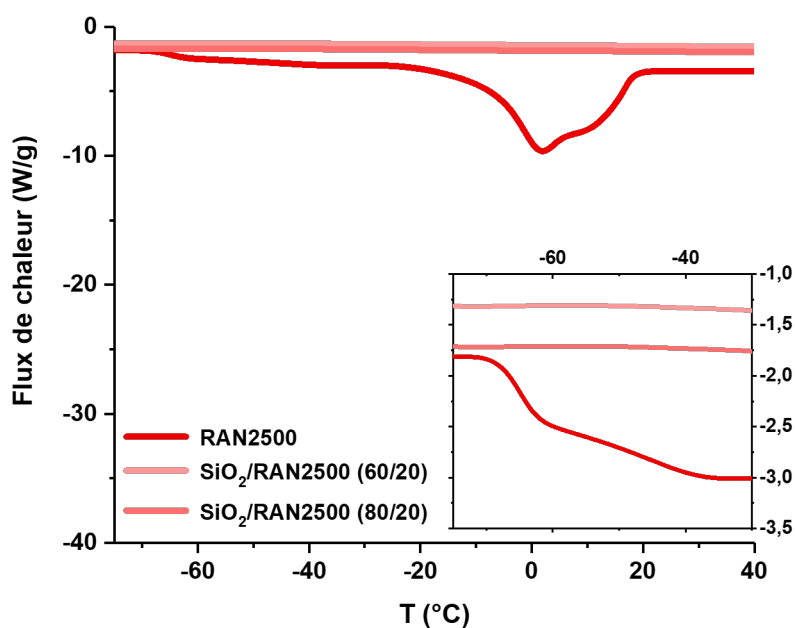
FIGURE V.7 – Thermogramme des NCs à base de RAN2500. Le balayage se fait de -80\text{ }^{\circ}\text{C} à 100\text{ }^{\circ}\text{C} à la vitesse de 10\text{ }^{\circ}\text{C}/\text{min} . Exo up.
