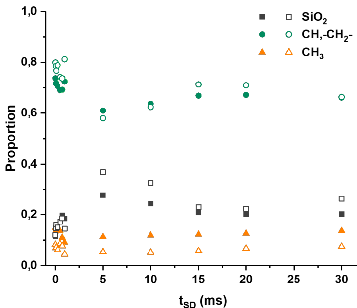
FIGURE VI.8 – Évolution de la proportion des groupements \text{CH} , \text{-CH}_2\text{-} et \text{CH}_3 en fonction de t_{SD} à \nu_r = 2\text{ kHz} et T = 343\text{ K} du nanocomposites (80/20) à base de RAN2500.
