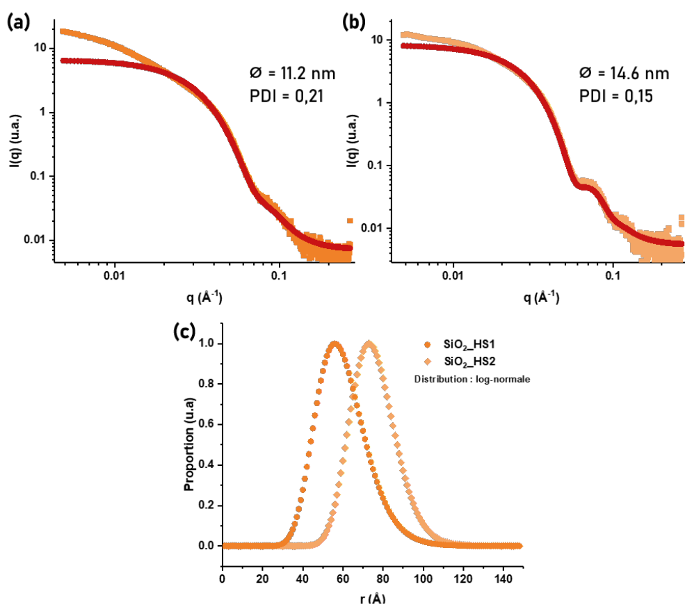
FIGURE III.5 – I(q) en fonction du vecteur de diffusion pour les lots HS1 (a) et HS2 (b) dilués à 1 wt%. Les ajustements des points expérimentaux (en rouge) ont été réalisés en choisissant le modèle d'une sphère et une polydispersité dont la distribution est de type log-normale. La distribution du rayon des nanoparticules de silice HS1 et HS2 est représentée en (c).
