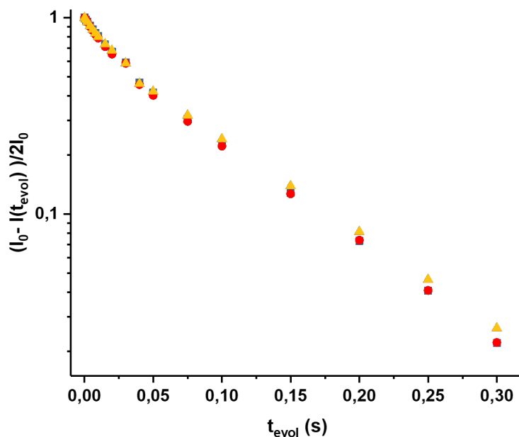
FIGURE IV.16 – Signaux de relaxation longitudinale T_1(^1\text{H}) des nanocomposite (80/20) à base de PEG3000 (bleue), RAN2500 (rouge) et RAN3900 (jaune), mesurés à T = 343 K.
