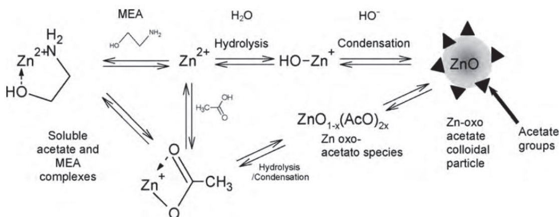
Figure II.4 : Schéma réactionnel d'hydrolyse et condensation dans le milieu Acétate de zinc / MEA / Alcool (Znaidi, 2003)
