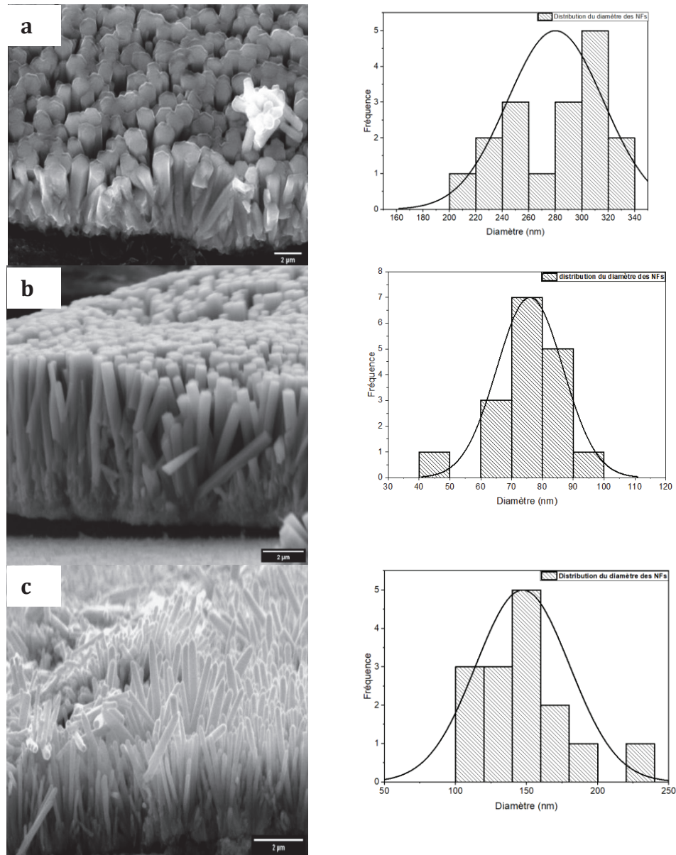
Figure IV.15 : Images MEB (vue en coupe) des nanofils de ZnO et distribution des diamètres à différentes température de dépôt (a) 70°C ; (b) 90°C et (c) 110°C - substrat S1, solution de précurseurs à 75mM et 50% de remplissage, une durée de croissance 5h
