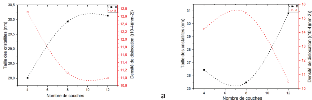
Figure III.14 : La taille cristalline et la densité de dislocation en fonction le nombre de couches de ZnO déposés avec l'isopropanol le long du pic de diffraction (100) pour une durée de recuit : (a) : t_1 et (b) : t_2 .
