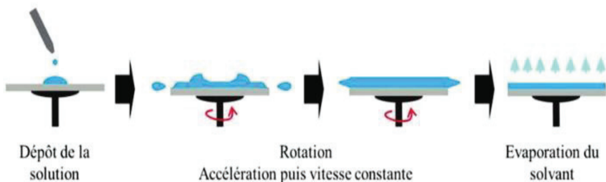
Figure II.3: Schéma de dépôt de couche mince par spin coating (Berthuy, 2015)
