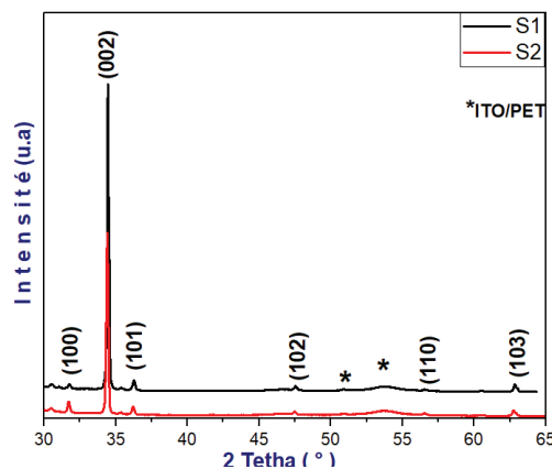
Figure IV.8 : Diffractogrammes de rayons X des nanofils de ZnO déposés sur deux différentes couches d'amorce (S1 : 2-méthoxyéthanol) et (S2 : isopropanol) pour une concentration de 75mM et un taux de remplissage de 50%
