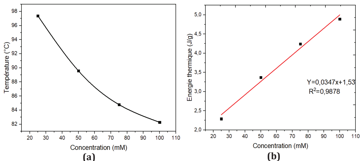
Figure IV.3 : (a) Variation de la température du sommet du second pic endothermique en fonction de la concentration de précurseurs (b) Variation de l'énergie du second pic endothermique en fonction de la concentration de précurseurs
