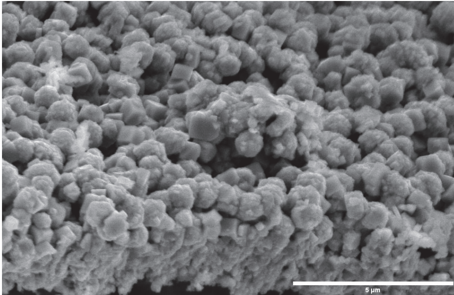
Figure V.10 : Images MEB en vue inclinée des hétérostructures de ZnO/PbS pour une concentration de Nitrate de Plomb 100mM ( C_{urée} = 0.3M )
