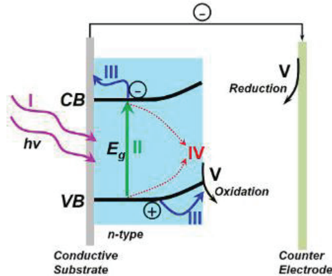
Figure I.10(b) : Principe d'une cellule photoélectrochimique (PEC) avec une photoélectrode de type n, (I) : Illumination ; (II) : Séparation de charge ; (III) : Migration de charge ; (IV) : Recombinaison de charge (V) : Réaction redox. CB= bande de conduction, VB = bande de valence, E_g = bande interdite (Li, 2015)
