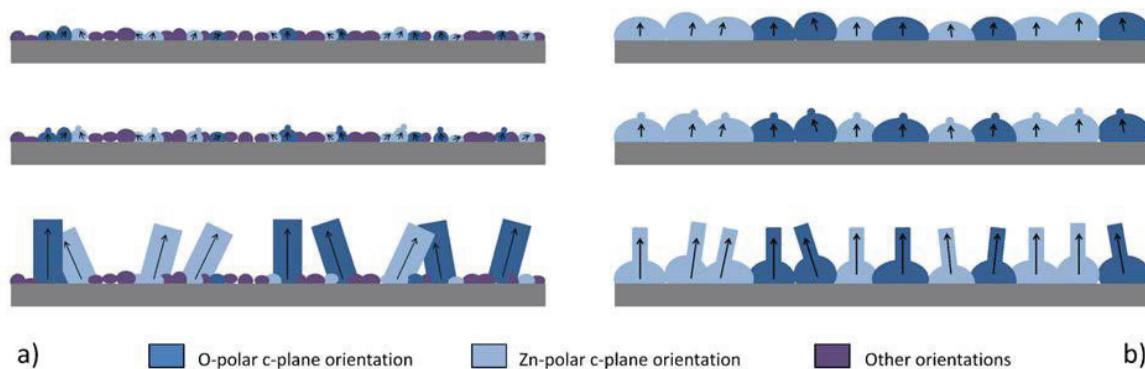
Figure III.1 : Diagramme schématisique des mécanismes de nucléation et de croissance de NFs d'oxyde de zinc élaborés par bain chimique sur couche d'amorce (a) fine, faiblement texturée (b) épaisse, fortement texturée (Guillemin, 2013)
