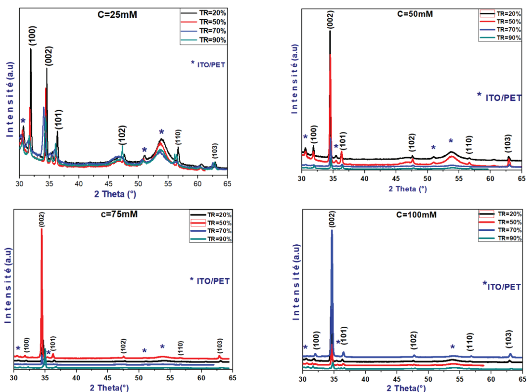
Figure IV.13 : Diffractogrammes de rayons X des nanofils de ZnO en fonction des taux de remplissage de l'autoclave (20%, 50%, 70% et 90%) pour différentes concentrations de précurseurs (25m, 50mM, 75mM et 100mM) - Couche tampon S1
