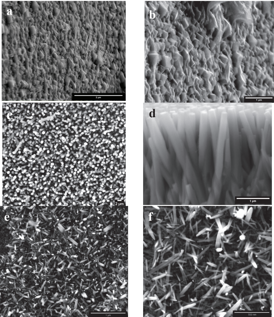
Figure IV.7 : Images MEB de nanostructures de ZnO déposées par voie hydrothermale à partir d'une solution de précurseur à 75mM et taux de remplissage 50% ; (a) et (b) sur le substrat ITO/PET sans la couche tampon ; (c) en vue de dessus et (d) en vue transversale sur la couche tampon S1 ZnO/ITO/PET ; (e) et (f) sur la couche tampon S2 ZnO/ITO/PET.
