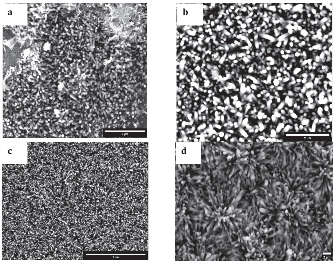
Figure IV.9 : Images MEB (vue de dessus) des nanofils de ZnO en fonction de différentes concentrations de précurseurs (a): 25mM (b): 50mM, (c) :75mM et (d) :100mM avec un taux de remplissage de 50% - couche tampon S1
