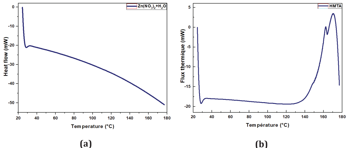
Figure IV.1 : Thermogramme (a) d'une solution aqueuse de Zn(NO_3)_2 \cdot 6H_2O à 75mM (b) d'une solution aqueuse de HMTA à 75mM.
