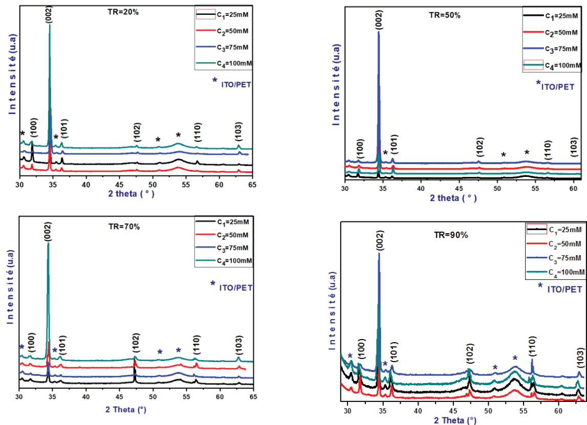
Figure IV.10 : Diffractogrammes de rayons X des nanofils de ZnO en fonction des concentrations de précurseurs (25m, 50mM, 75mM et 100mM) pour différents taux de remplissage 20%, 50%, 70% et 90% - Couche tampon S1
