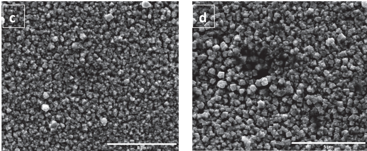
Figure V.8 : Images MEB des hétéro-structures de ZnO/PbS (a) 10mM, (b) 25mM, (c) 50mM et (d) 75mM avec C_{urée} = 0.3M déposés sur ZnO/ITO/PET à faible grossissement.
