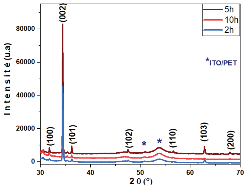
Figure IV.18 : Diffractogrammes de rayons X des réseaux de nanofils de ZnO obtenus en faisant varier le temps de croissance 2h, 5h et 10h - substrat S1, solution de précurseurs à 75mM et 50% de remplissage, température de croissance 90°C
