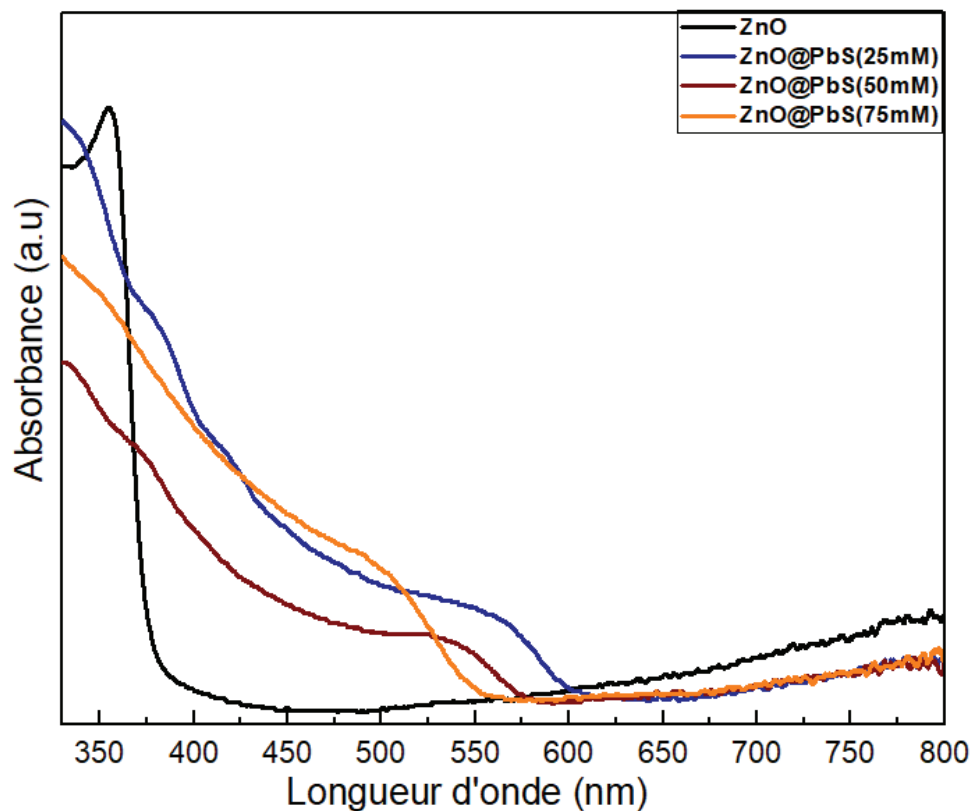
Figure V.15 : Spectres d'absorption de NFs de ZnO et de l'hétérojonction ZnO@PbS avec différentes concentrations de nitrate de plomb (25mM, 50mM et 75mM) et une concentration d'urée de 0.4M
