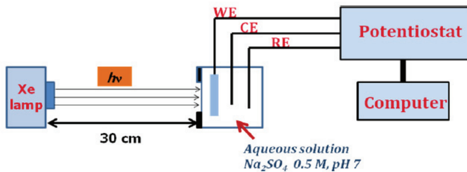
Figure II.15 : Montage photo-électrochimique disponible au laboratoire
