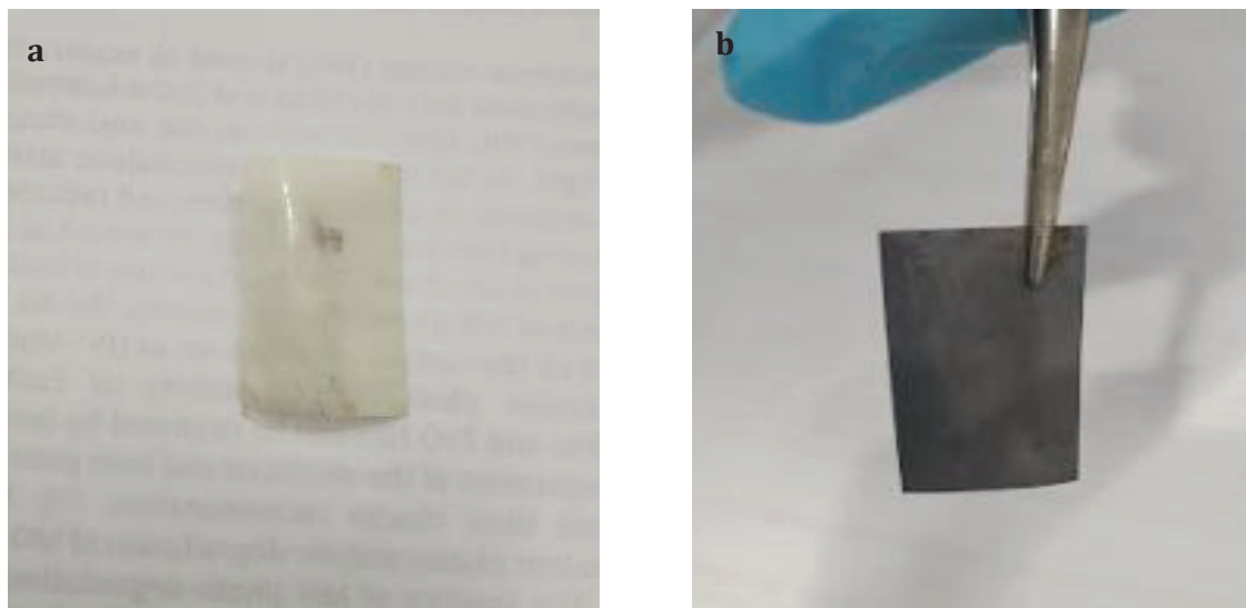
Figure V.1 : Aspect de l'échantillon (a) : des NFs de ZnO (b) : après le dépôt du NPs de PbS par voie hydrothermale
