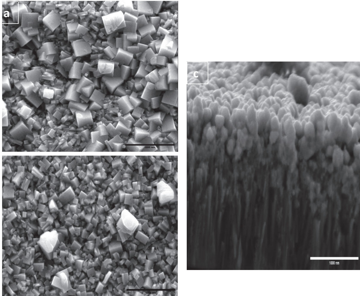
Figure V.6 : Images MEB des hétérojonctions avec (a) 0 M urée, (b) 0.3 M, (c) 0.4 M et une C(Pb(NO_3)_2) de 25mM
