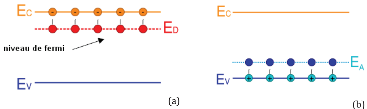
Figure I.5 : Représentation des niveaux d'énergie du (a) Semi-conducteur extrinsèque de type n et (b) Semi-conducteur extrinsèque de type p ( E_D niveau donneur ; E_A niveau accepteur)
