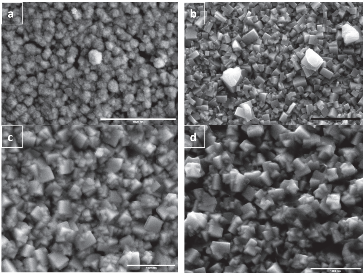
Figure V.9 : Images MEB des hétéro-structures de ZnO/PbS (a) 10mM, (b) 25mM, (c) 50mM et (d) 75mM avec C_{urée} = 0.3M déposés sur ZnO/ITO/PET à fort grossissement.
