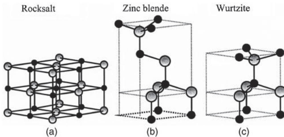
Figure I.16. : Représentation des structures cristallines du ZnO : (a) rocksalt cubique, (b) zinc blende cubique, (c) Wurtzite hexagonale. Atomes de zinc en gris et oxygène en noir (Özgür, 2005)
