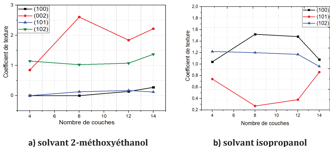
Figure III.10 : Evolution du coefficient de texture des couches d'amorce de ZnO en fonction du nombre de couches déposées avec (a) : le 2-méthoxyethanol (b) l'isopropanol
