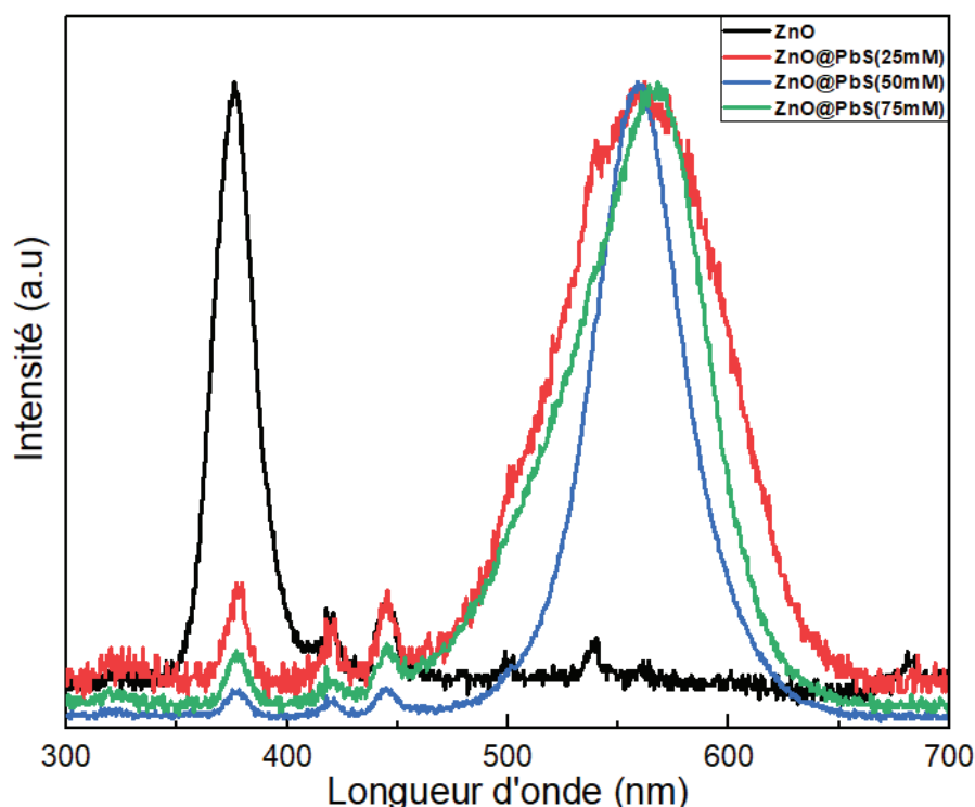
Figure V.17 : Spectres de photoluminescence de ZnO et de ZnO@PbS avec différentes concentrations de Nitrate de Plomb (25mM ; 50mM et 75mM) et une concentration d'urée de 0.4M
