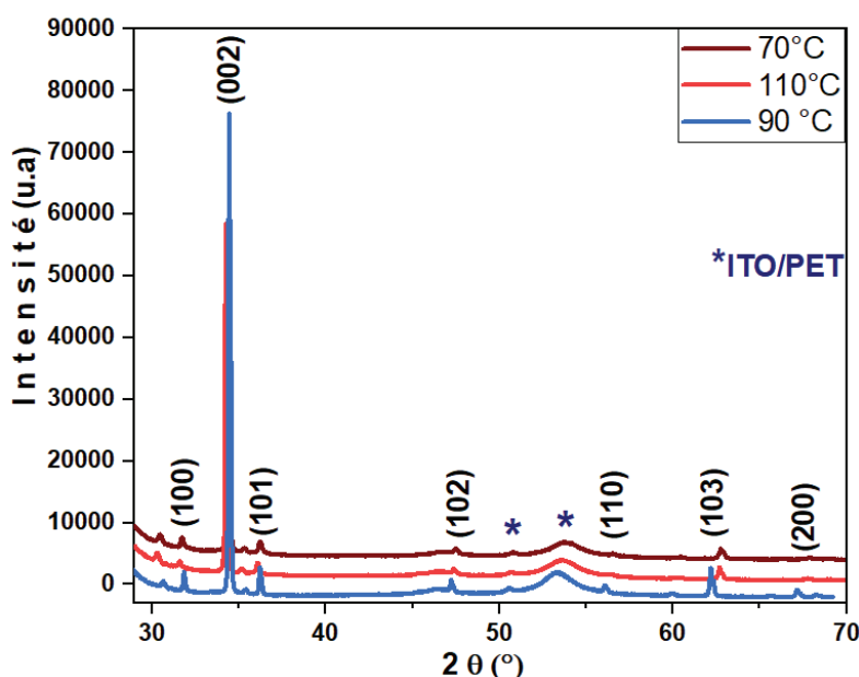
Figure IV.16: Diffractogrammes de rayons X des réseaux de nanofils de ZnO obtenus en faisant varier la température de croissance : 70, 90 et 110°C - substrat S1, solution de précurseurs à 75mM et 50% de remplissage, une durée de croissance 5h
