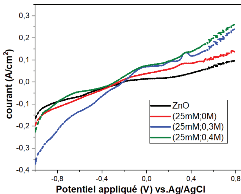
Figure V.19.b : Voltammogrammes à balayage linéaire des nanofils de ZnO (désignés par NFs ZnO) et des hétérostructures ZnO/PbS sous illumination dans une solution aqueuse de \text{Na}_2\text{SO}_4 et avec une vitesse de balayage de 10 \text{ mV s}^{-1} .
