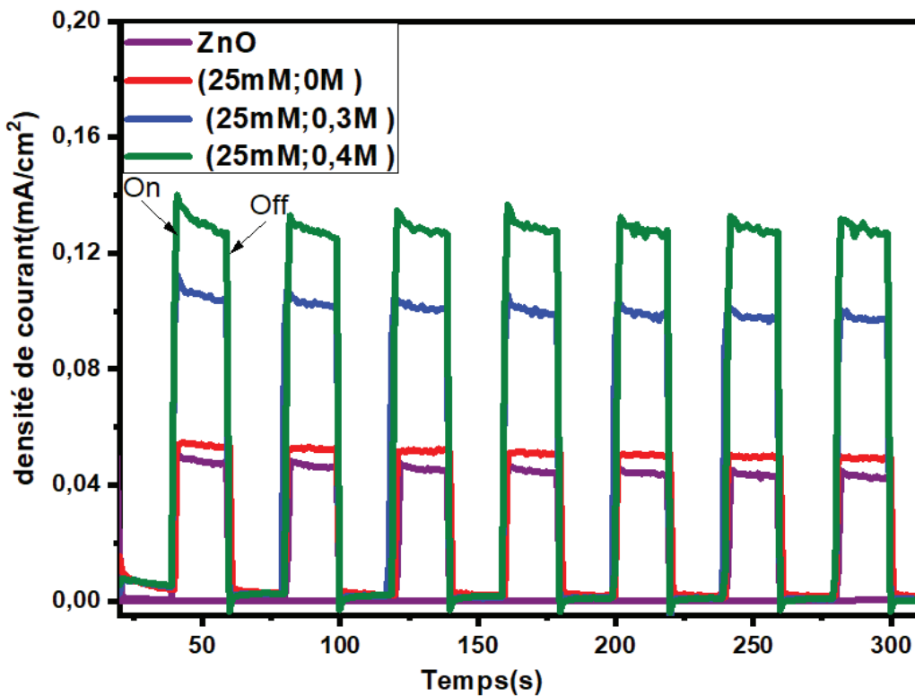
Figure V.19: Les réponses photocourant dans la solution aqueuse de Na_2SO_4 (0,5 M, pH = 7) des échantillons étudiés (les nanofils de ZnO et les hétérostructures (ZnO/PbS) à différentes concentrations d'urée) à une tension appliquée de 0.5V pendant 20 secondes de cycles illumination/obscurité.
