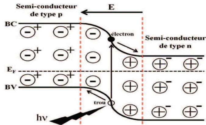
Figure I.8 : Schéma simple des phénomènes photovoltaïques dans les matériaux semi-conducteurs à jonction p-n (Fonash, 2010)
