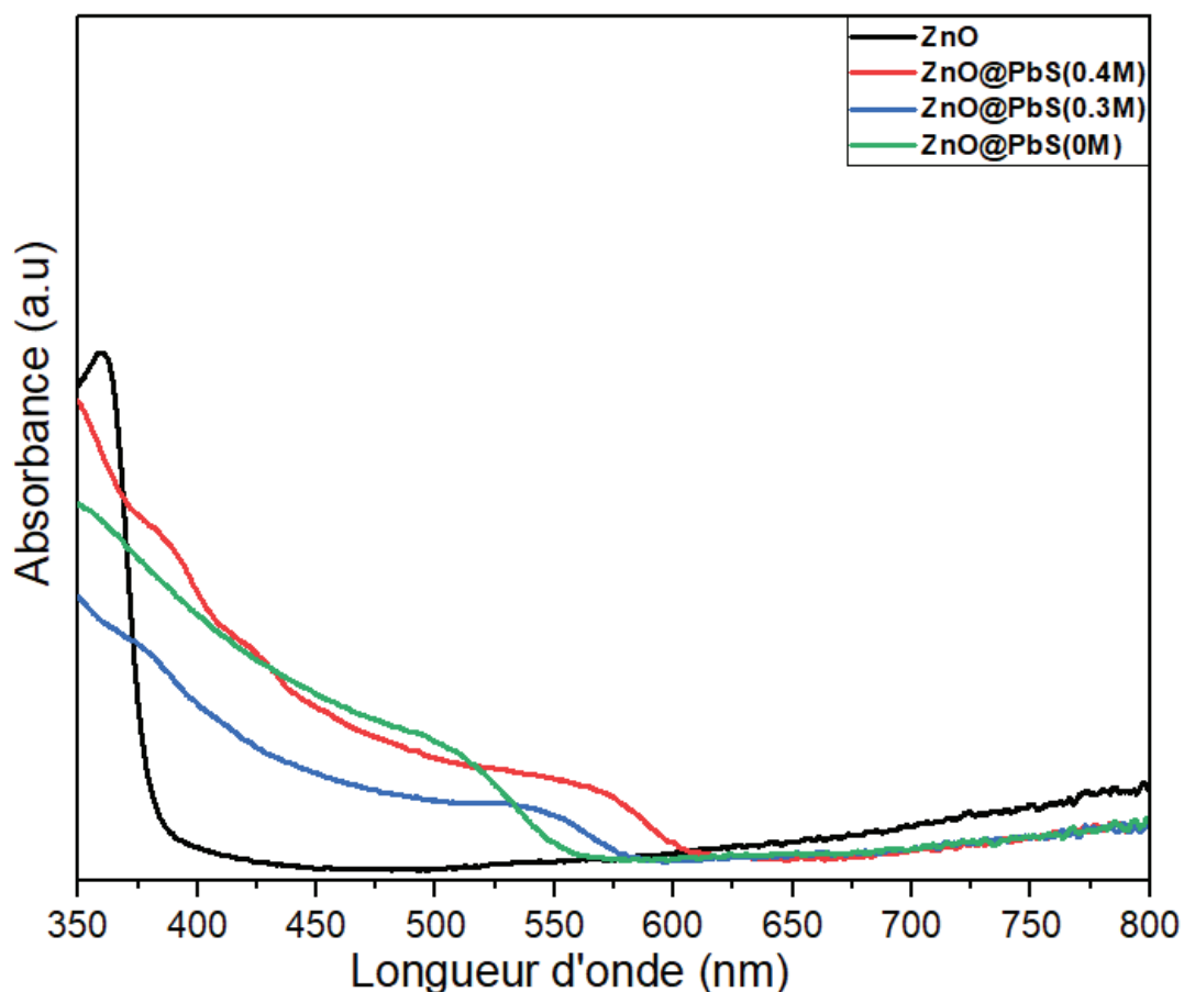
Figure V.14 : Spectres d'absorption de NFs de ZnO et de l'hétérojonction ZnO@PbS avec différentes concentrations d'urée (0M, 0.3M, 0.4M)
