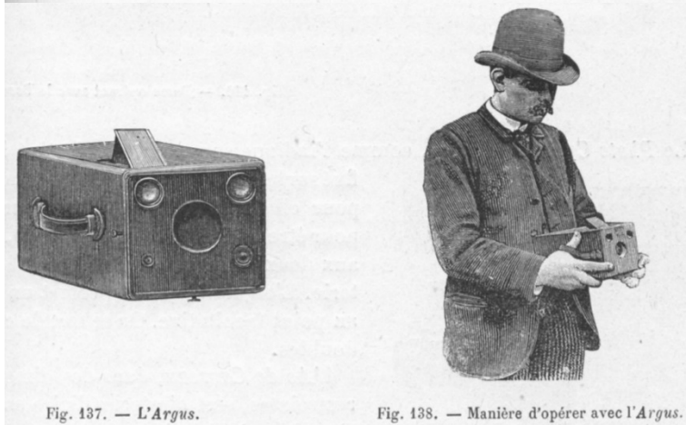
Appareil de type détective, Georges Brunel, La Photographie pour tous , Paris, 1894, p. 303
