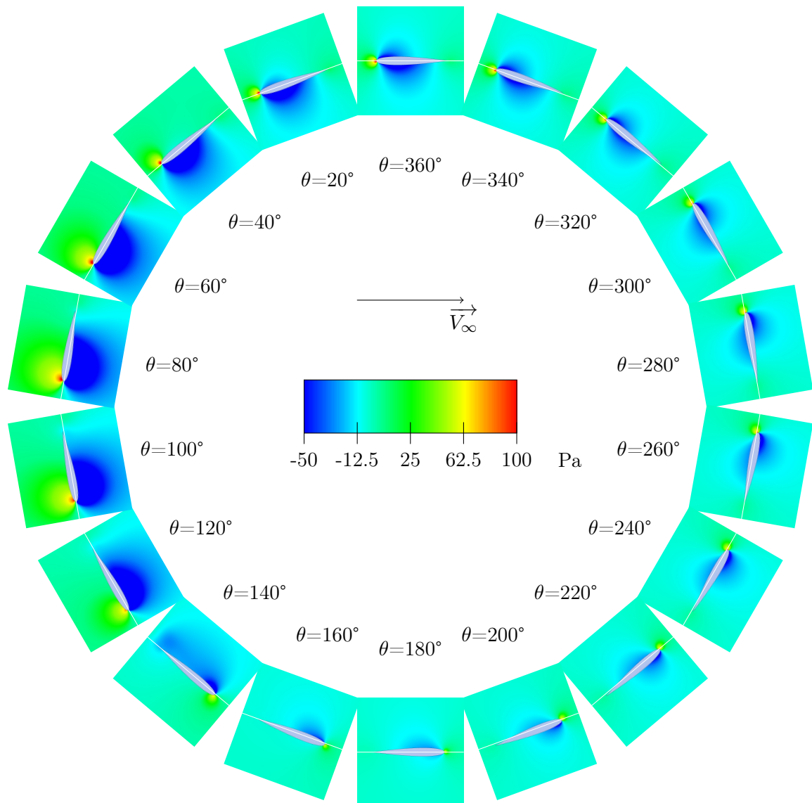
FIGURE 5.53 – champs de pression autour du foil dans le cas f3amoins1
