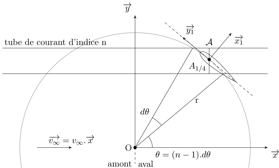
FIGURE 4.2 – Représentation schématique d'un tube
