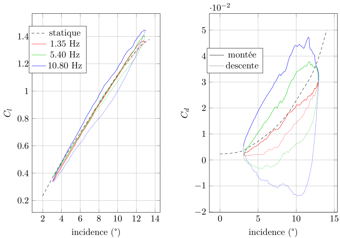
FIGURE 3.6 – Effets dynamiques sur les coefficients aérodynamiques en régime de décrochage léger
