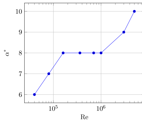
FIGURE 4.19 – Variation de l'angle de finesse maximale en fonction du nombre Reynolds selon les tables d'interpolation utilisées
