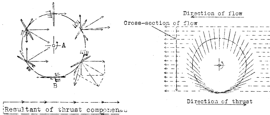
FIGURE 1.17 – Illustrations du système Kirsten-Boeing extraites de [Sachse 1926]
