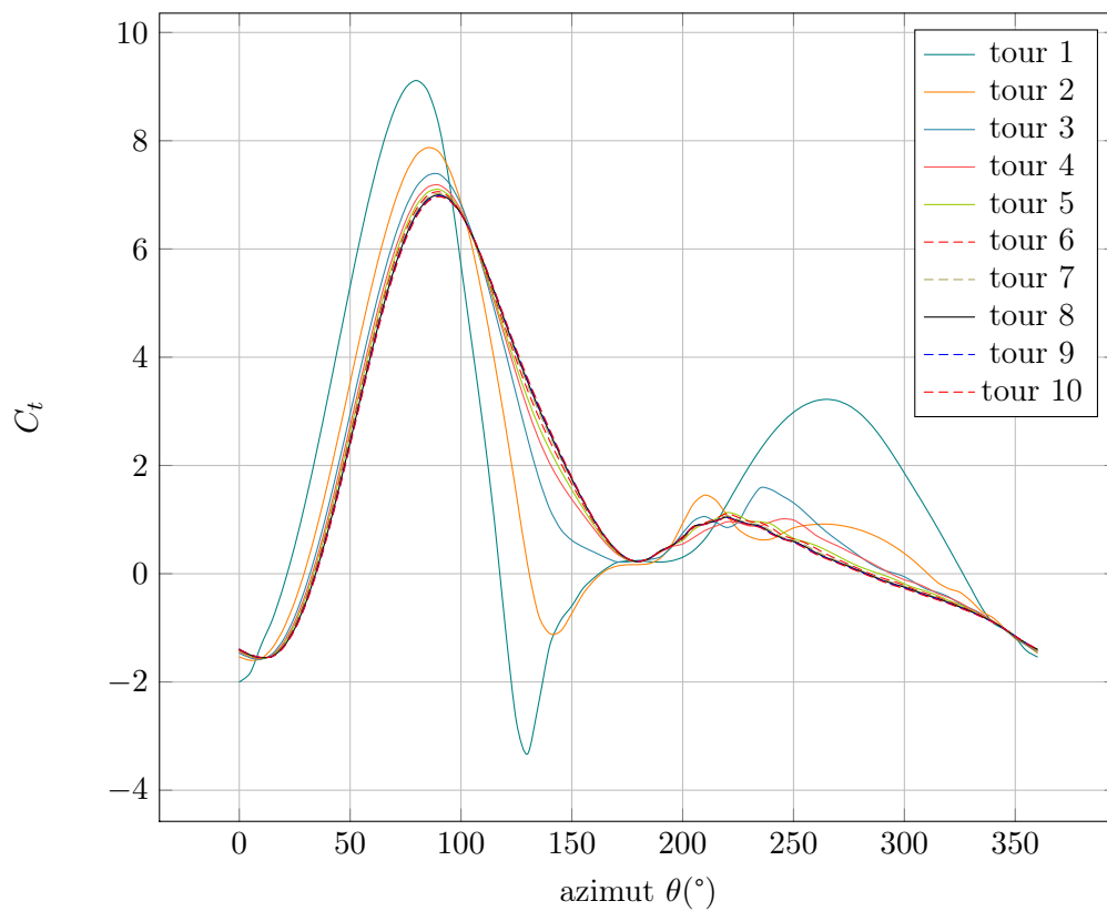
FIGURE 5.7 – Etude de convergence de sillage dans le cas D, \lambda = 5 table 2.2
