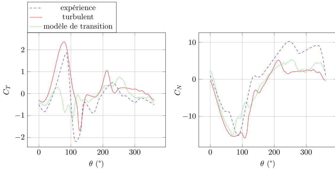
FIGURE 5.12 – Etude de modèle fluide : comparaison turbulent/transition, cas A, 10ème tour
