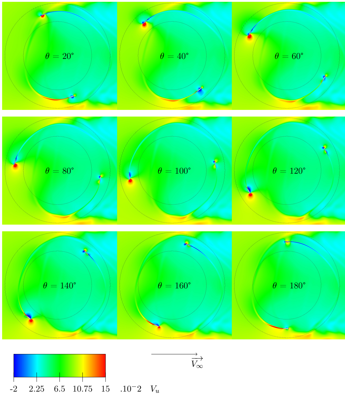
FIGURE 5.56 – Vitesse du fluide selon l'axe x pour le cas f3a3, \lambda = 5
