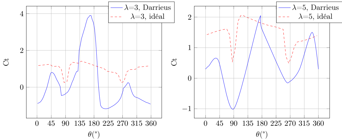
FIGURE 4.21 – efforts tangentiels comparés entre loi de pas idéal et Darrieus d’après le modèle DMST
