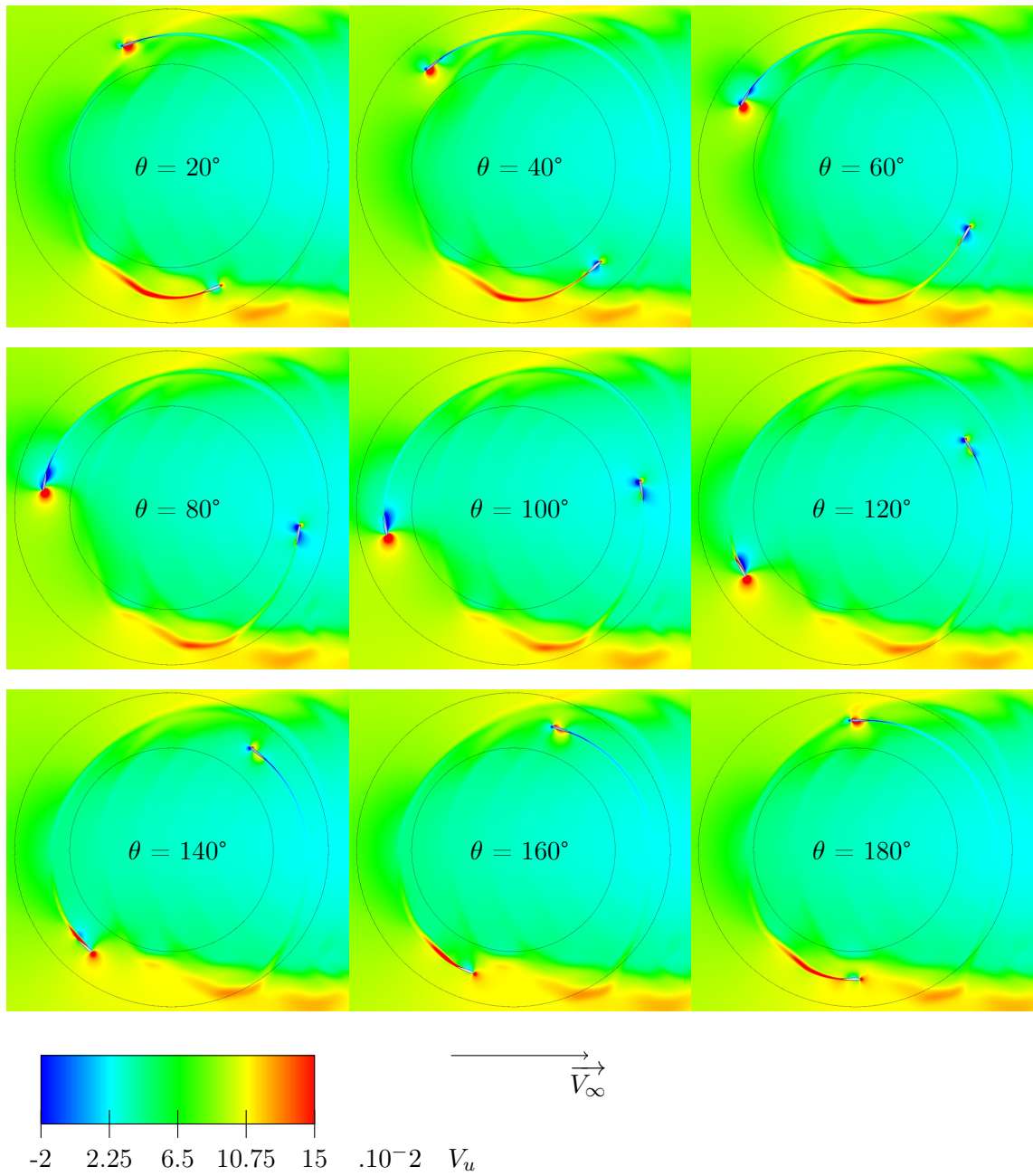
FIGURE 5.55 – Vitesse du fluide selon l'axe x pour le cas f3amoin1
