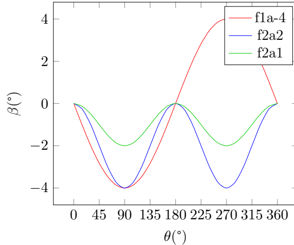
FIGURE 5.57 – lois de pas de f1a-4, f2a2 et f2a1
