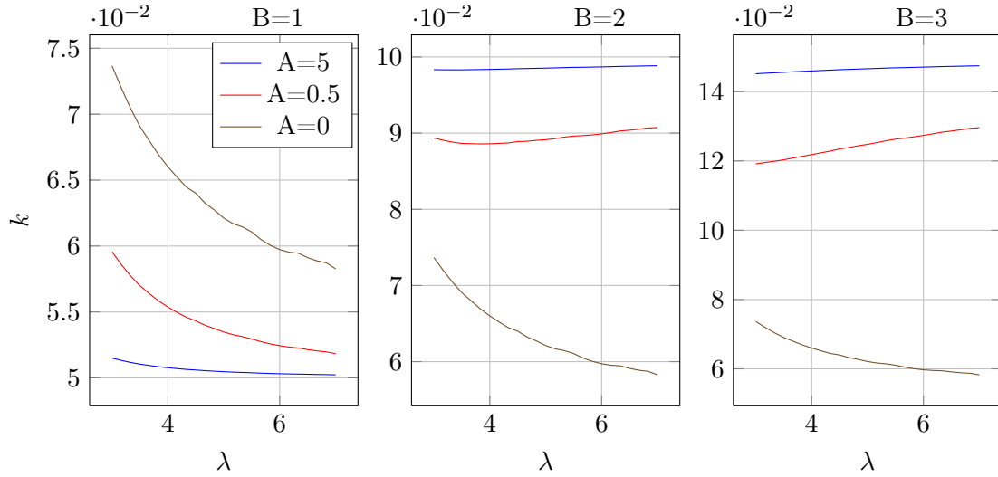
FIGURE 2.8 – Influence de \lambda , la fréquence et l’amplitude de variation d’une loi de pas sinusoïdale sur la fréquence réduite d’une turbine à axe transverse pour laquelle c/r = 1 . (A=0 : pas fixe)
