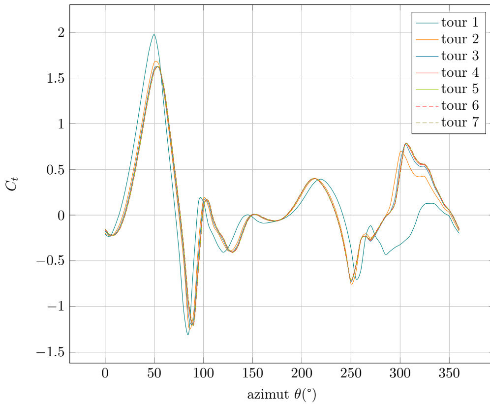
FIGURE 5.6 – Etude de convergence de sillage dans le cas C, \lambda = 2.5 table 2.2
