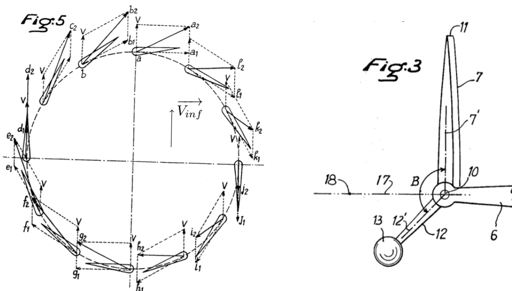
FIGURE 1.6 – Schémas du système Sicard issus de [Sicard 1977]
