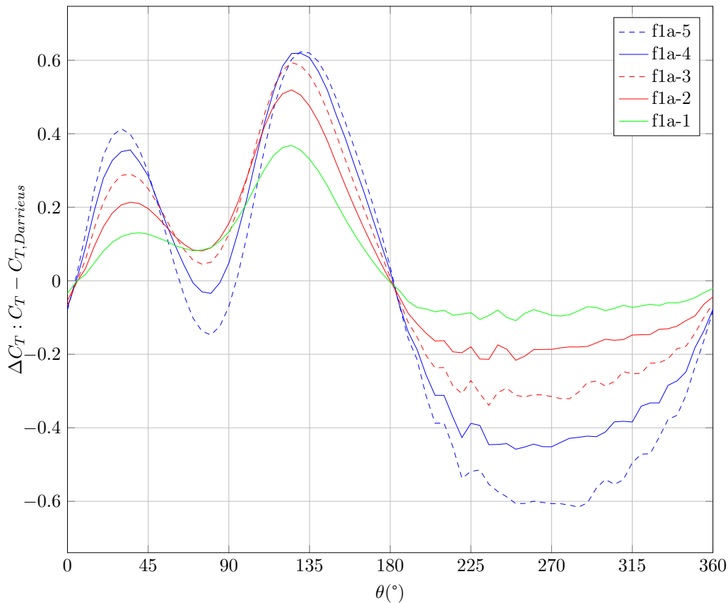
FIGURE 5.39 – Différence entre loi de pas variable et Darrieus pour le coefficient d'effort tangentiel, cas D, \lambda = 5
