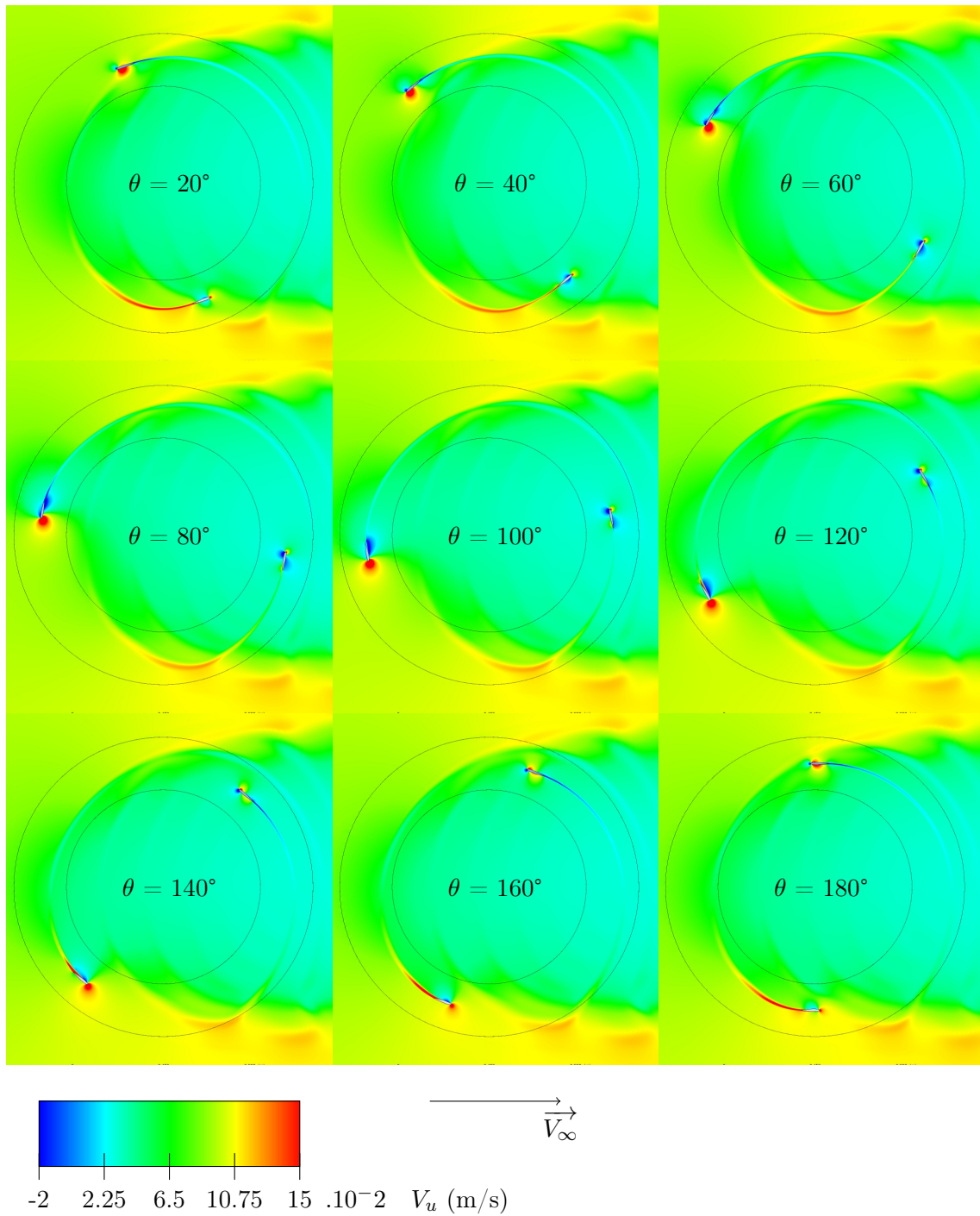
FIGURE 5.26 – Champs de vitesse projeté sur l’axe horizontal pour le système Darrieus cas D, \lambda = 5
