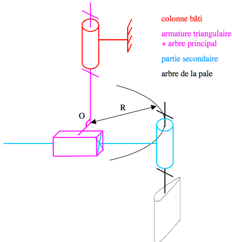
FIGURE D.1 – Schéma cinématique minimal du prototype SHIVA
