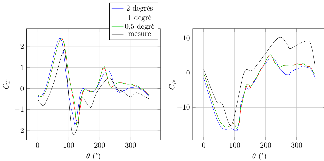
FIGURE 5.9 – Étude de convergence sur le pas angulaire
