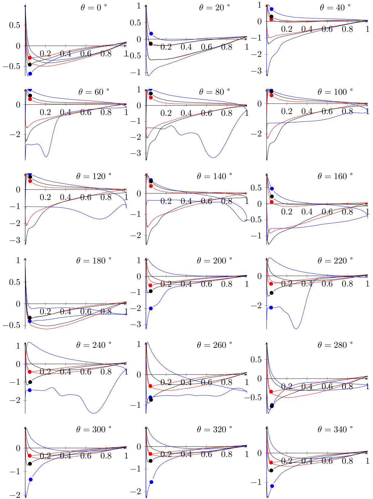
FIGURE C.2 – Coefficient de pression pour les cas C, D et E, Re = 10^4
