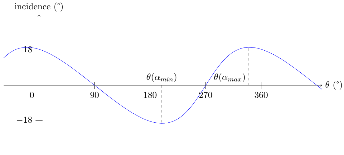
FIGURE 2.18 – Incidence géométrique au quart de corde pour \lambda=3
