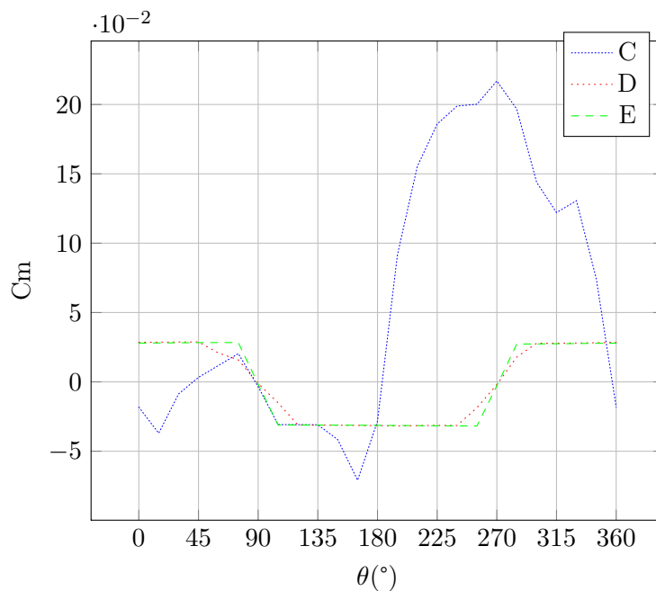
FIGURE 4.34 – Coefficients de moments calculés par le modèle ONERA-EDLIN pour les cas C, D et E
