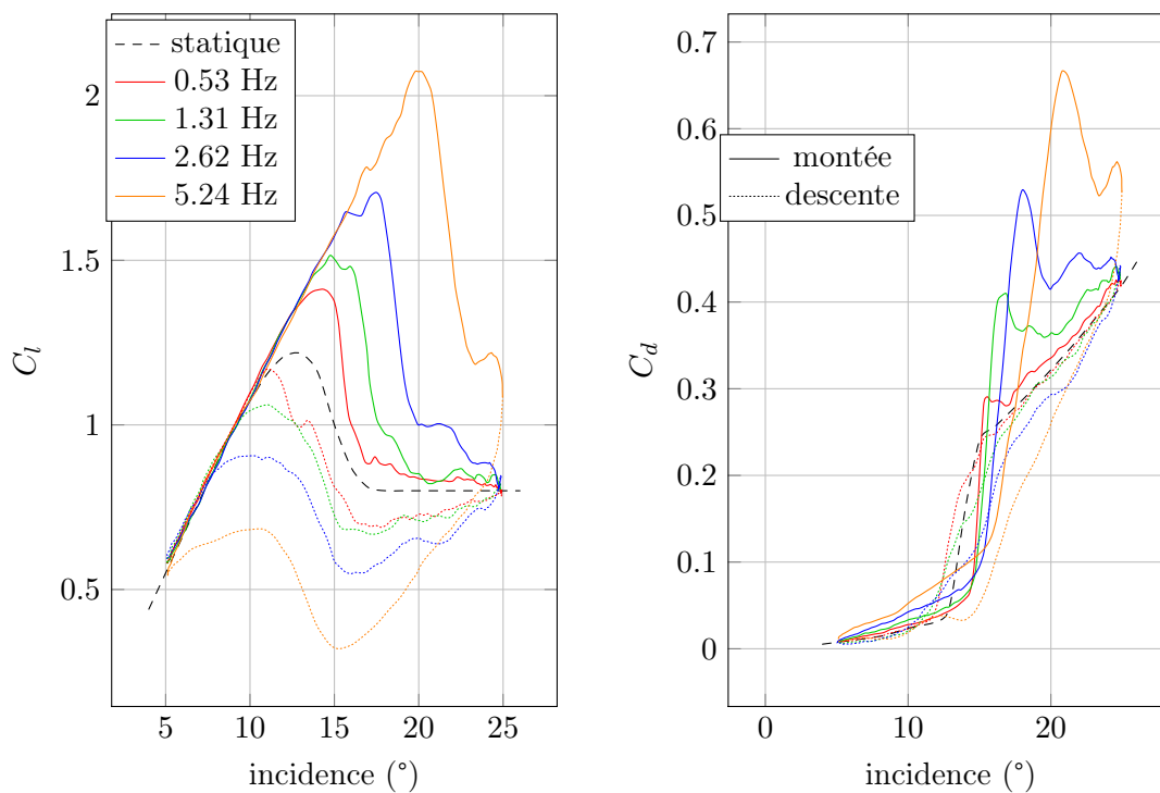
FIGURE 3.5 – Effets dynamiques sur les coefficients aérodynamiques en régime décroché
