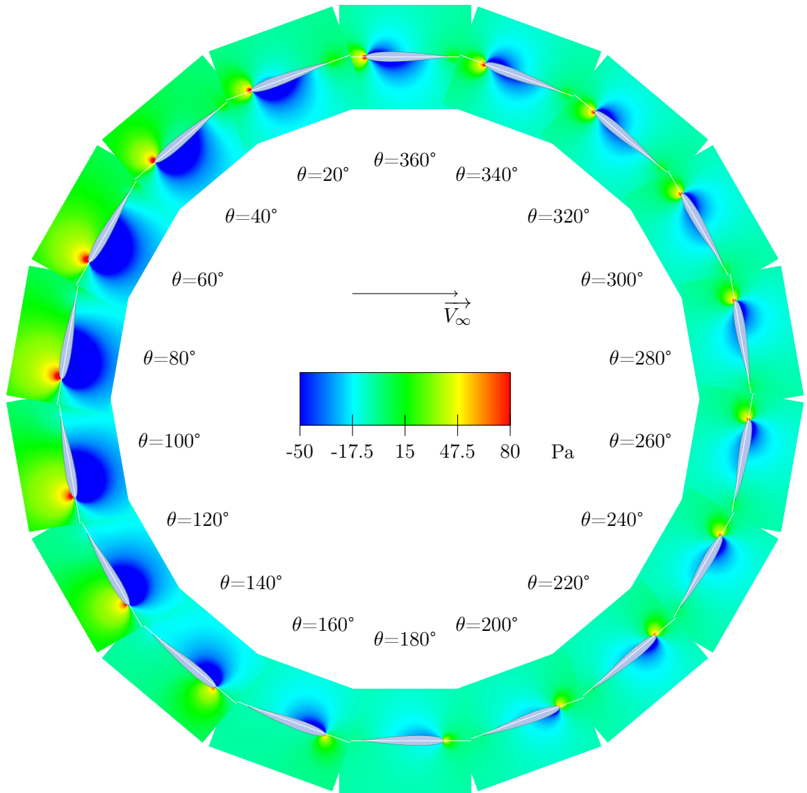
FIGURE 5.22 – Champs de pression pour un pas fixe, cas D, \lambda = 5
