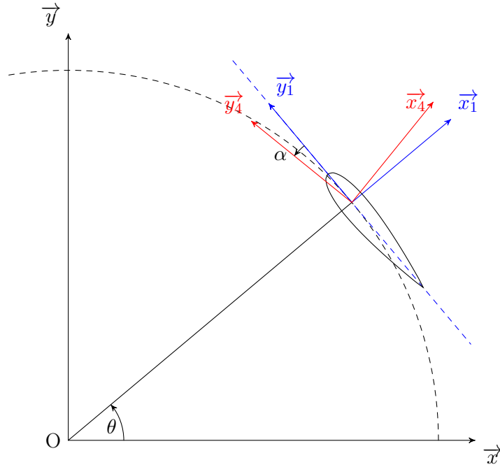
FIGURE 2.5 – Description des différents repères de projection des efforts hydrodynamiques
