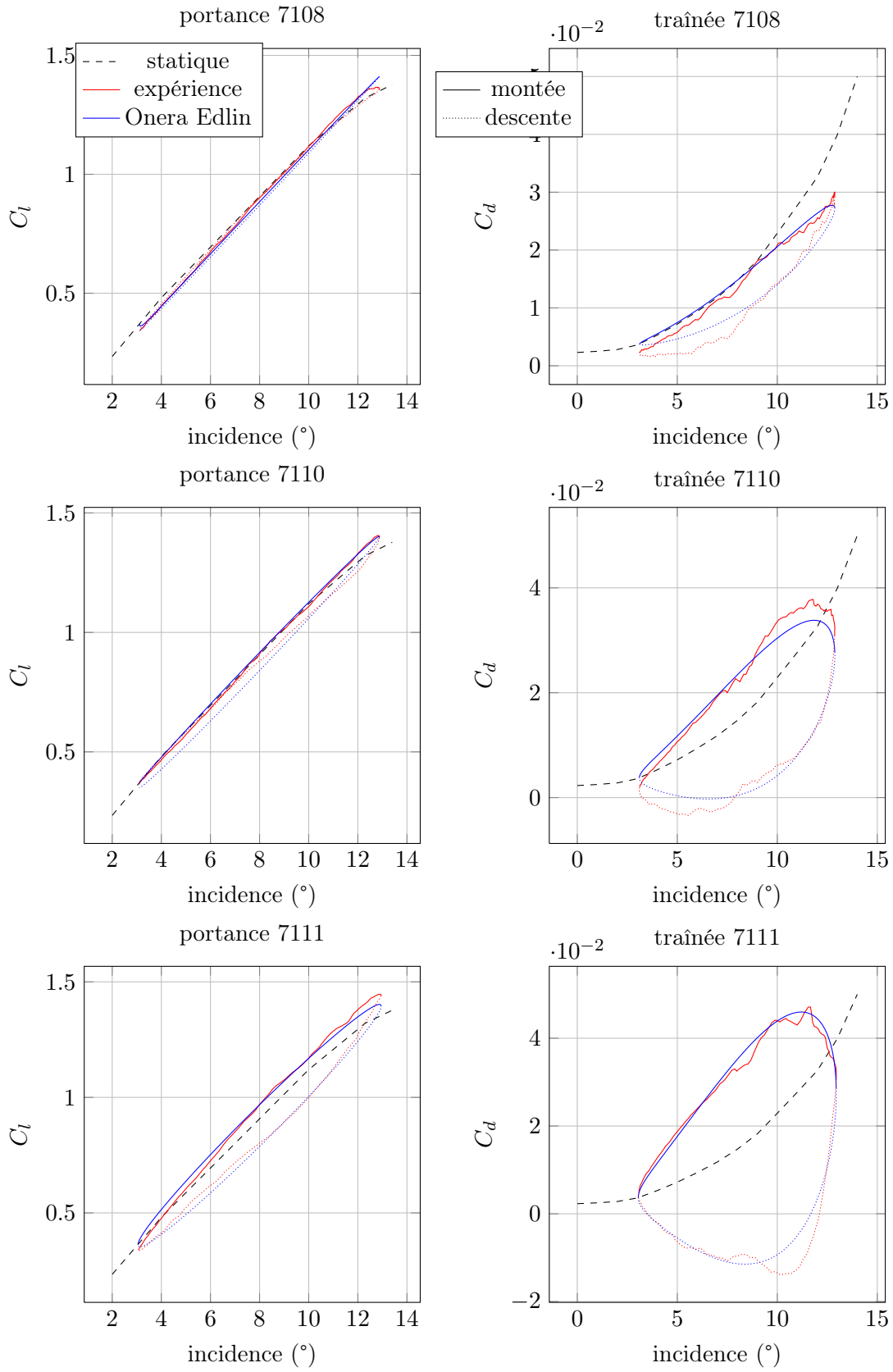
FIGURE 3.15 – Comparaison numérique expérience en décrochage léger
