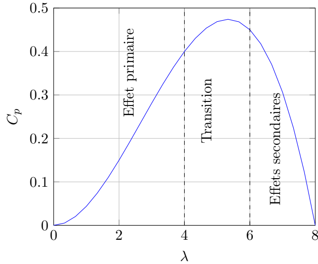
FIGURE 2.9 – Les différents domaines de fonctionnement d’un système Darrieus
