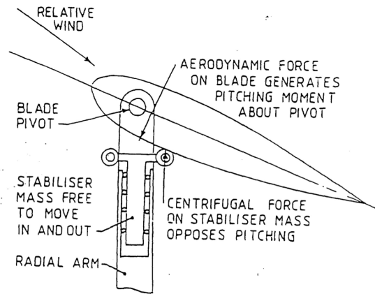
FIGURE 1.9 – Schéma du système Kirke/Lazauskas issu de [Lazauskas and Kirke 1992]
