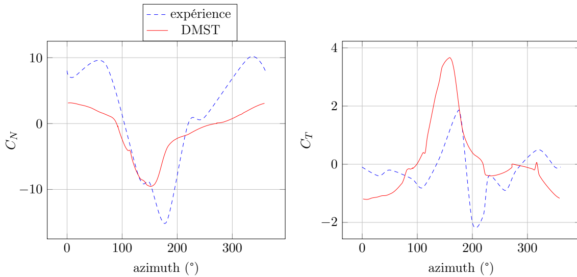
FIGURE 4.10 – Validation DMST pour le cas A : 2 pales, \lambda=3
