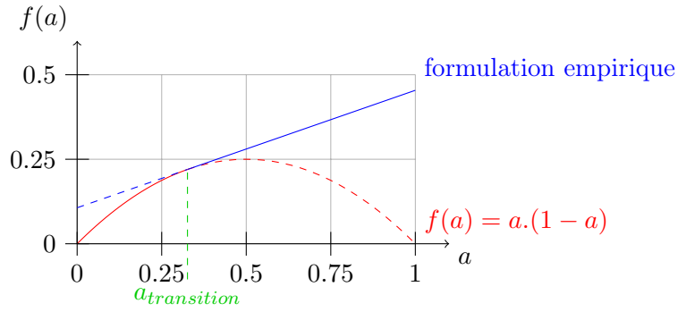
FIGURE 4.9 – Tracé de la formulation empirique de C_a en fonction de a
