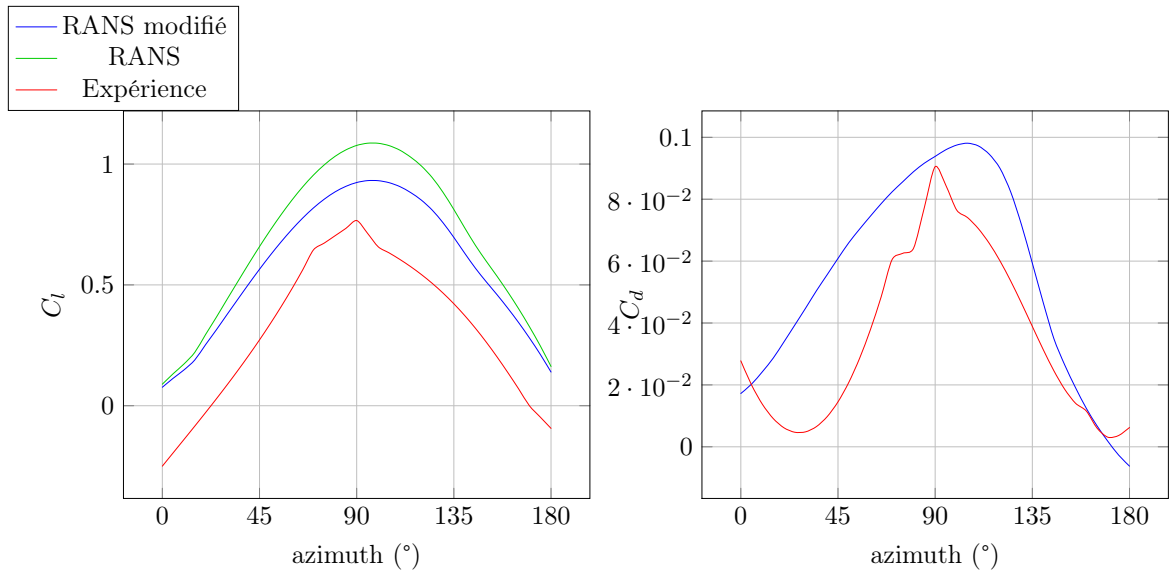
FIGURE 5.20 – Comparaison portance/trainée pour le cas D à l’amont, \lambda=5
