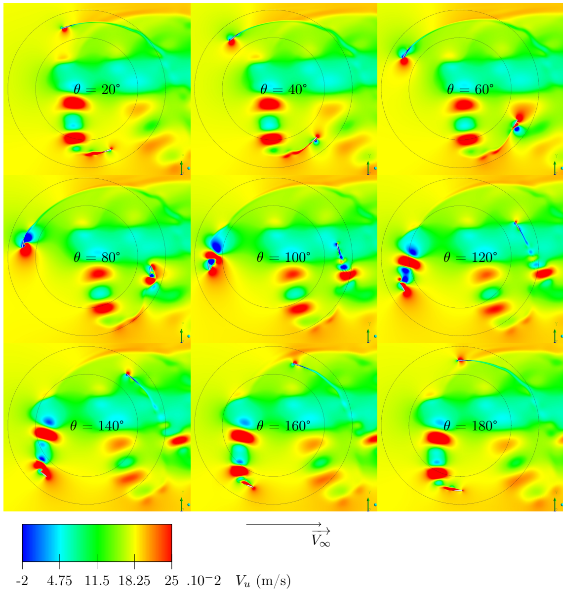
FIGURE 5.25 – Champs de vitesse projeté sur l’axe horizontal pour le système Darrieus cas C, \lambda = 2.5
