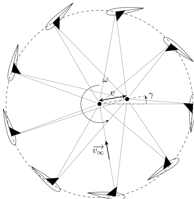
FIGURE 1.19 – Schéma du système Voith Schneider avec e = \frac{r}{3}
