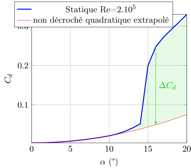
FIGURE 3.13 – Shématisation des éléments statiques de traînée
