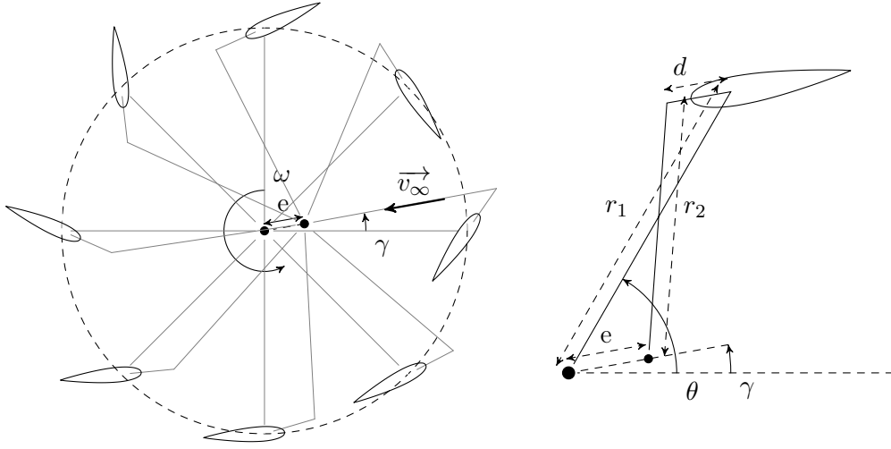
FIGURE 1.22 – Schéma général du système Pinson
