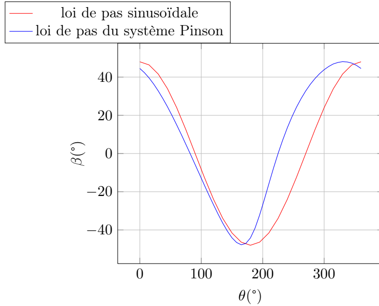
FIGURE 1.24 – Evolution du calage pour le système Pinson avec \gamma = 0 , r_1 = r_2 = 1 , e = 0.35 et d = 0.5
