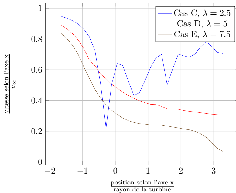
FIGURE 5.24 – Ralentissement du fluide pour les pas fixe à l'ordonnée nulle
