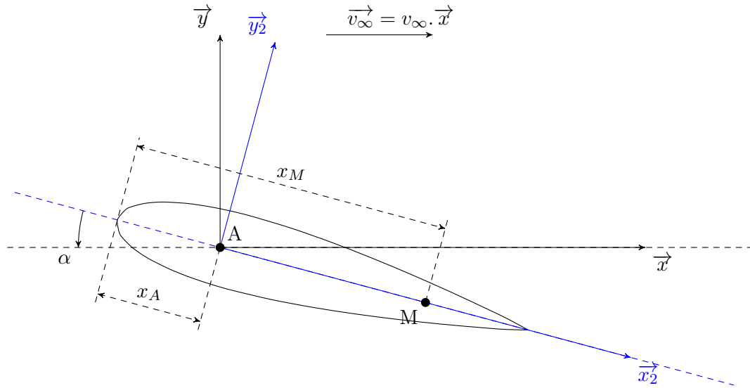
FIGURE 3.7 – Repère d'étude utilisé dans la mise en tangage sinusoïdale d'un profil
