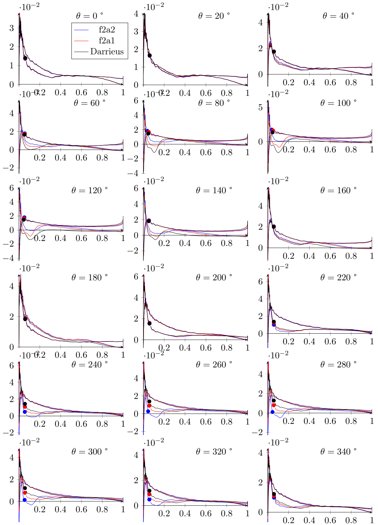
FIGURE C.7 – Coefficient de frottement à la paroi pour les cas f2a2 et f2a1
