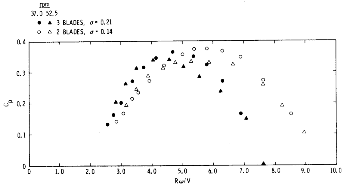
FIGURE 2.2 – Figure originale de variation du coefficient de performance avec la solidité mesuré sur la turbine DOE/Sandia. Reproduit de [Worstell 1980]
