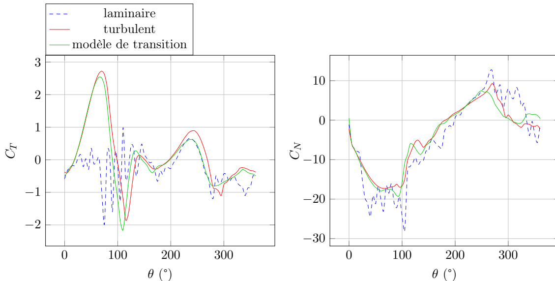
FIGURE 5.10 – Etude de modèle fluide pour le tour 2 du cas A
