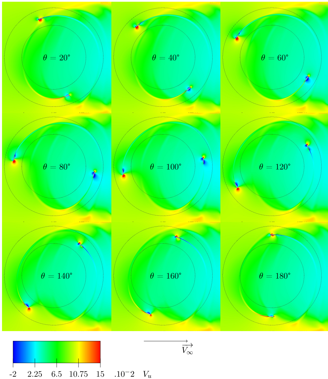
FIGURE 5.65 – Vitesse du fluide selon l'axe x pour le cas f2a2, \lambda = 5
