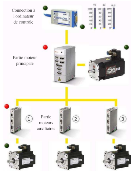
FIGURE D.4 – Schéma du contrôle des différentes rotations du système
