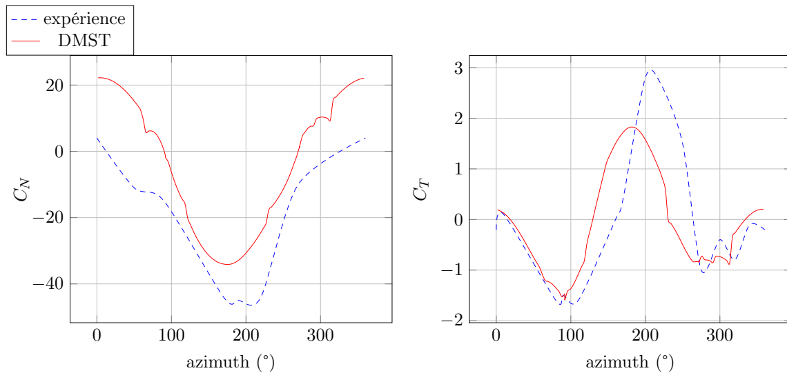
FIGURE 4.15 – Validation DMST pour le cas E : 2 pales, \lambda=7.5
