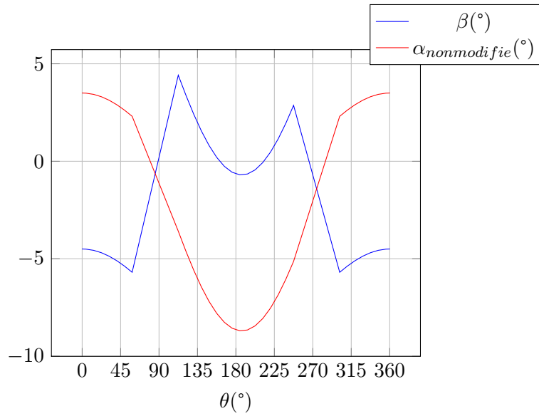
FIGURE 4.36 – Loi de pas idéale
