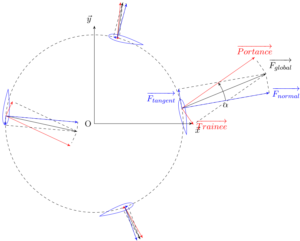
FIGURE 2.22 – Projection des efforts sur le repère lié à la pale
