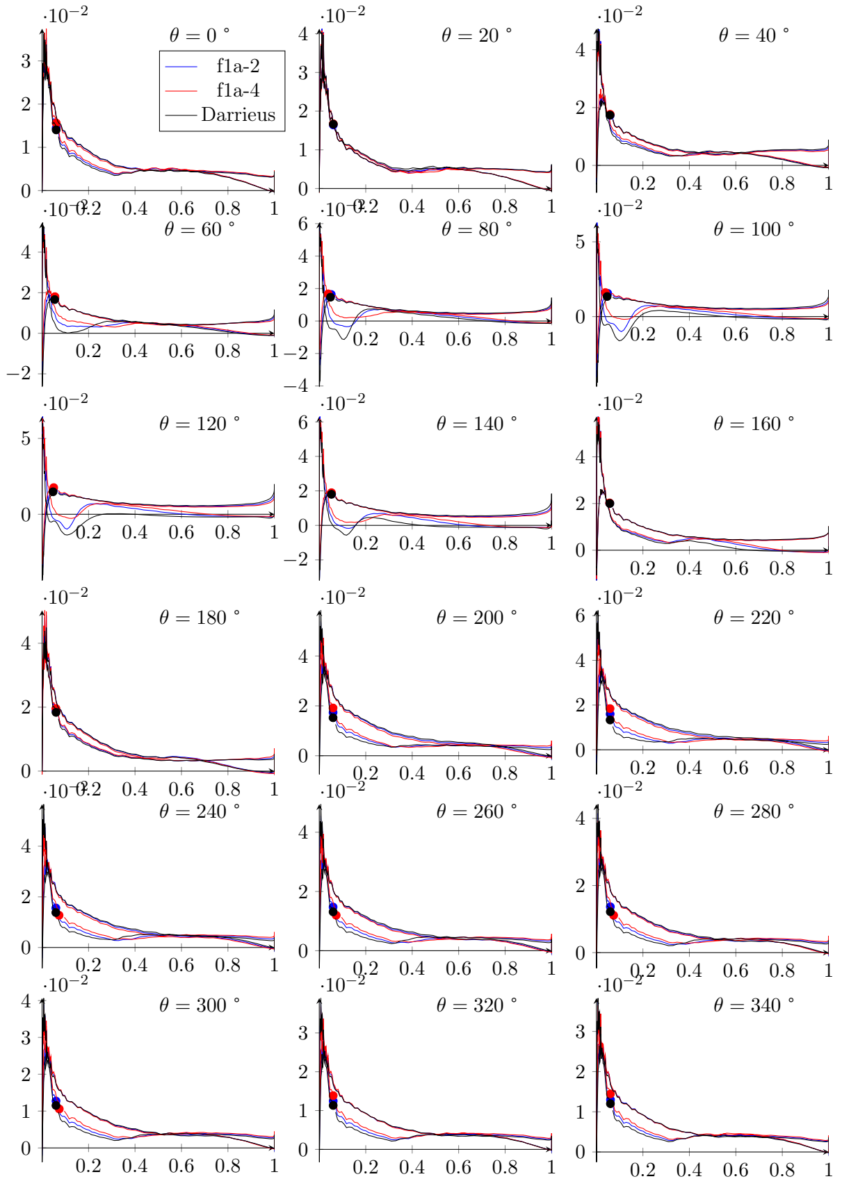
FIGURE C.3 – Coefficient de frottement à la paroi pour les cas fla-2 et fla-4
