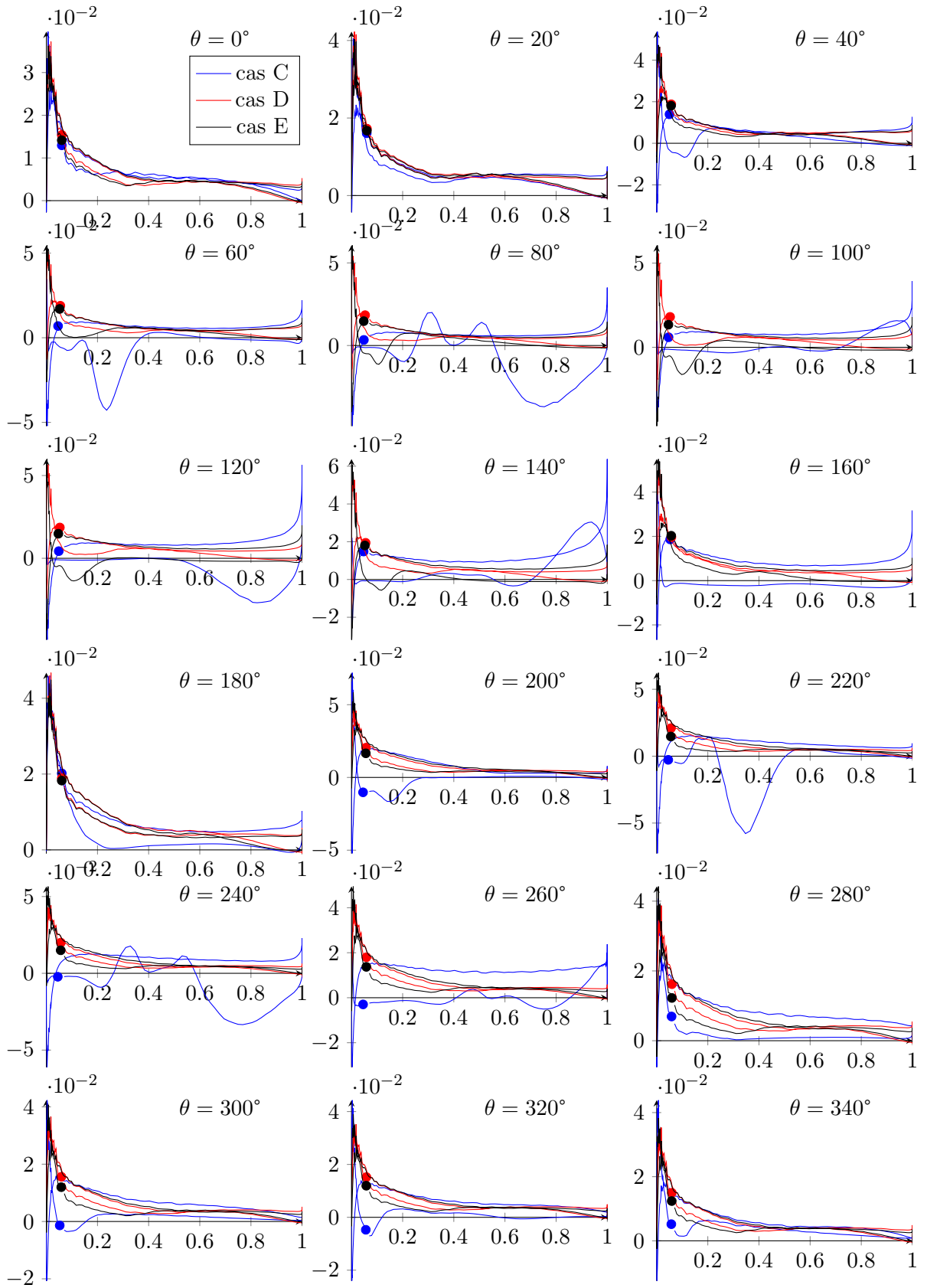
FIGURE C.1 – Coefficient de frottement à la paroi pour les cas C, D et E, Re = 10^4
