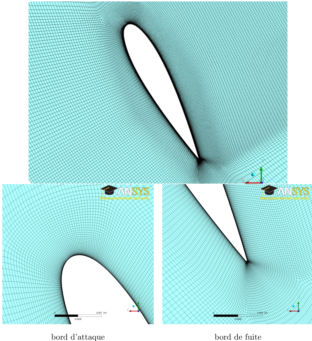
FIGURE 5.3 – Vue de la région proche paroi du maillage
