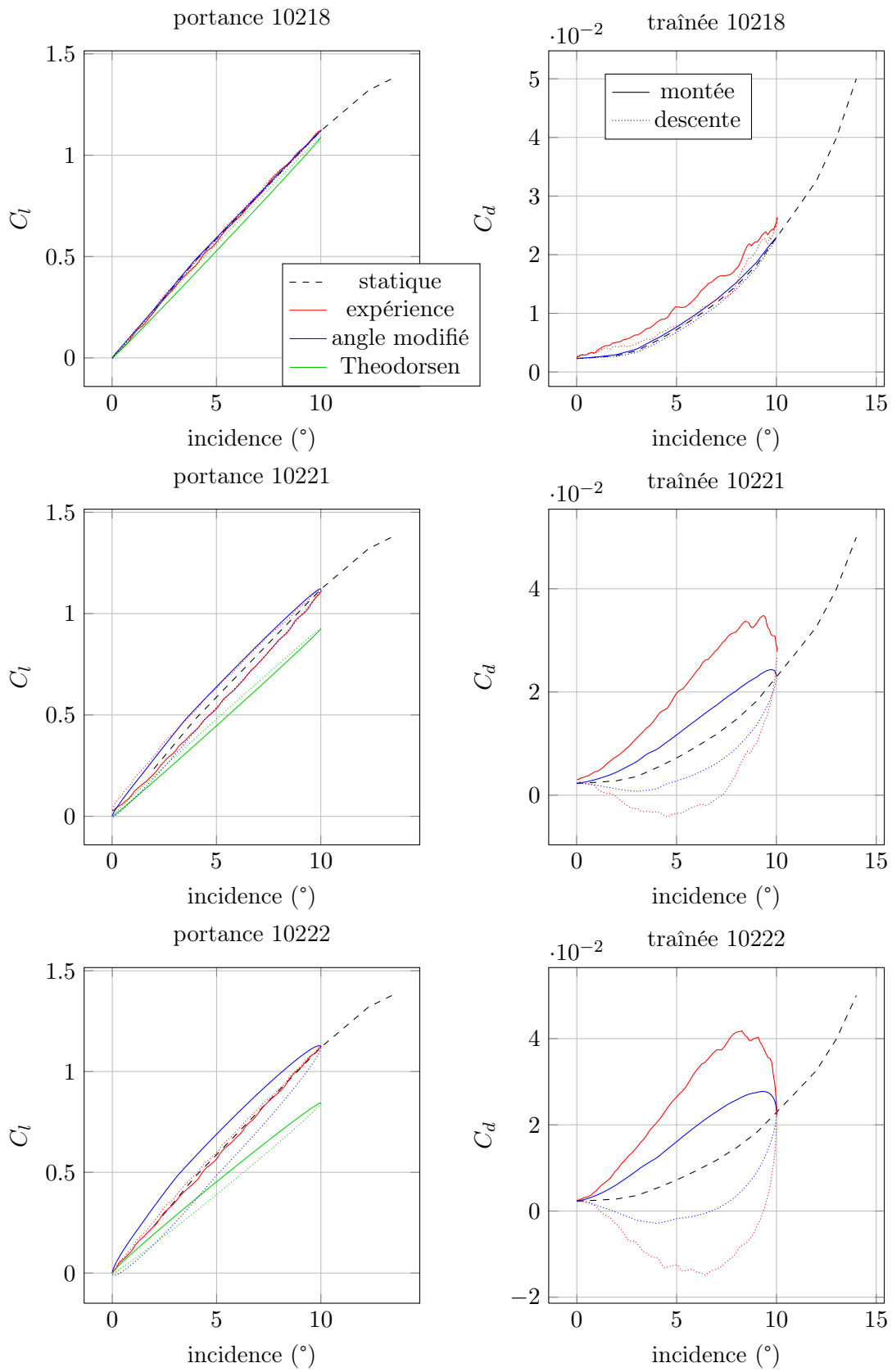
FIGURE 3.9 – Comparaison numérique expérience en écoulement accroché
