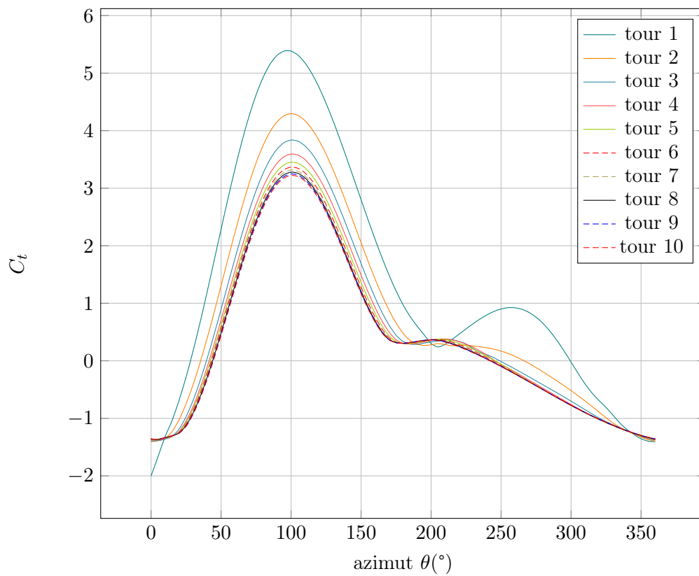
FIGURE 5.8 – Etude de convergence de sillage dans le cas E, \lambda = 7.5 table 2.2
