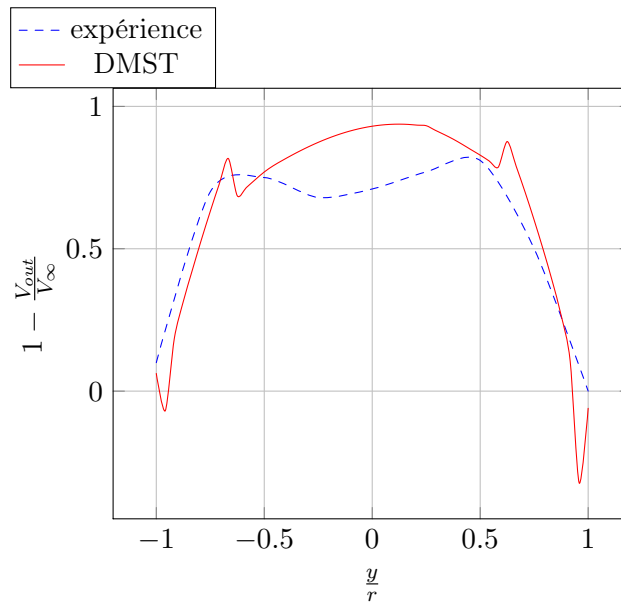
FIGURE 4.14 – Comparaison numérique-expérience du déficit de vitesse en aval du rotor
