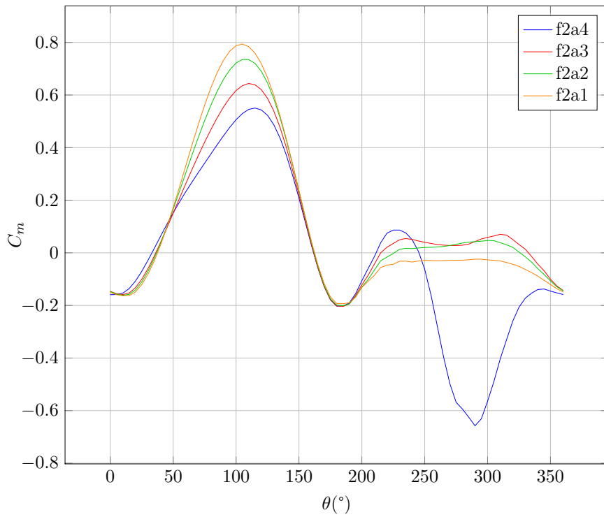
FIGURE 5.66 – Coefficients de moment pour les fonctions f2, \lambda = 5
