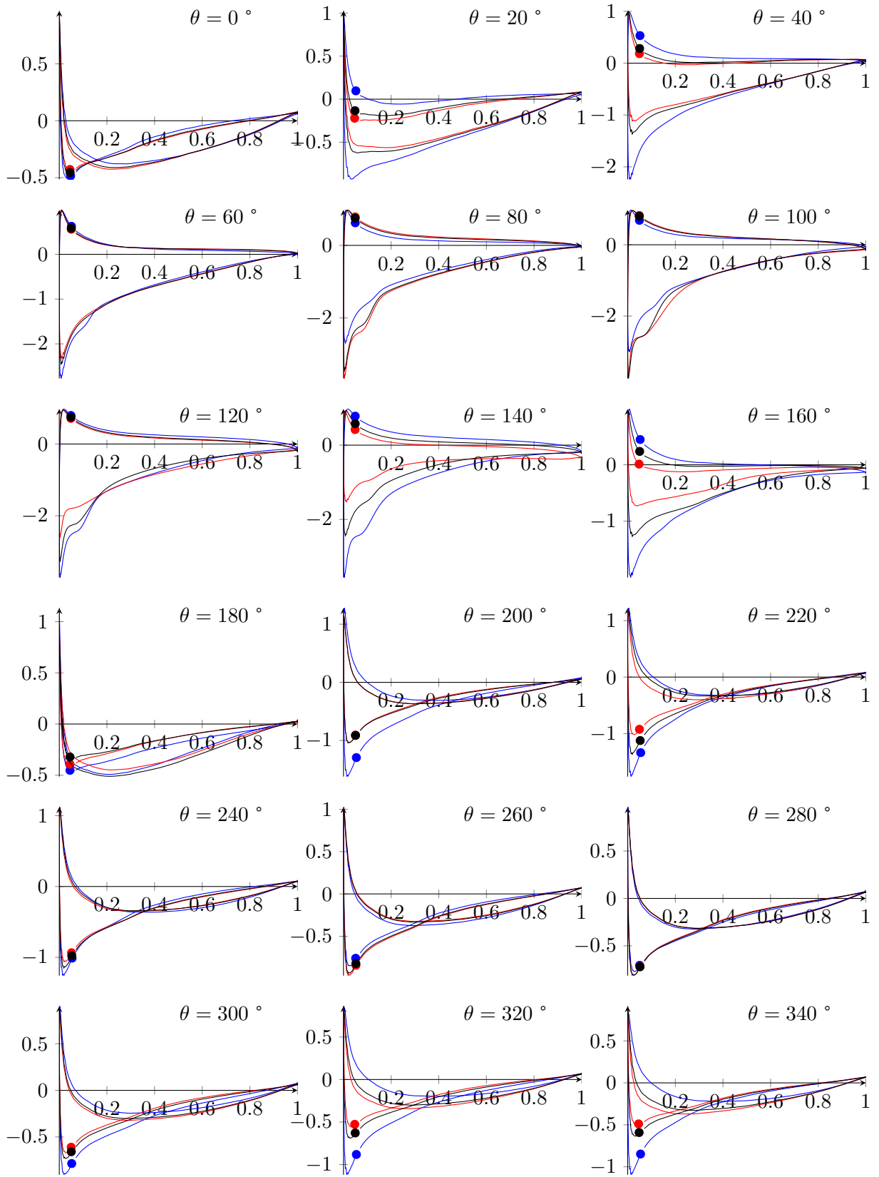
FIGURE C.6 – Coefficient de pression pour les cas f3a3 et f3a-1
