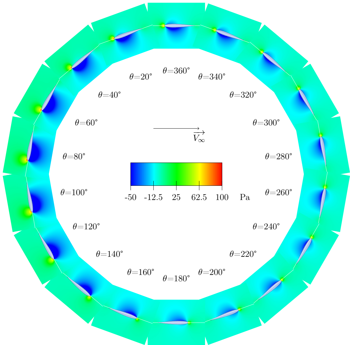
FIGURE 5.23 – Champs de pression pour un pas fixe, cas E, \lambda = 7.5
