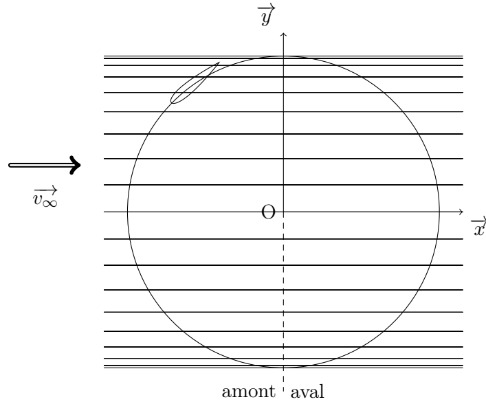
FIGURE 4.1 – La décomposition du domaine fluide en tubes à intervalles angulaires égaux
