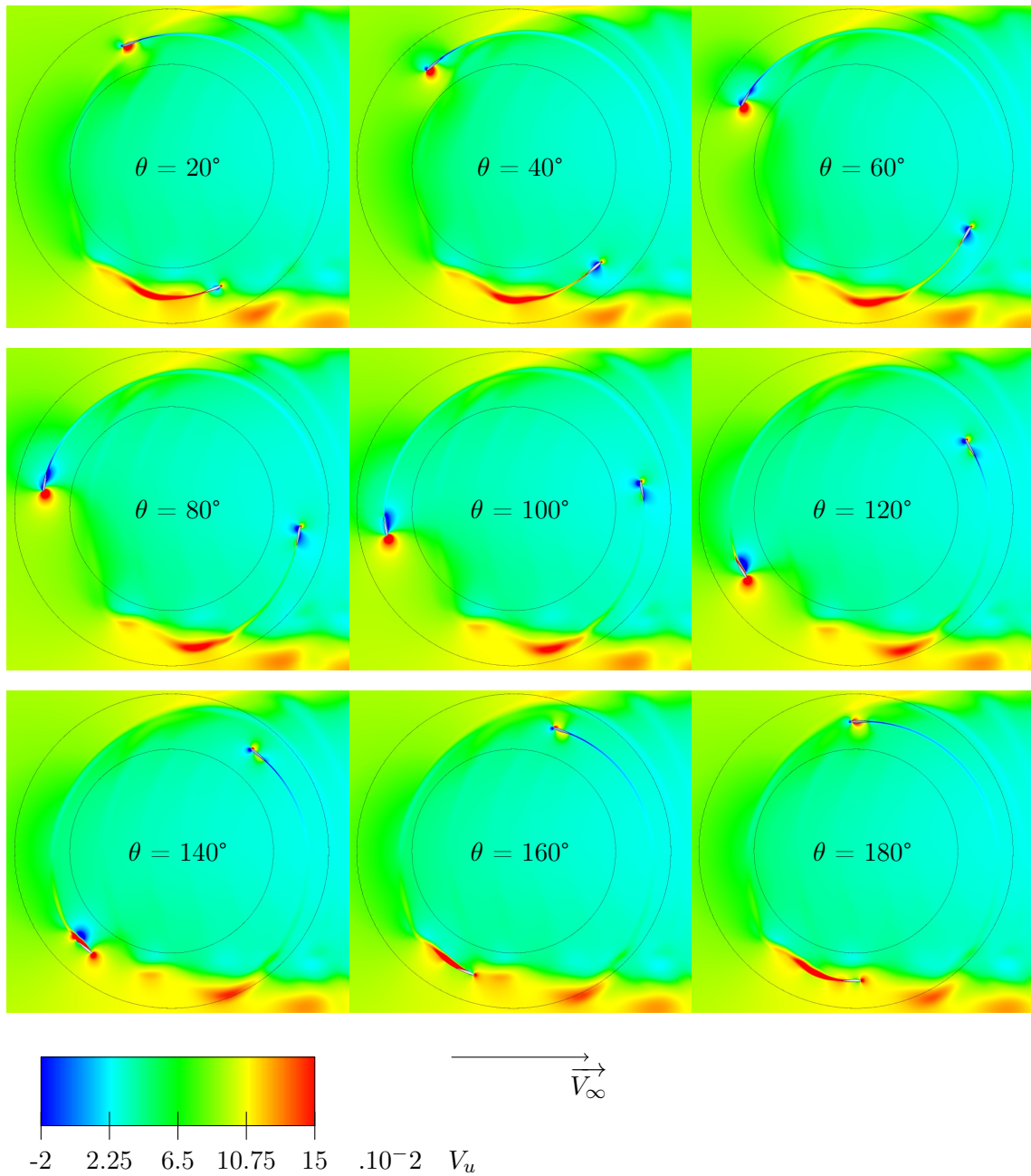
FIGURE 5.35 – Vitesse du fluide selon l'axe x pour le cas fl1a1, \lambda = 5
