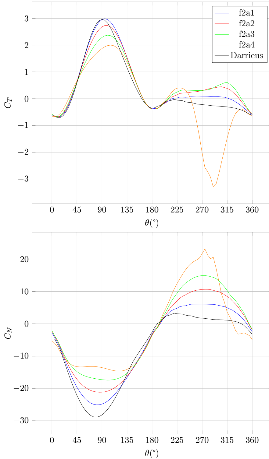
FIGURE 5.58 – Résultats d'efforts pour des lois de pas de fréquence égale à la deux fois la fréquence machine, \lambda = 5
