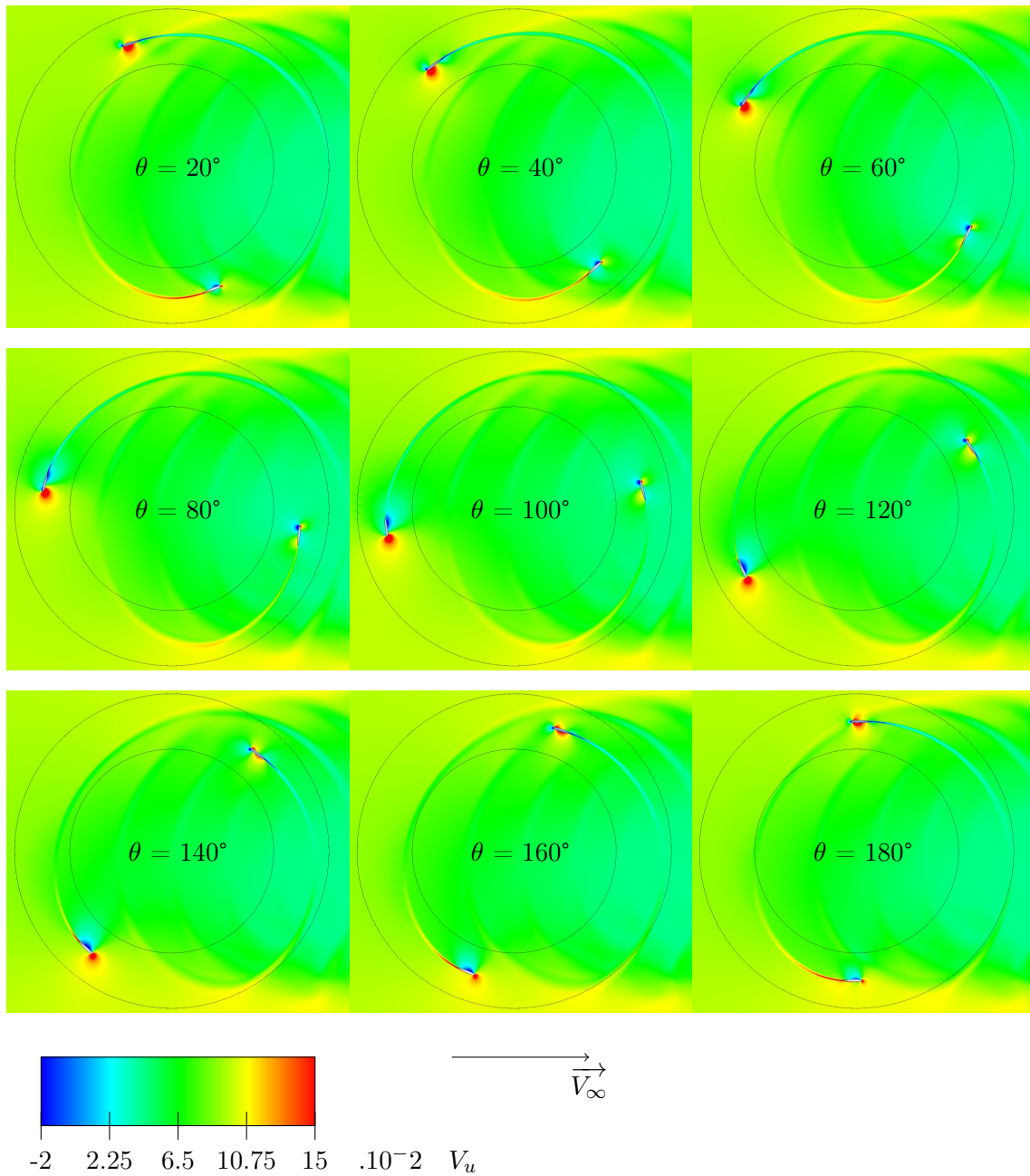
FIGURE 5.45 – Vitesse du fluide selon l’axe x pour le cas flamins4, \lambda = 5
