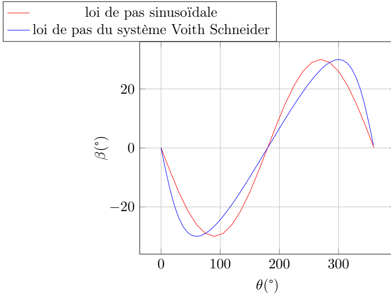
FIGURE 1.20 – Evolution du calage pour e = \frac{r}{2} pour le système Voith-Schneider
