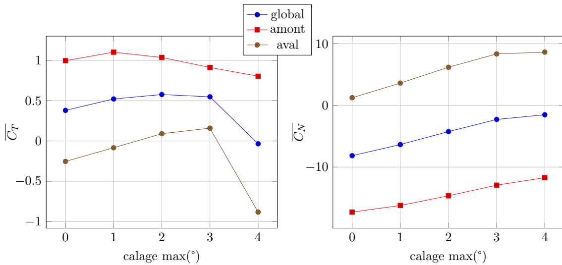
FIGURE 5.60 – Evolution de la moyenne des coefficients d’effort en fonction de l’amplitude de la loi de type f2 utilisée, \lambda = 5
