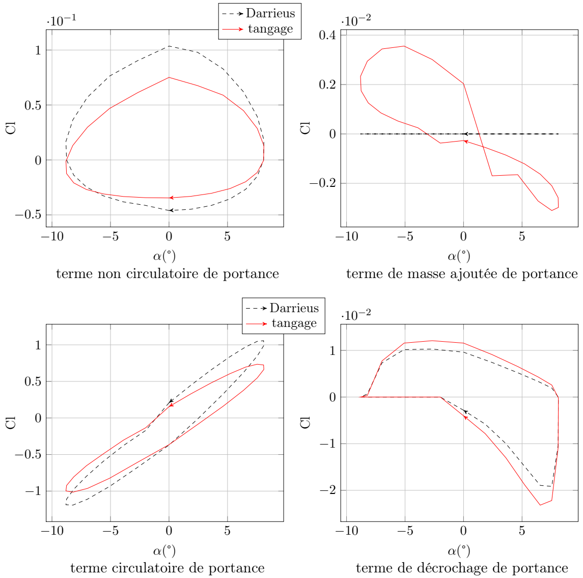
FIGURE 4.32 – Les différentes composantes de portance du modèle ONERA en tangage et Darrieus pour le cas D
