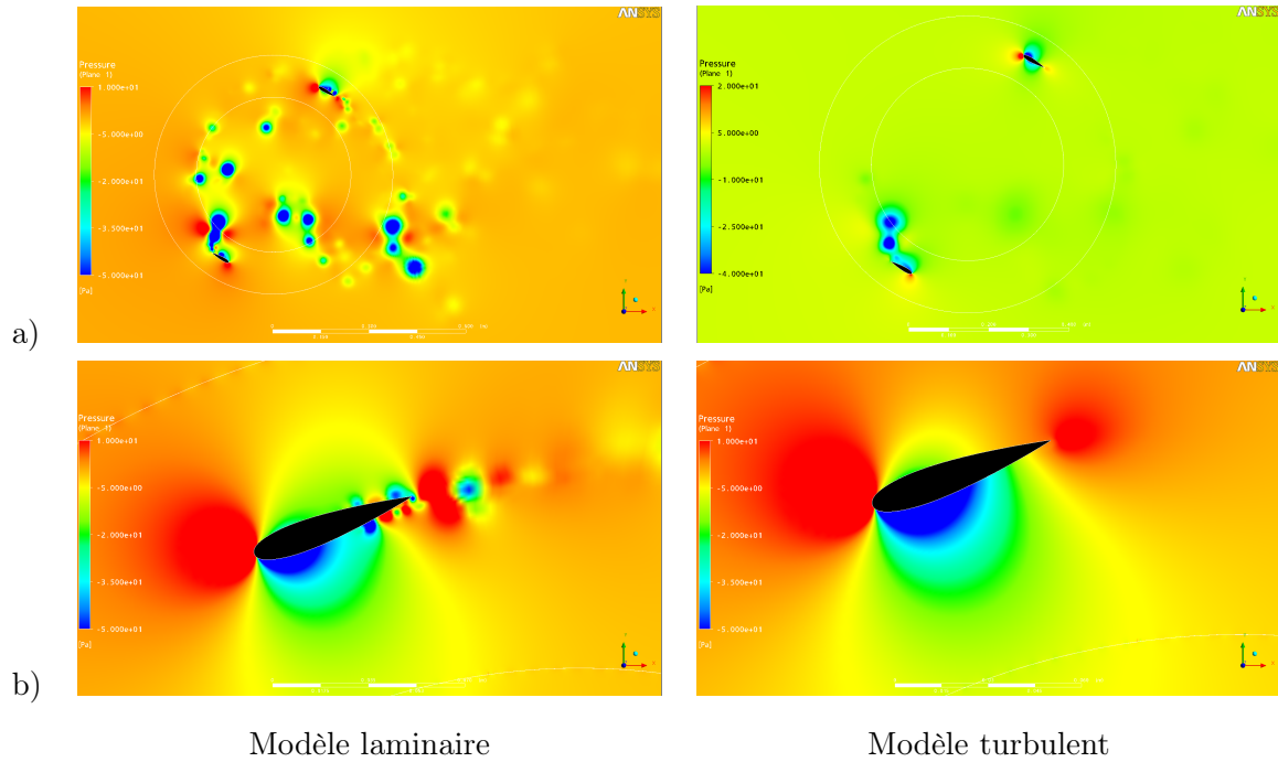
FIGURE 5.11 – Champ de pression pour deux modèles pour le cas A à \theta=40^\circ . a) champ global, b) vue rapproché d’une pale
