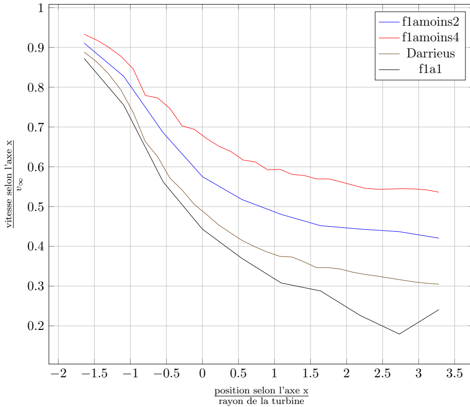
FIGURE 5.46 – Ralentissement du fluide pour les cas fl1a-2 et fl1a-4 à l'ordonnée nulle, cas D, \lambda = 5
