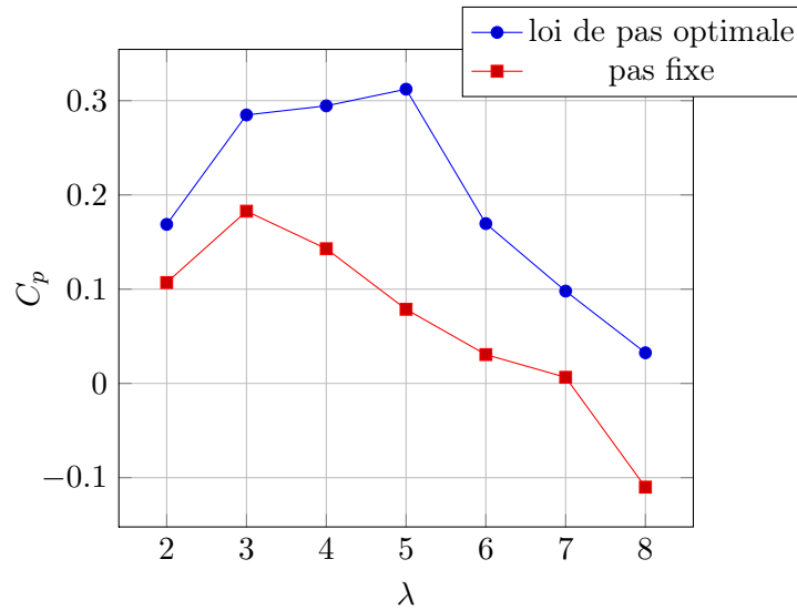
FIGURE 4.20 – Variations des performances obtenues avec une loi de pas idéale
