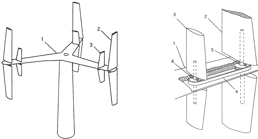
FIGURE 1.8 – Schémas du système Verastegui issus de [Verastegui 1996]
