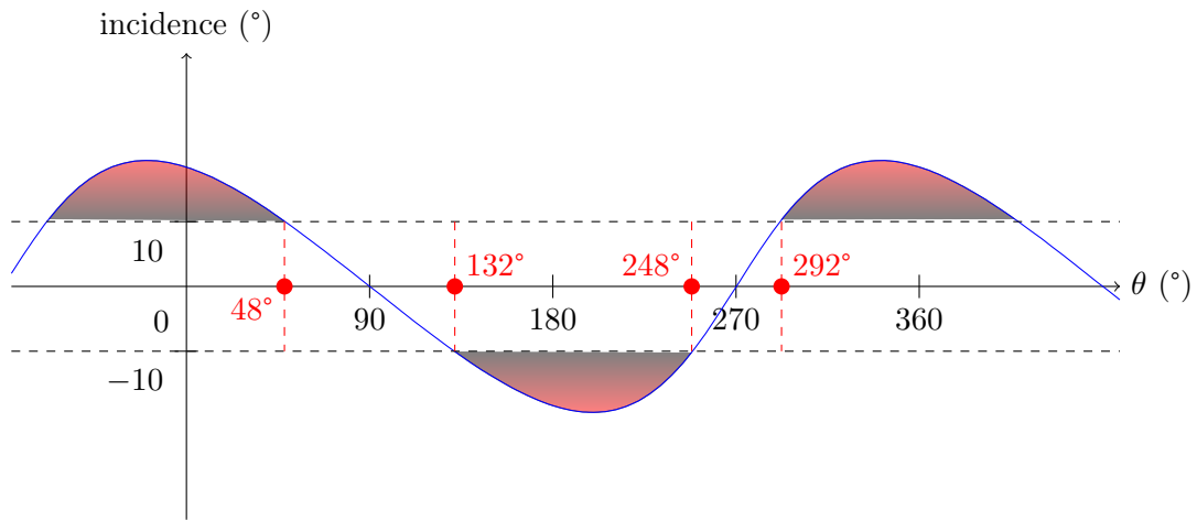
FIGURE 2.20 – Zones décrochées pour \lambda = 3
