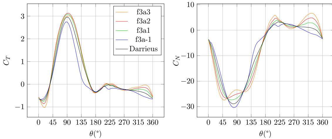
FIGURE 5.47 – Résultats d’effort pour des lois de pas de fréquence égale à la trois fois la fréquence machine, cas D, \lambda = 5
