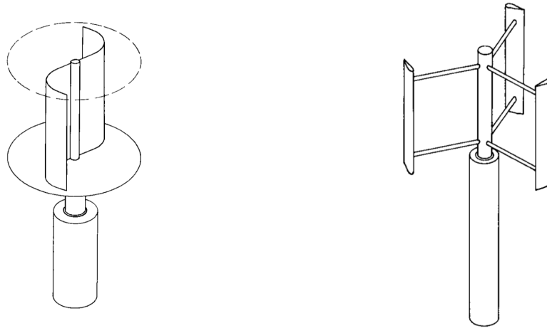
FIGURE 1.3 – Vues en perspective du système Savonius à gauche et Darrieus à droite
