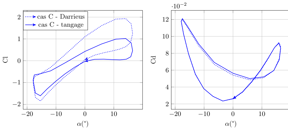
FIGURE 4.28 – Comparaison tangage simple/Darrieus pour le cas C
