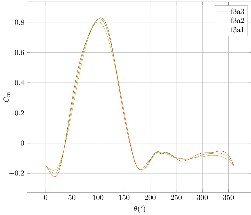
FIGURE 5.68 – Coefficients de moment pour les fonctions f3, \lambda = 5
