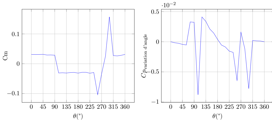
FIGURE 4.38 – Influence du moment hydrodynamique sur les performances lors de la variation d'angle
