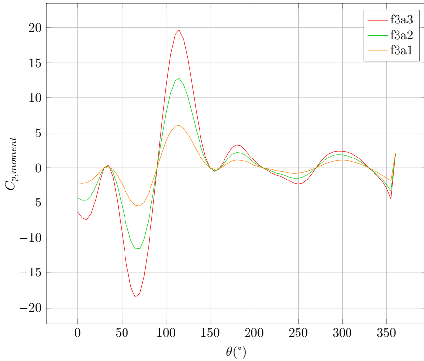
FIGURE 5.69 – influence du moment sur les coefficients de performance pour les fonctions f3, \lambda = 5
