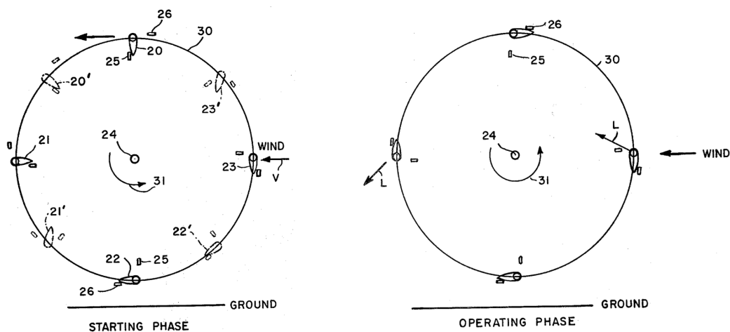
FIGURE 1.7 – Schémas du système Drees issus de [Drees 1979]
