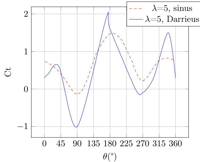
FIGURE 4.22 – efforts tangentiels comparés entre loi de pas sinusoïdale et Darrieus d’après le modèle DMST
