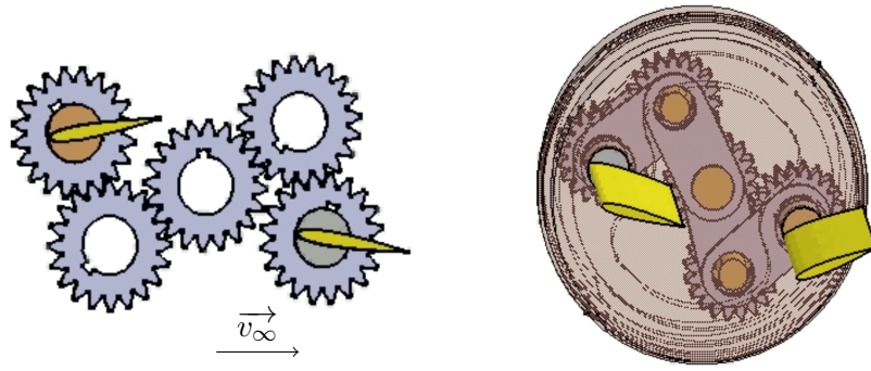
FIGURE 1.12 – Schémas du système Lipp
