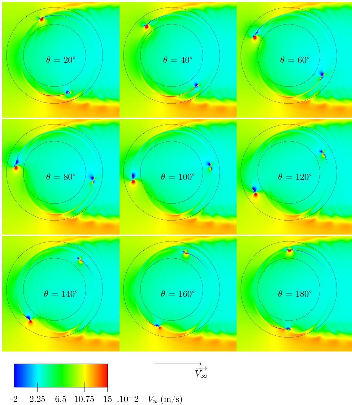
FIGURE 5.27 – Champs de vitesse projeté sur l’axe horizontal pour le système Darrieus cas E, \lambda = 7.5
