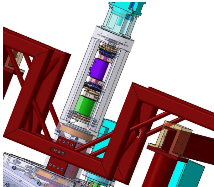
FIGURE D.5 – Implantation du collecteur tournant et du couplemètre
