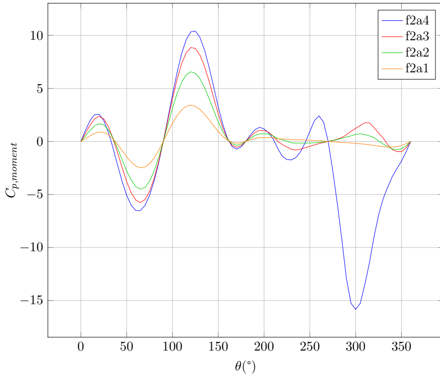
FIGURE 5.67 – influence du moment sur les coefficients de performance pour les fonctions f2, \lambda = 5
