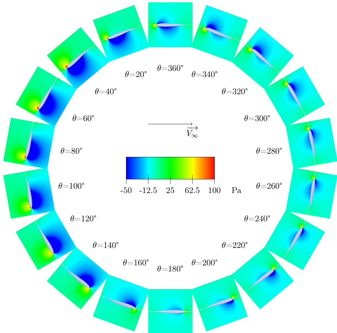
FIGURE 5.54 – champs de pression autour du foil dans le cas f3a3, \lambda = 5
