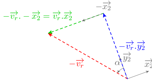
FIGURE 4.8 – Schéma des vecteurs formant l'incidence en un point du profil
