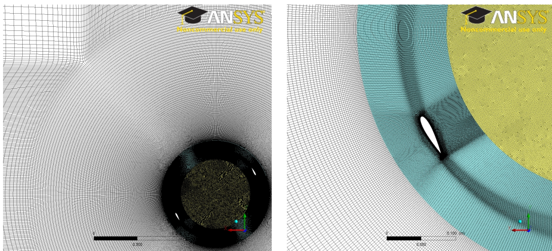
FIGURE 5.5 – Vue rapprochée de l'anneau de la turbine pour le maillage retenu
