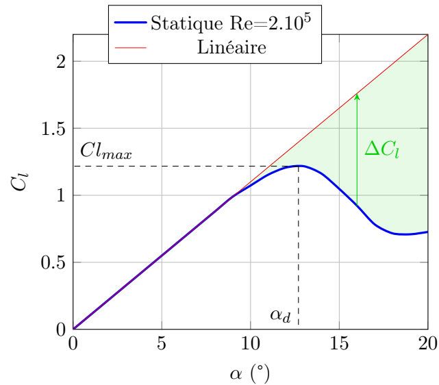
FIGURE 3.11 – Shématisation de la grandeur de mesure de décrochage en portance
