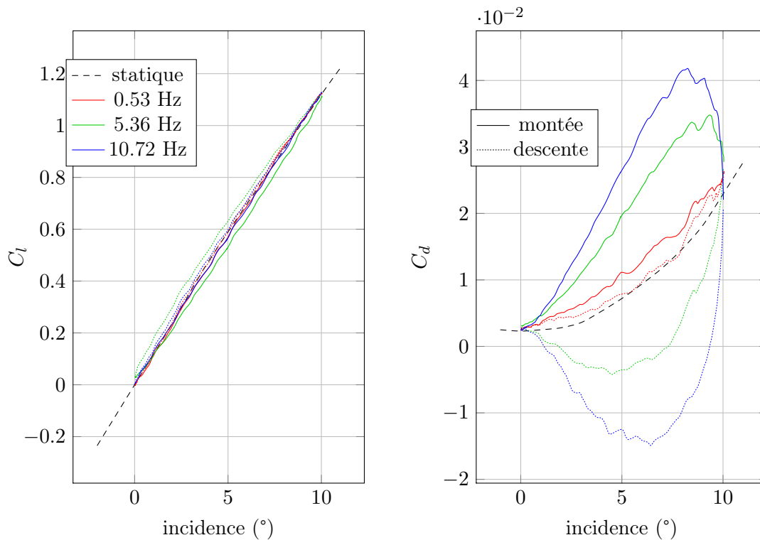
FIGURE 3.4 – Effets dynamiques sur les coefficients aérodynamiques en régime non décroché
