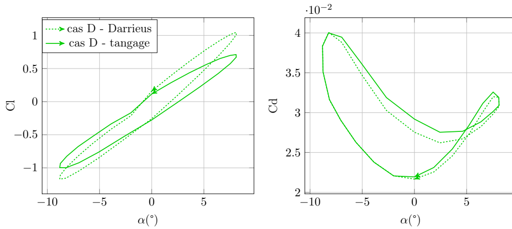
FIGURE 4.29 – Comparaison tangage simple/Darrieus pour le cas D
