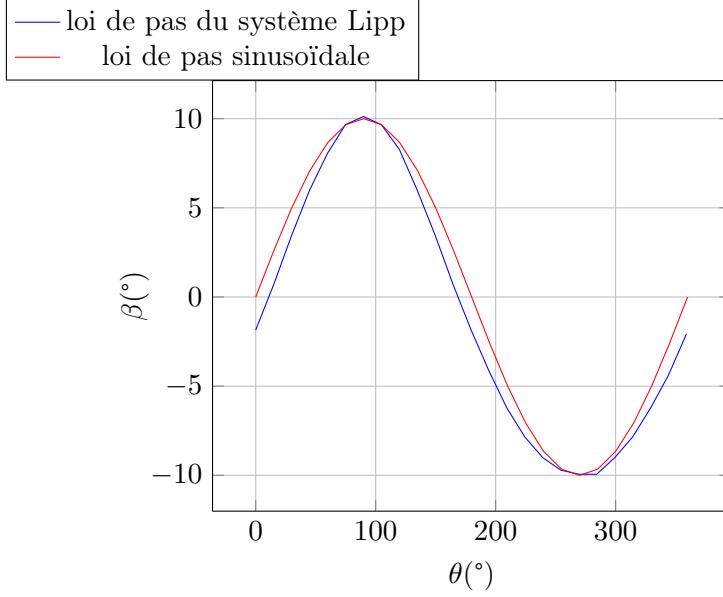
FIGURE 1.13 – Loi d’incidence du rotor Lipp pour \frac{R}{2(r+r_1)} = 0.11 , e/R = 0.4
