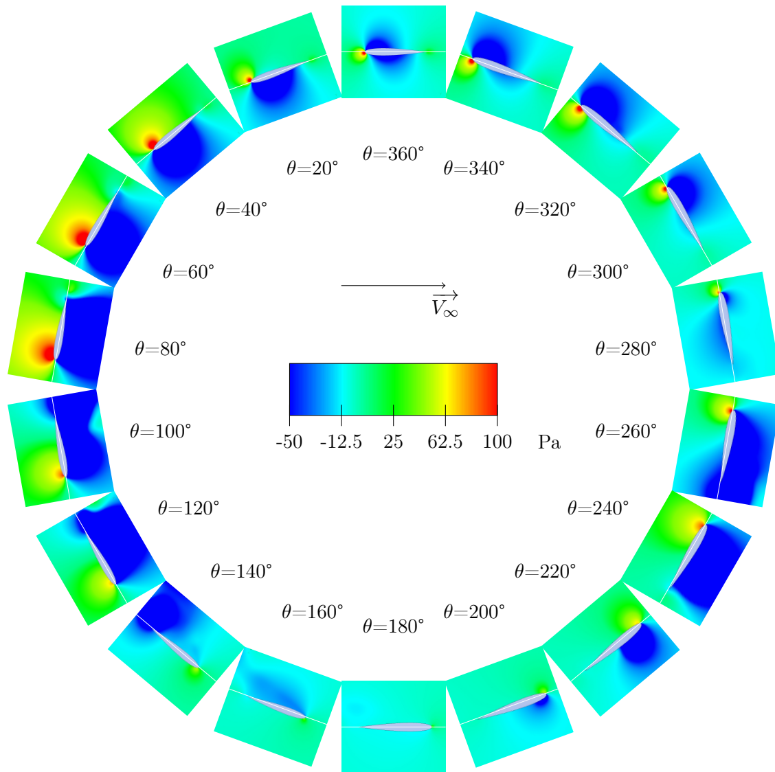
FIGURE 5.21 – Champs de pression pour un pas fixe, cas C, \lambda = 2.5
