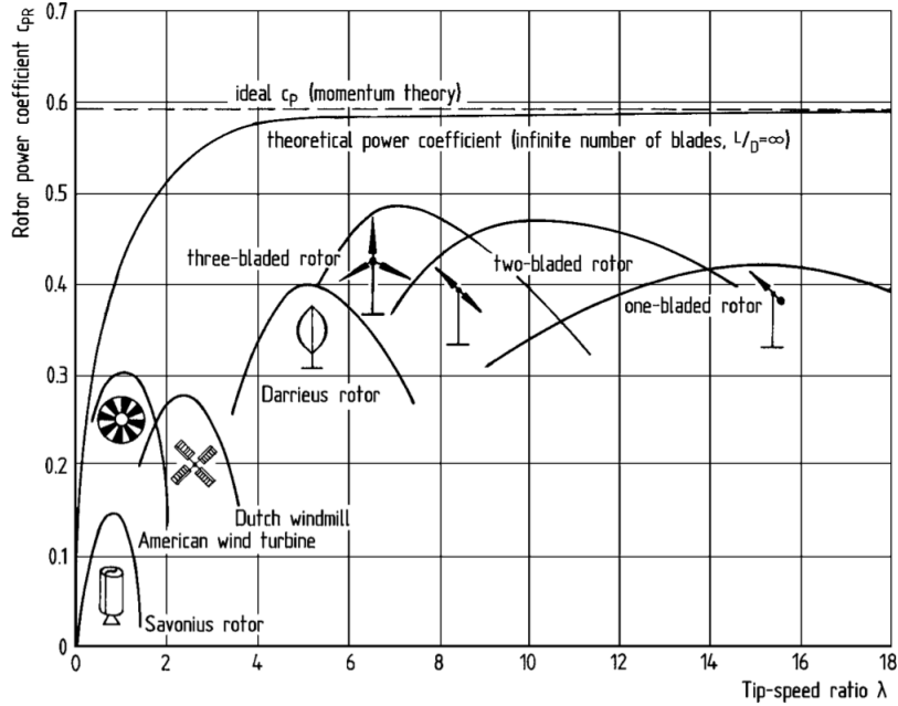
FIGURE 2.1 – Variation du coefficient de performance avec \lambda pour plusieurs systèmes. Reproduit de [Hau 2006]
