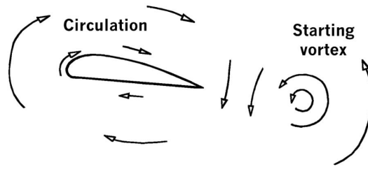
FIGURE 3.2 – Scématisation d'un changement de quantité de circulation autour d'un profil dû à une augmentation d'angle d'attaque, et influence sur le sillage
