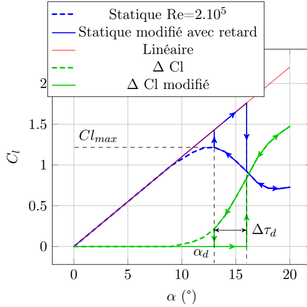
FIGURE 3.12 – Shématisation des données en portance avec retard au décrochage pendant un cycle montée-descente
