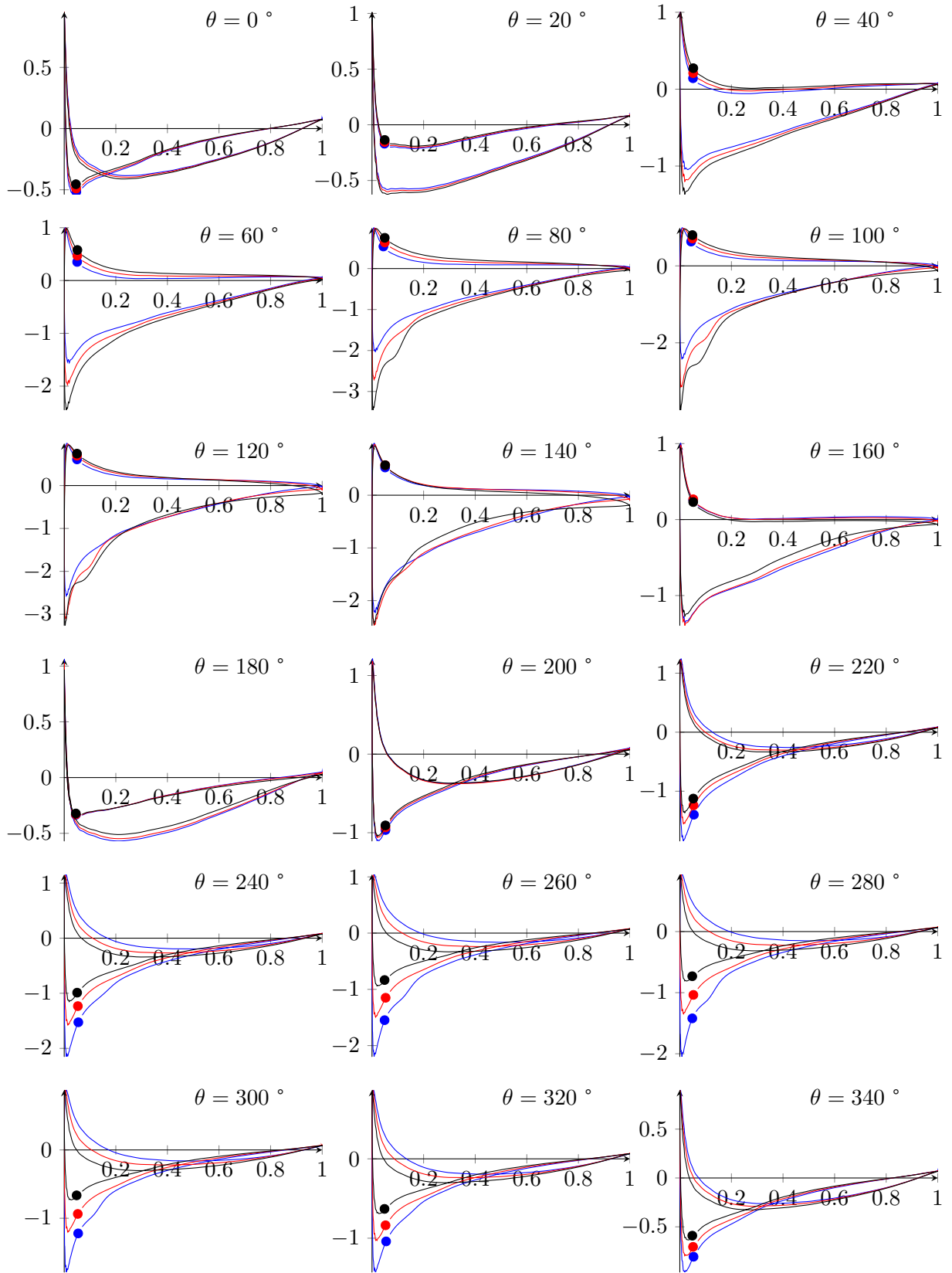
FIGURE C.8 – Coefficient de pression pour les cas f2a2 et f2a1
