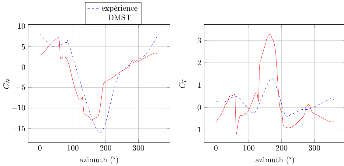
FIGURE 4.12 – Validation DMST pour le cas C : 2 pales, \lambda=2.5
