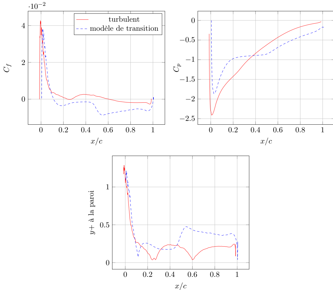
FIGURE 5.14 – Etude de modèle fluide : comparaison turbulent/transition, \theta = 140^\circ
