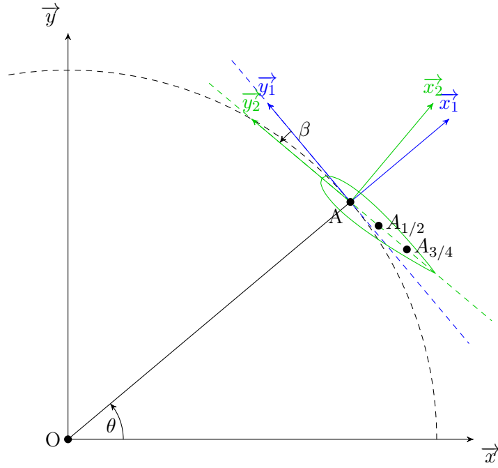
FIGURE 4.7 – Définition des différents points de calcul de l'incidence
