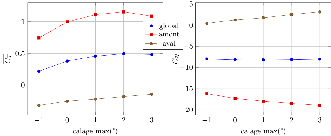
FIGURE 5.49 – Evolution de la moyenne des coefficients d’effort en fonction de l’amplitude de la loi de type f3 utilisée, cas D
