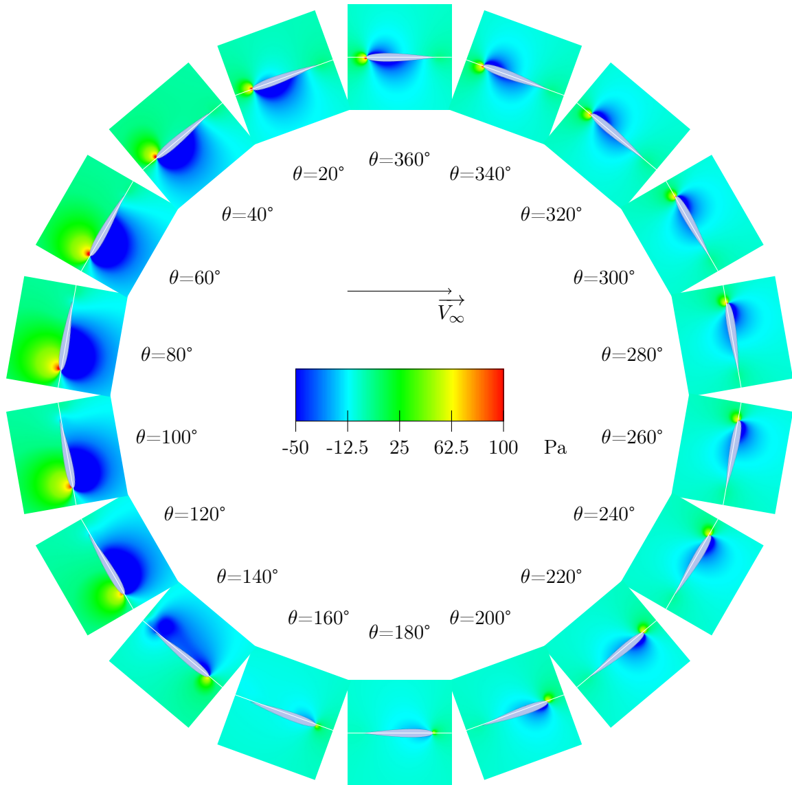
FIGURE 5.34 – champs de pression autour du foil dans le cas fl1a1, \lambda = 5
