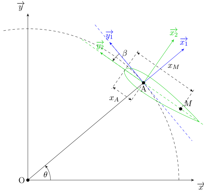
FIGURE 4.23 – Repérage de l'adaptation du modèle ONERA-EDLIN à la méthode DMST
