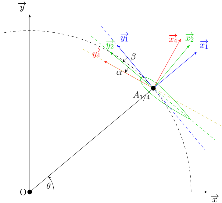
FIGURE 4.6 – Repères mis en place pour l'étude
