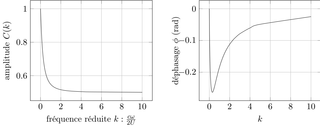
FIGURE 3.8 – Phase et amplitude de la fonction de déficit de portance utilisée dans le modèle de Theodorsen
