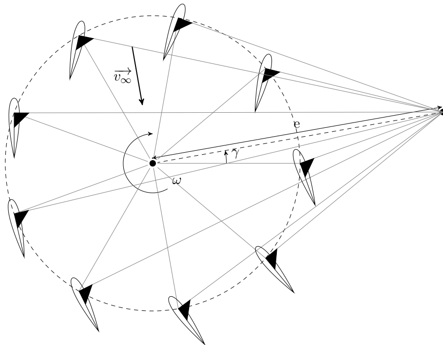
FIGURE 1.14 – Schéma du système Bose Lai avec \gamma = 10^\circ et e = 2r
