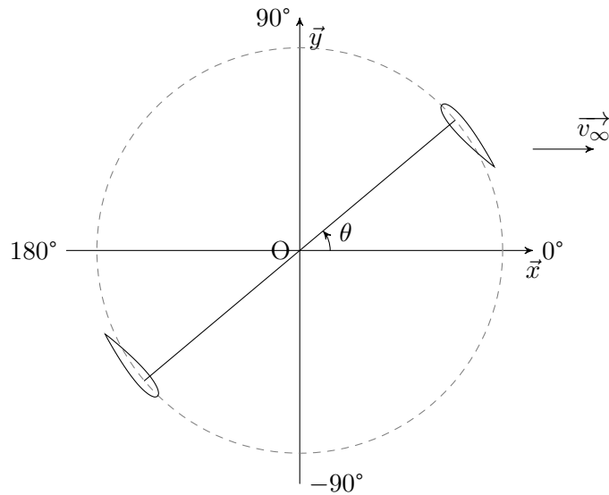
FIGURE 2.4 – Repère utilisé pour les calculs et simulations préliminaires
