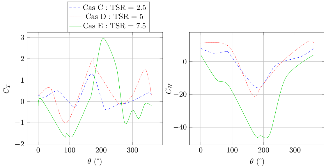
FIGURE 2.12 – Données expérimentales pour les cas C, D et E
