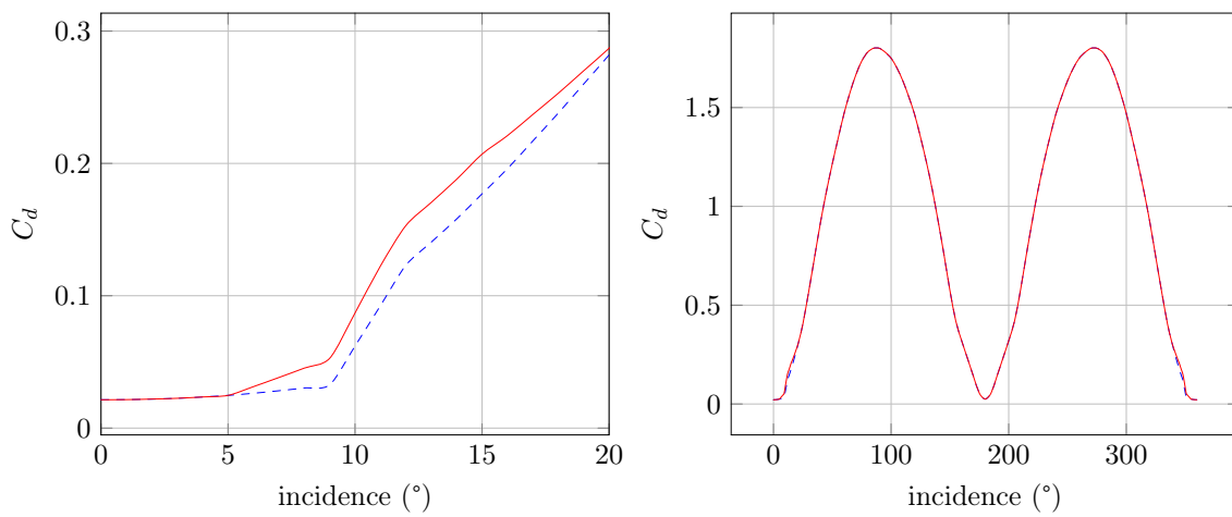
FIGURE 2.15 – Coefficients de traînée [Vittecoq and Laneville 1982, Sheldahl and Klimas 1981, Paraschivoiu 1998]
