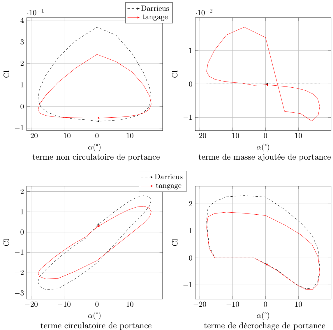
FIGURE 4.33 – Les différentes composantes de portance du modèle ONERA en tangage et Darrieus pour le cas C
