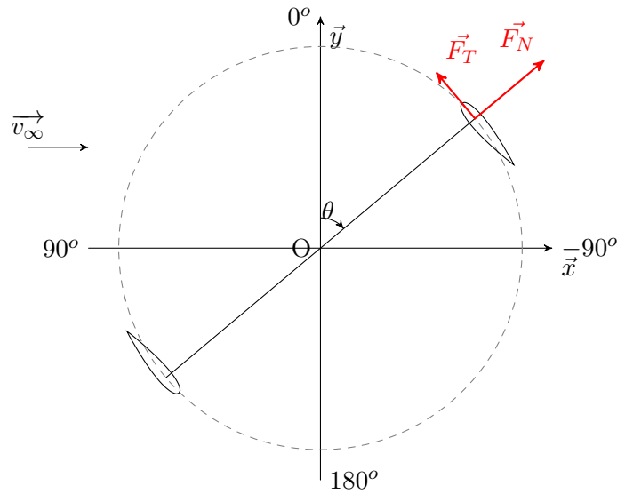
FIGURE 5.1 – Repère utilisé dans le modèle RANS
