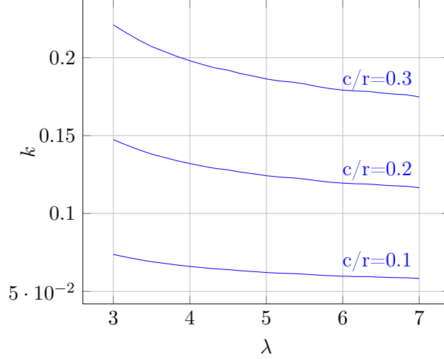
FIGURE 2.6 – Influence de \lambda et c/r sur la fréquence réduite d'une turbine Darrieus
