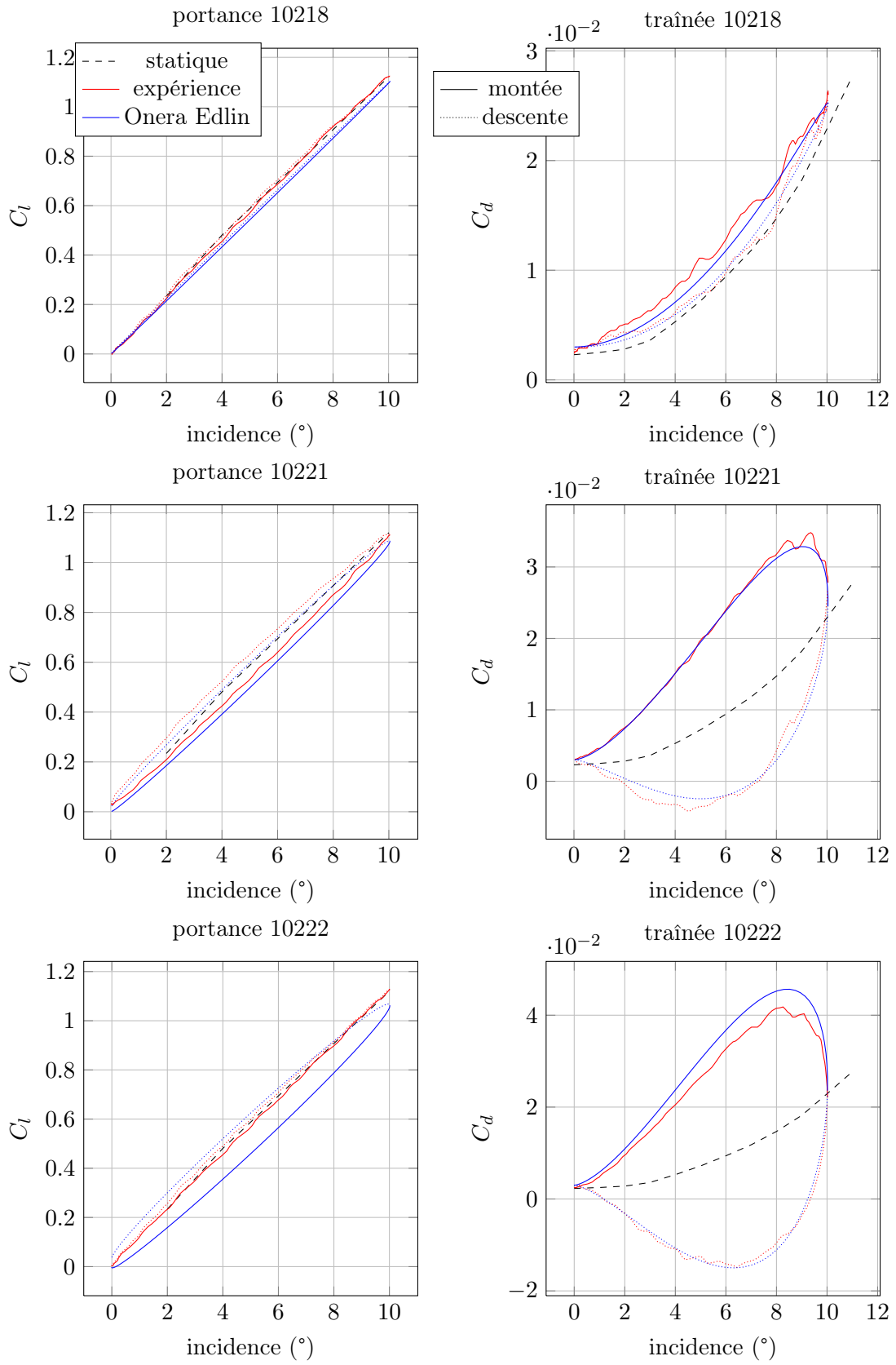
FIGURE 3.14 – Comparaison numérique expérience en écoulement accroché
