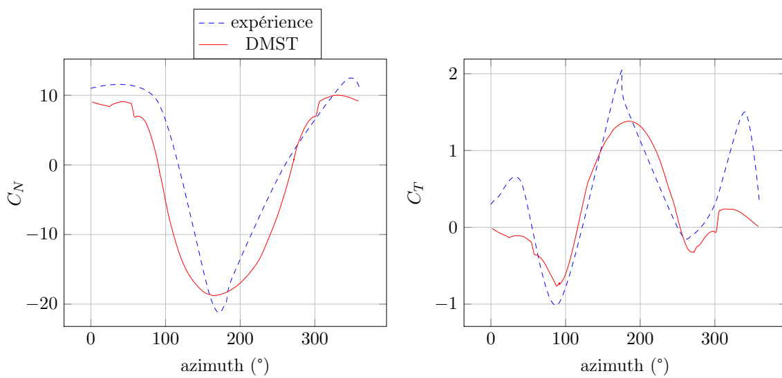
FIGURE 4.13 – Validation DMST pour le cas D : 2 pales, \lambda=5
