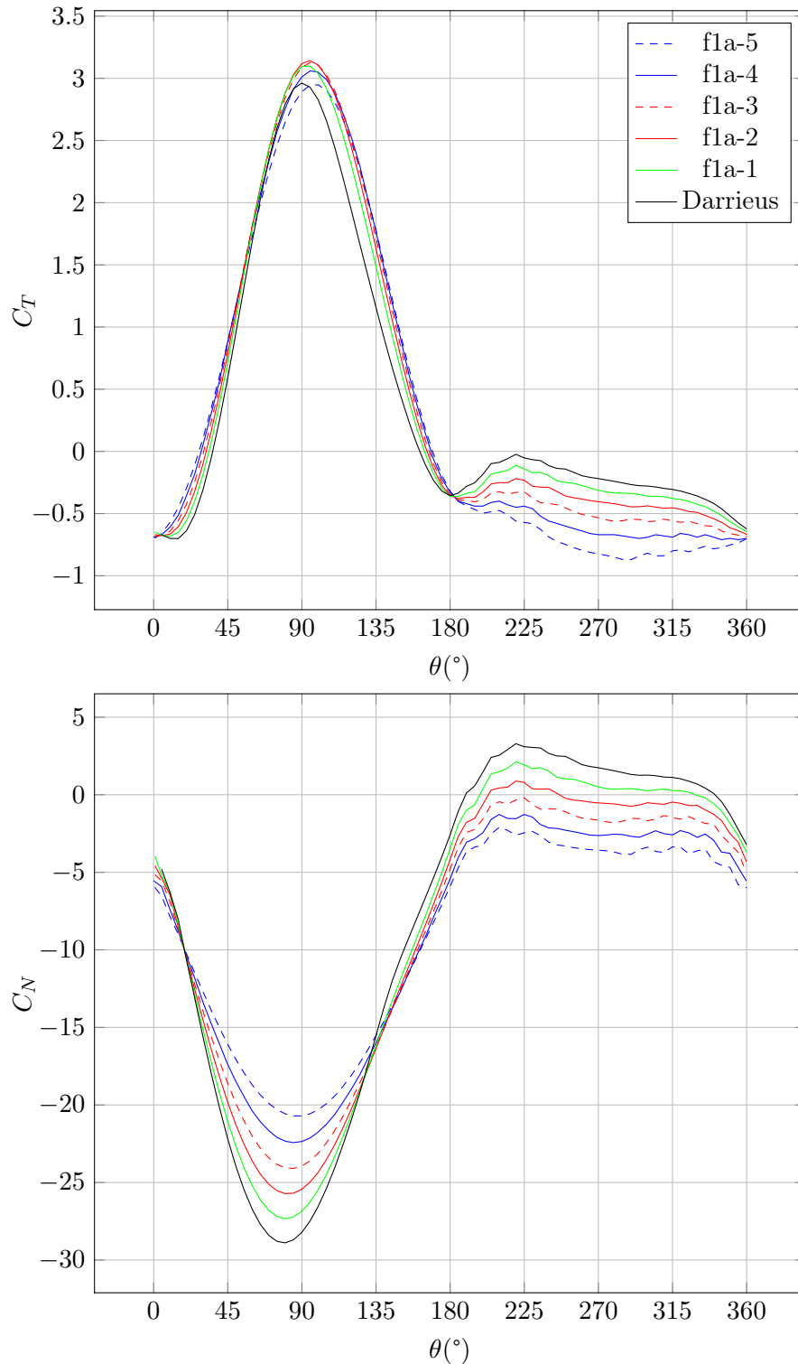
FIGURE 5.37 – Résultats d'effort pour des lois de pas de fréquence égale à la fréquence machine et d'amplitude négative, cas D, \lambda = 5
