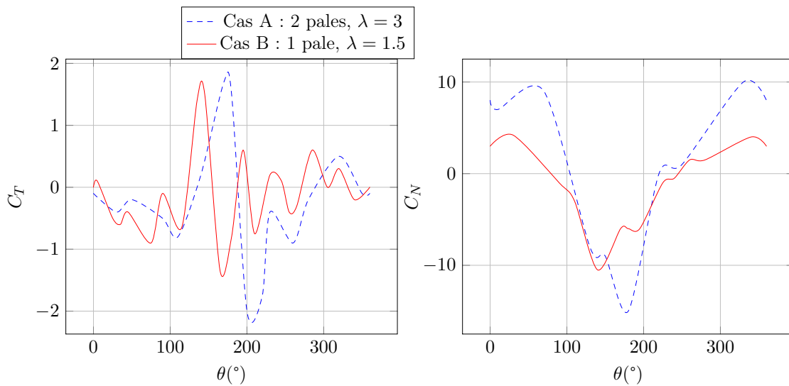
FIGURE 2.11 – Données expérimentales pour les cas A et B
