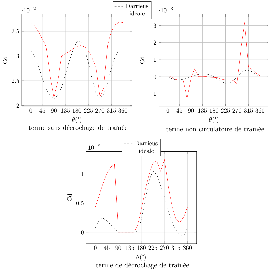
FIGURE 4.40 – Comparaison des différentes composantes de traînée du modèle ONERA
