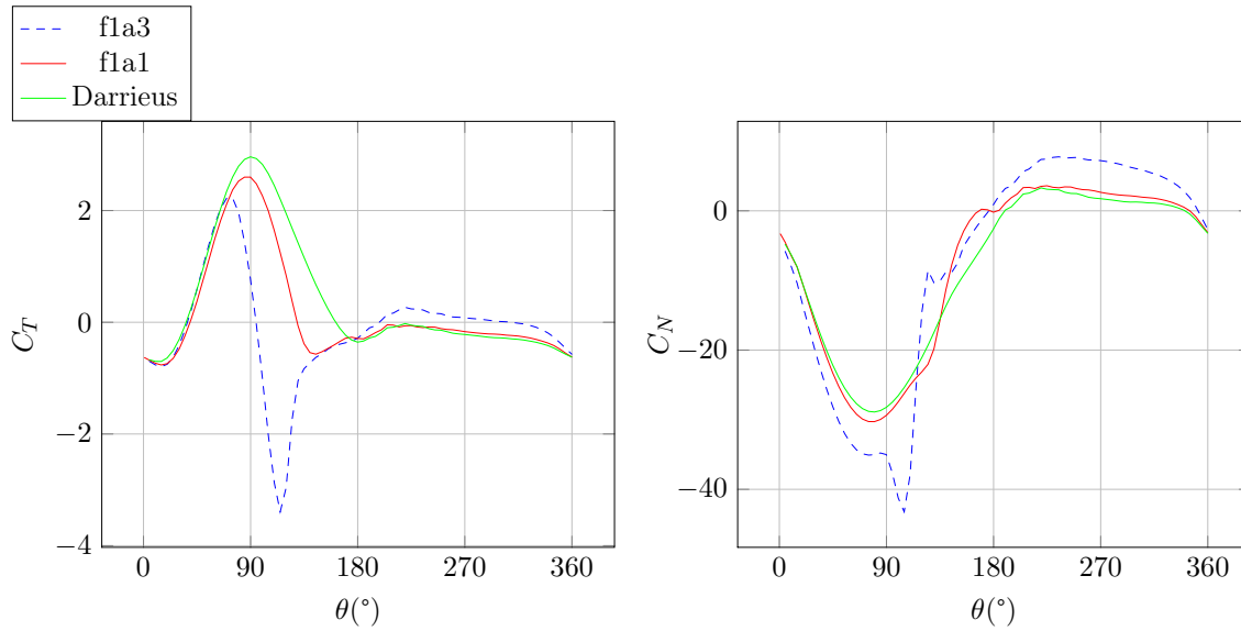
FIGURE 5.31 – Résultats d’effort pour des lois de pas de fréquence égale à la fréquence machine et d’amplitude positive, \lambda = 5
