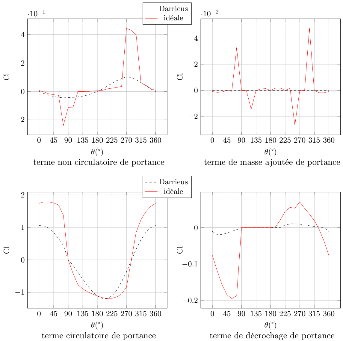
FIGURE 4.39 – Comparaison des différentes composantes de portance du modèle ONERA
