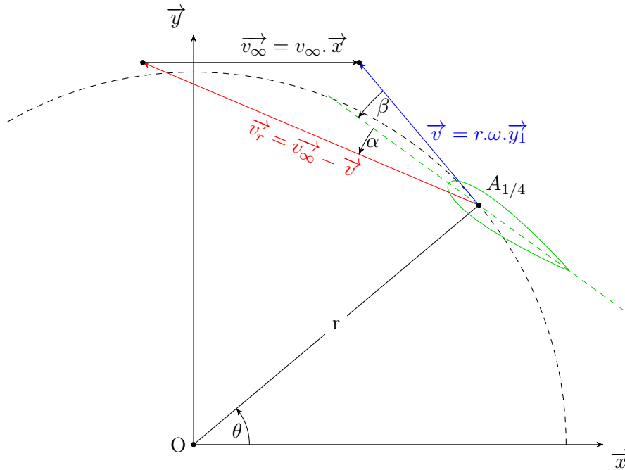
FIGURE 4.5 – Pale d’une turbine à axe transverse
