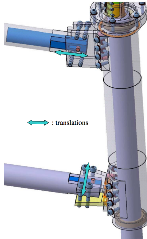
FIGURE D.3 – Réglage de verticalité des pales sur le système de variation de solidité
