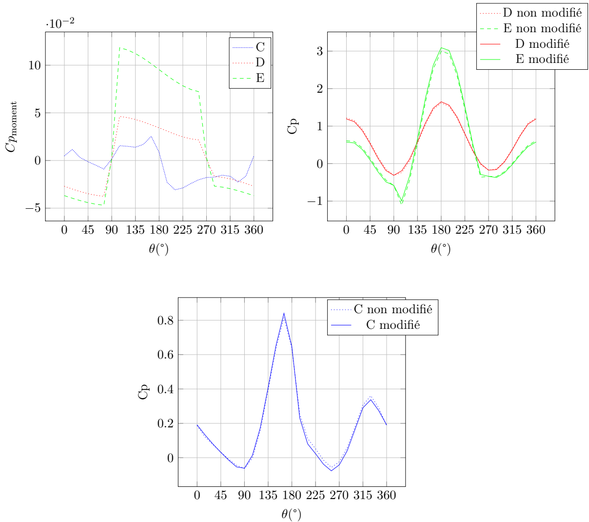
FIGURE 4.35 – Influence du moment sur les performance pour les cas C, D et E
