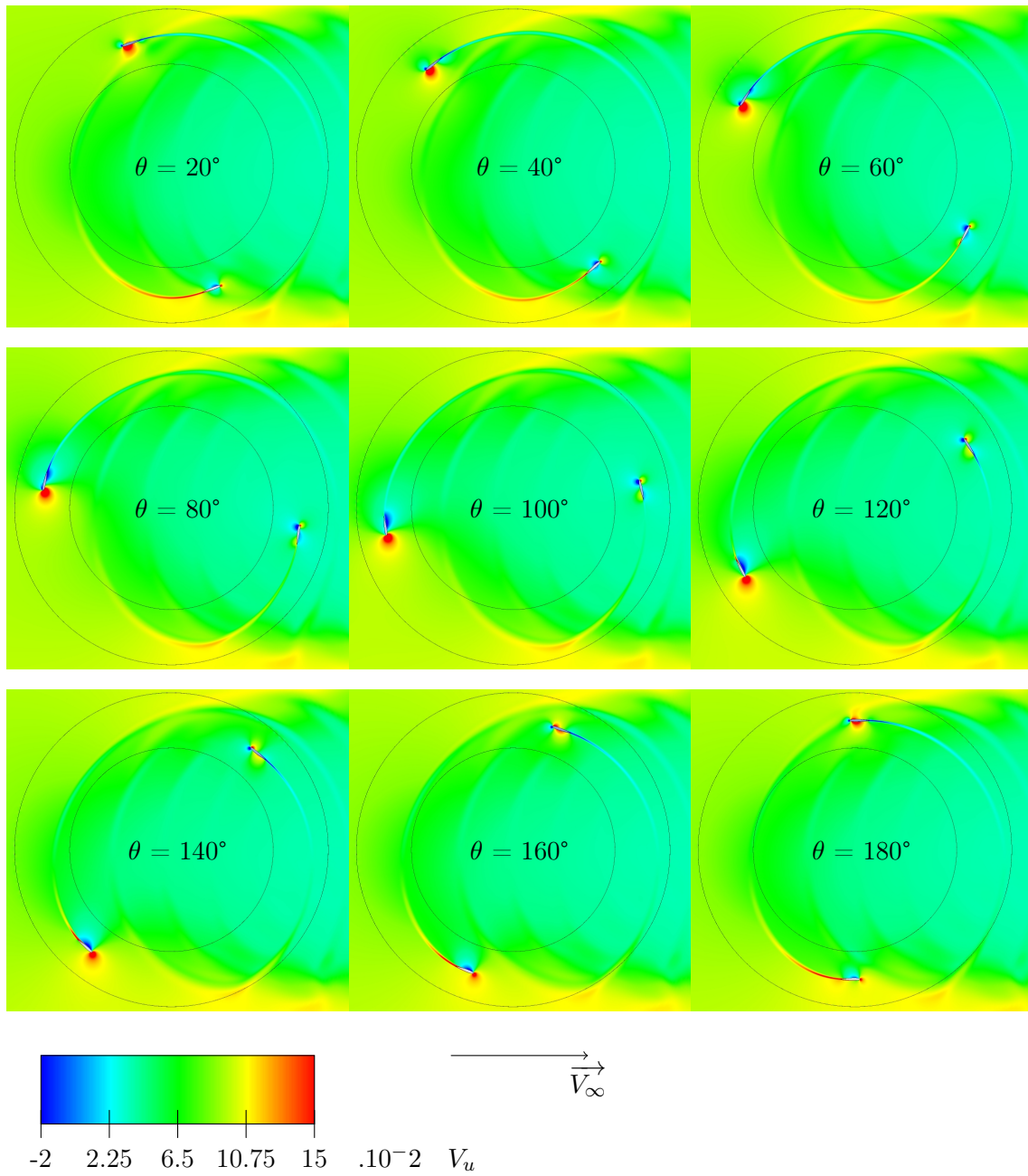
FIGURE 5.44 – Vitesse du fluide selon l'axe x pour le cas flamins2, \lambda = 5
