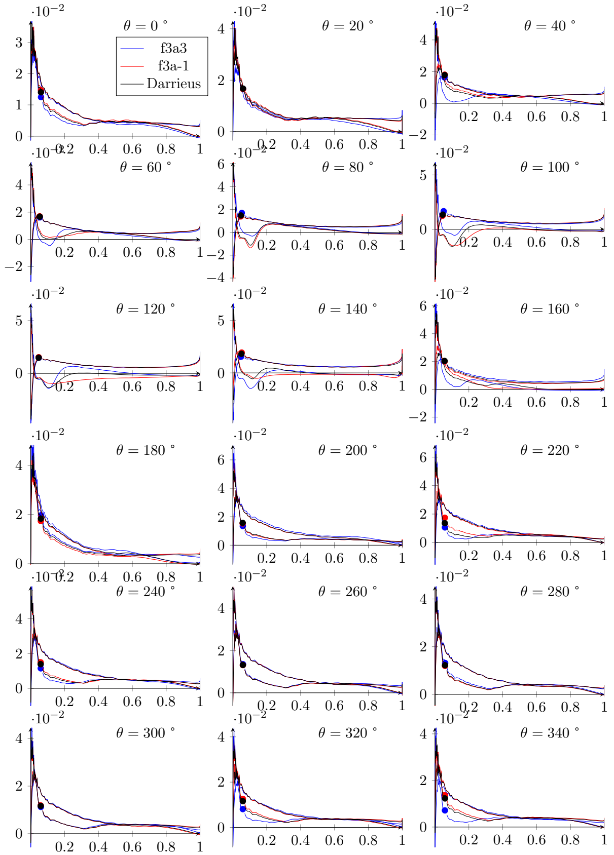
FIGURE C.5 – Coefficient de frottement à la paroi pour les cas f3a3 et f3-1
