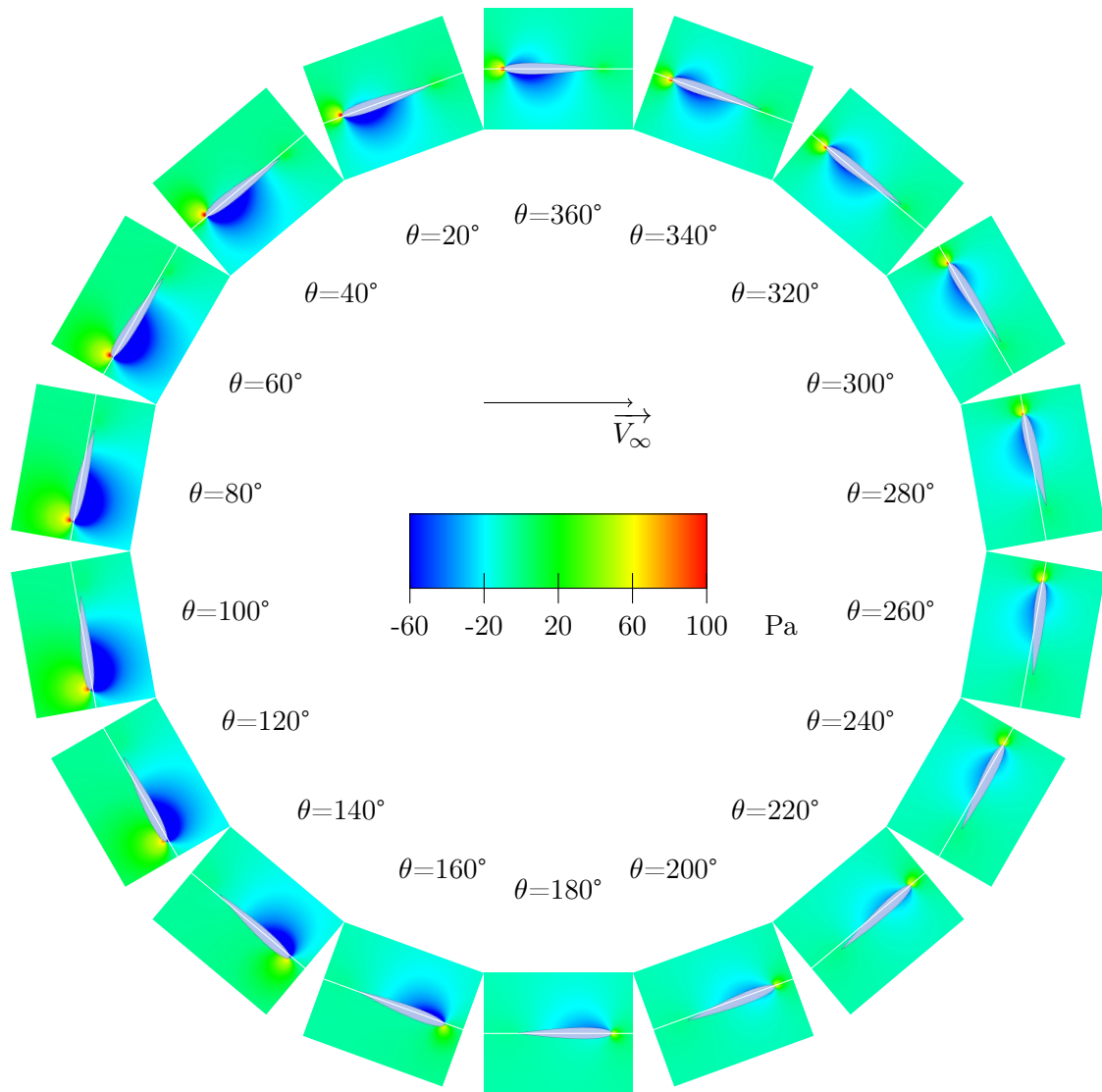
FIGURE 5.43 – champs de pression autour du foil dans le cas flamoin4, \lambda = 5
