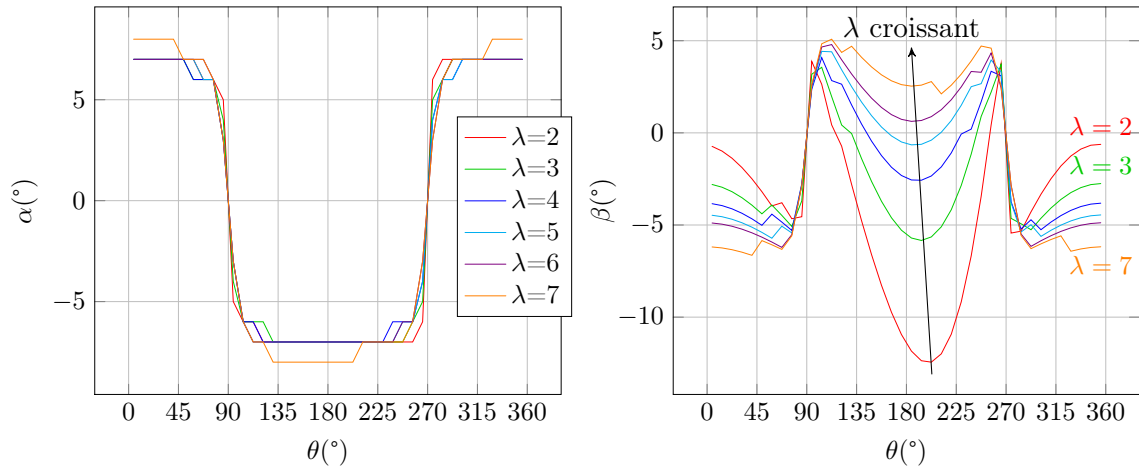
FIGURE 4.17 – Incidence et calage donnant les performances idéales d'après le modèle DMST à Reynolds faible
