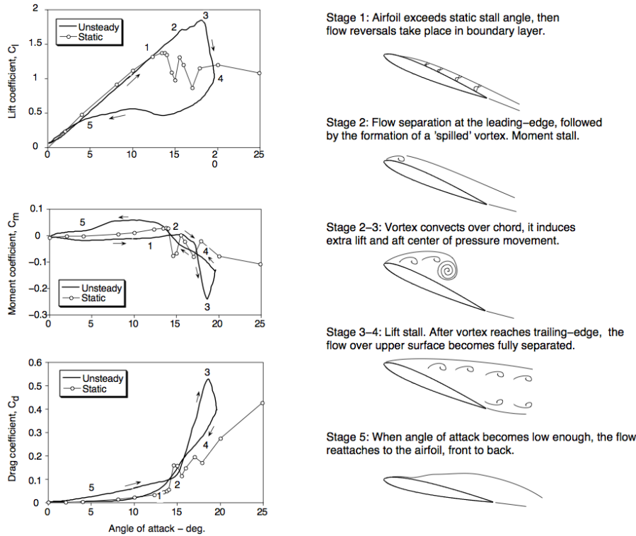
FIGURE 3.3 – Evolution typique du phénomène de décrochage dynamique. Extrait de [Leishman 2002]
