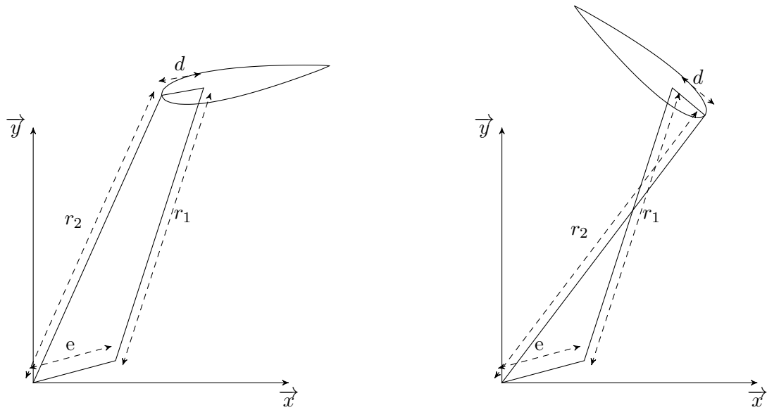
FIGURE A.2 – Les deux positions cinématiques possibles du système Pinson pour un ensemble de paramètres fixés.
