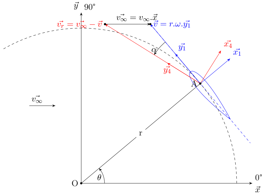
FIGURE 2.13 – Repère du modèle statique
