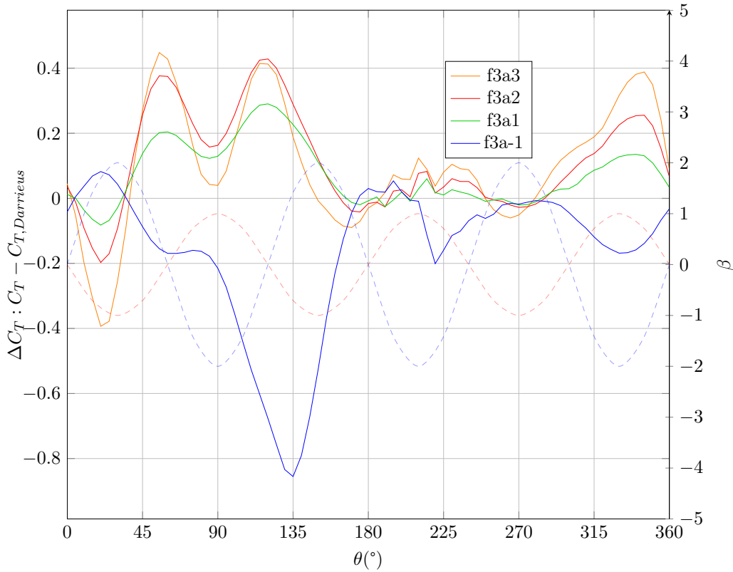
FIGURE 5.48 – Différence entre loi de pas variable et Darrieus pour le coefficient d’effort tangentiel, cas D, \lambda = 5
