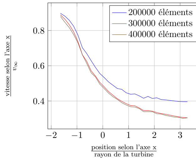
FIGURE 5.4 – Ecart de prédiction de sillage moyen en fonction du maillage
