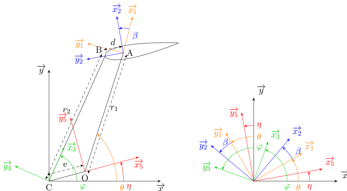
FIGURE A.1 – Repérage du système Pinson
