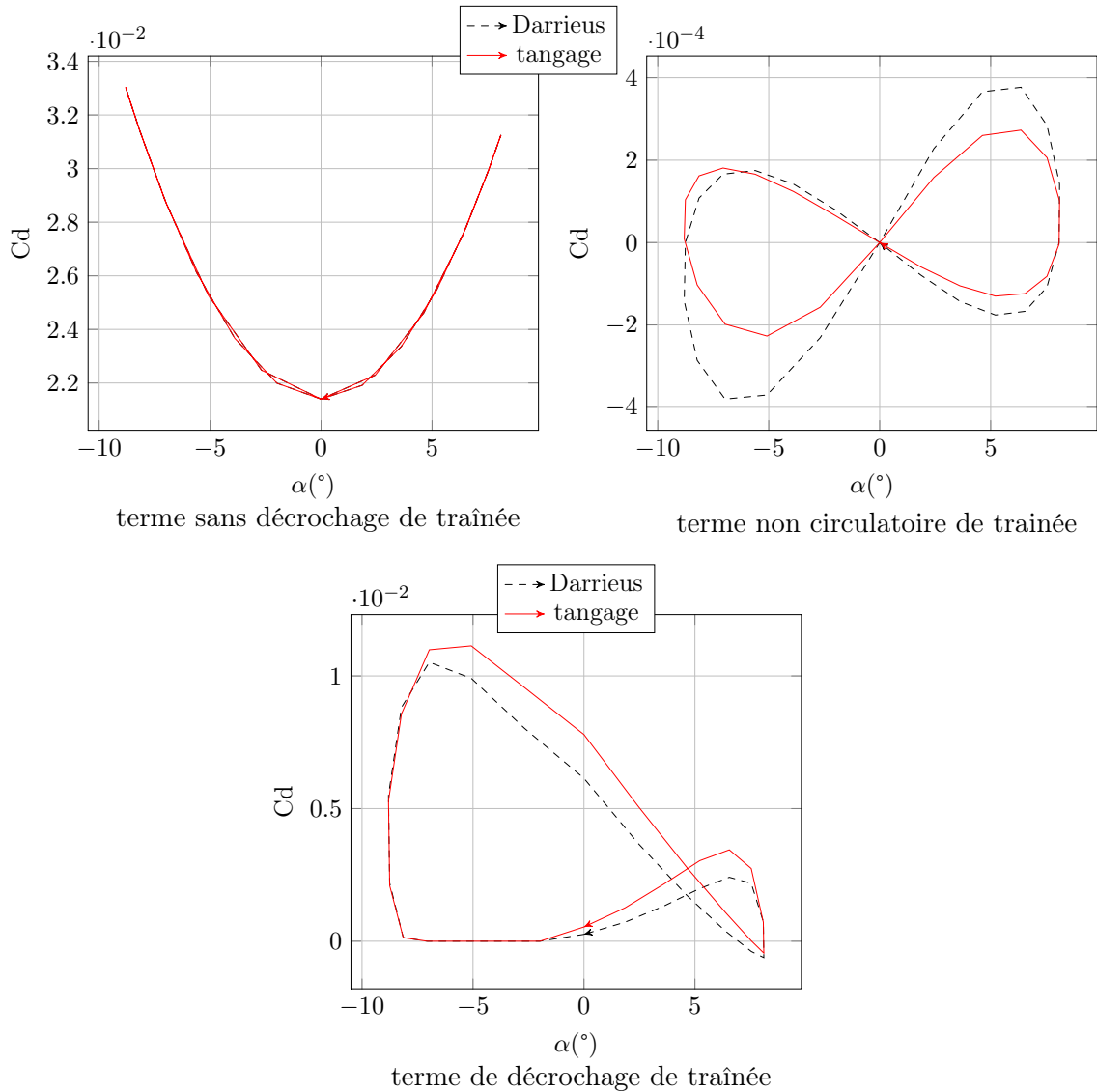
FIGURE 4.31 – Les différentes composantes de traînée du modèle ONERA en tangage et Darrieus pour le cas D
