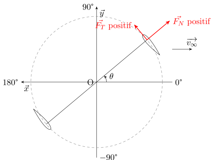
FIGURE 2.10 – Repère utilisé et orientation des efforts pour les cas expérimentaux
