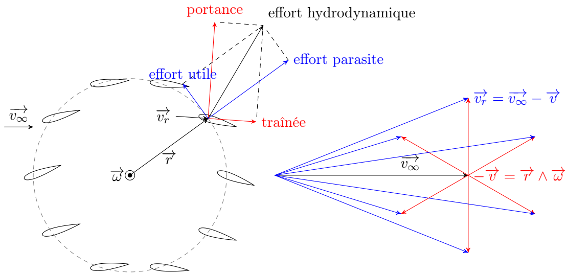
FIGURE 1.11 – Représentation des rotors dont \lambda < 1 ( \lambda \sim 0,7 ). L'échelle n'est pas respectée
