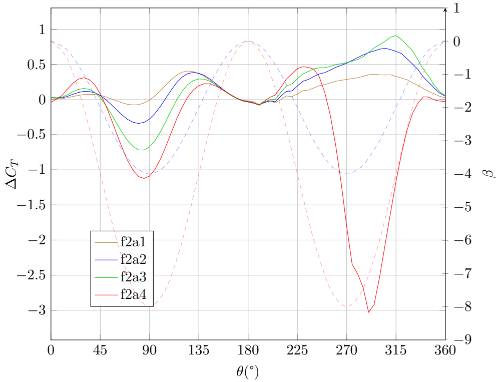
FIGURE 5.59 – Différence entre loi de pas f2 et Darrieus pour le coefficient d’effort tangentiel, \lambda = 5
