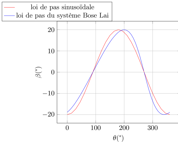
FIGURE 1.15 – Evolution de l'incidence du système Bose-Lai en fonction de la position azimutale pour une incidence maximal de 20^\circ
