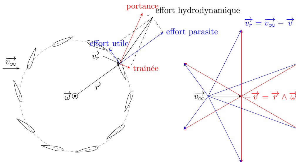
FIGURE 1.18 – Cinématique d'un rotor pour lequel \lambda > 1 ( \lambda \sim 3 )
