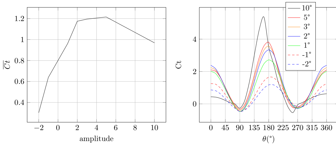
FIGURE 4.41 – Simulation de lois sinusoïdales de fréquence relative unitaire par le modèle ONERA-EDLIN
