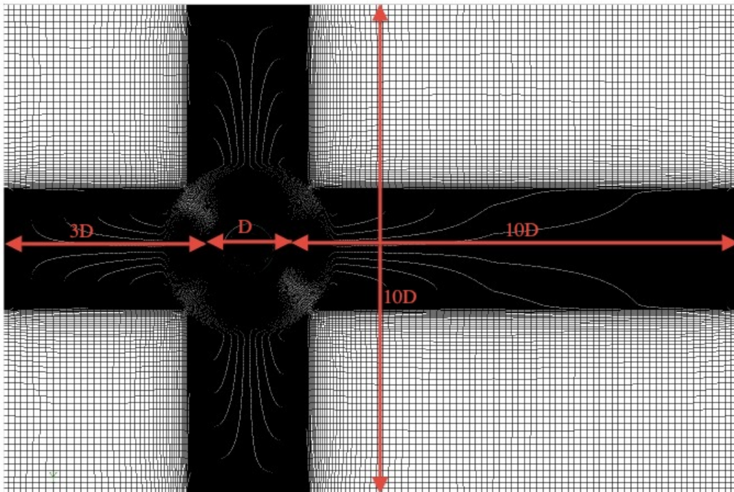
FIGURE 5.2 – Vue globale du maillage utilisé
