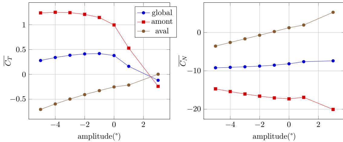
FIGURE 5.38 – Evolution de la moyenne des coefficients d'effort en fonction de l'amplitude, cas D, \lambda = 5
