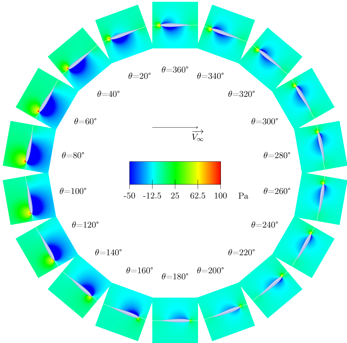
FIGURE 5.42 – champs de pression autour du foil dans le cas flamoin2, \lambda = 5
