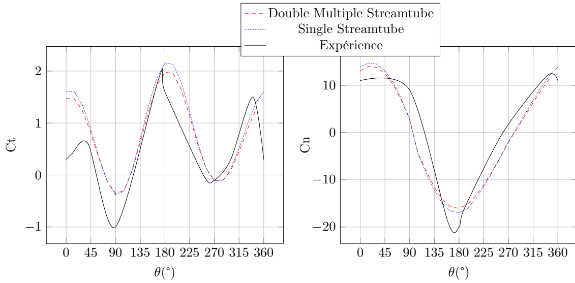
FIGURE 4.24 – Comparaison entre les différentes approches de simulation de ralentissement de fluide pour le modèle ONERA-EDLIN
