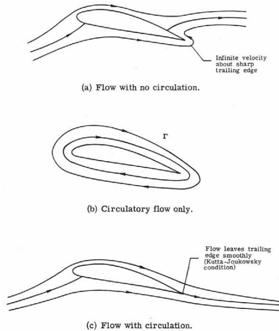
FIGURE 3.1 – Décomposition de l'écoulement autour d'un profil en terme circulaire et non circulaire
