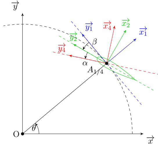
FIGURE 2.7 – Définition de l'angle de calage \beta
