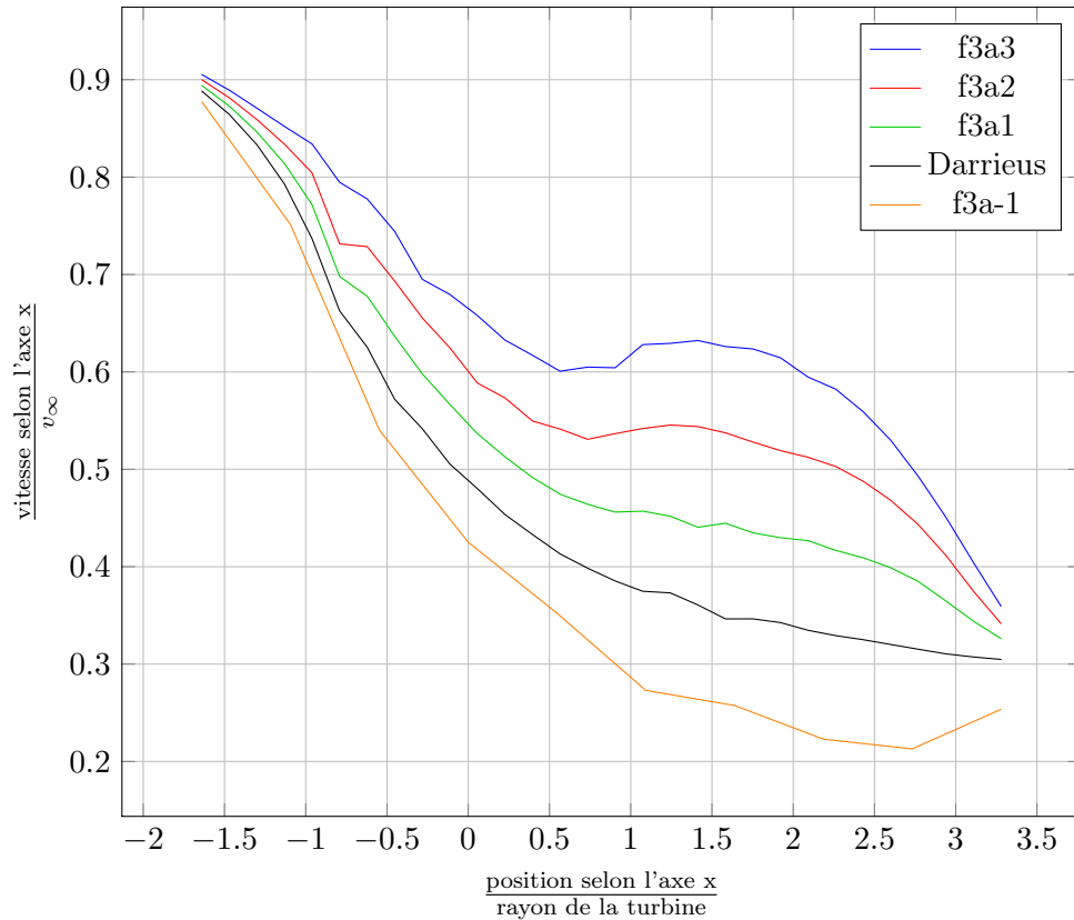
FIGURE 5.50 – Ralentissement du fluide pour les cas f3a-1, f3a1, f3a2 et f3a3 à l’ordonnée nulle, cas D, \lambda = 5
