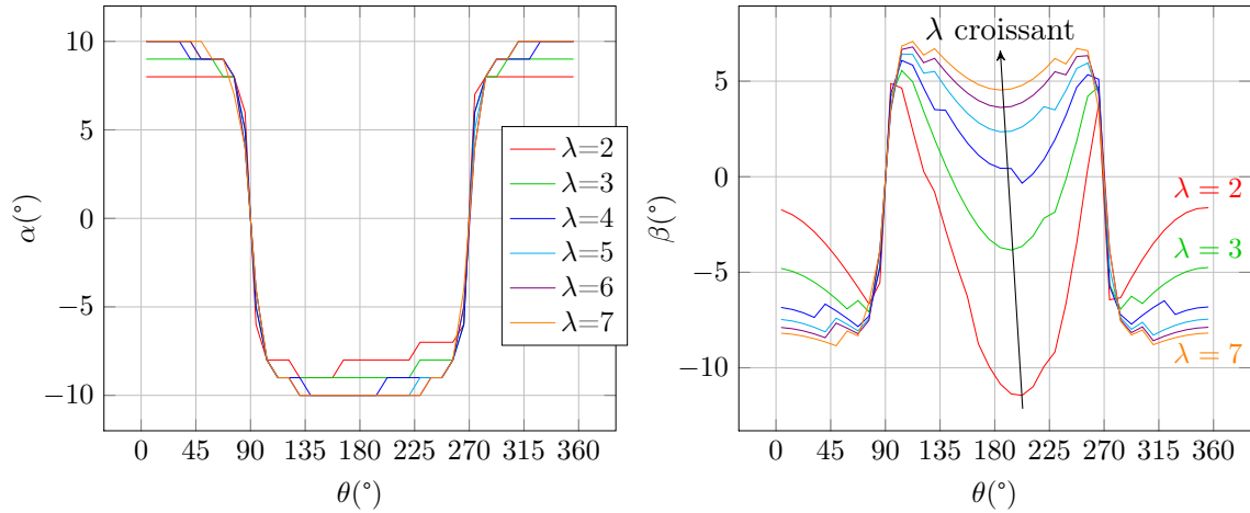
FIGURE 4.16 – Incidence et calage donnant les performances idéales d'après le modèle DMST à Reynolds élevé
