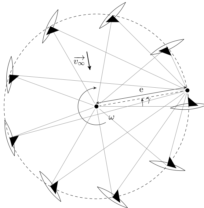
FIGURE 1.16 – Schéma du système Kirsten-Boeing avec \gamma = 10^\circ
