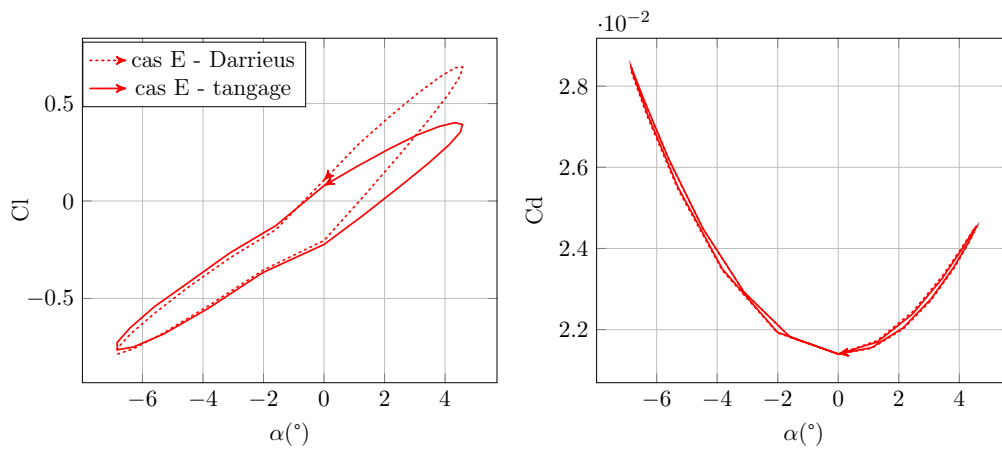
FIGURE 4.30 – Comparaison tangage simple/Darrieus pour le cas E
