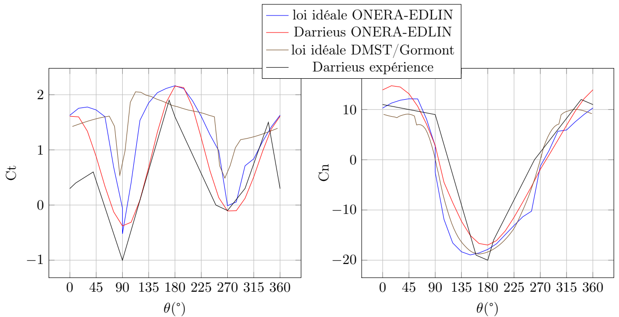
FIGURE 4.37 – loi idéale appliquée au cas D
