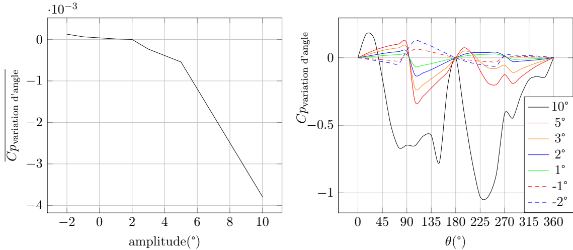
FIGURE 4.42 – Influence du moment hydrodynamique sur les performances pour des lois sinusoïdales de fréquence relative unitaire par le modèle ONERA-EDLIN
