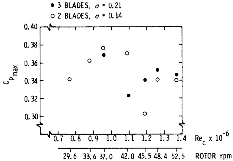
FIGURE 2.3 – Variation du coefficient de performance avec le nombre de Reynolds mesuré sur la turbine DOE/Sandia. Reproduit de [Worstell 1980]
