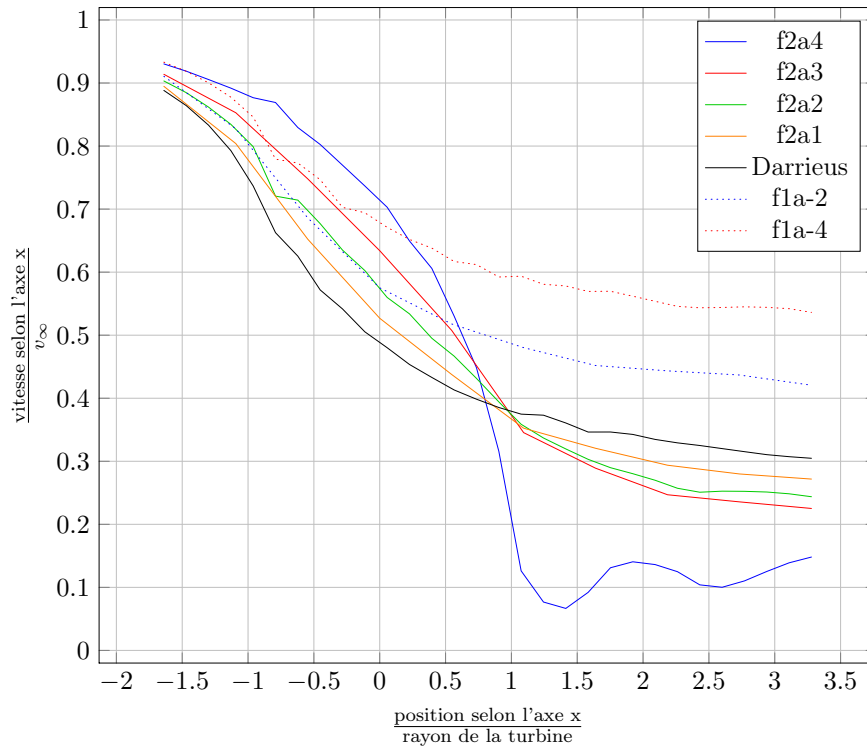
FIGURE 5.61 – Ralentissement du fluide pour les cas f2a1, f2a2, f2a3 et f2a4 à l’ordonnée nulle, \lambda = 5
