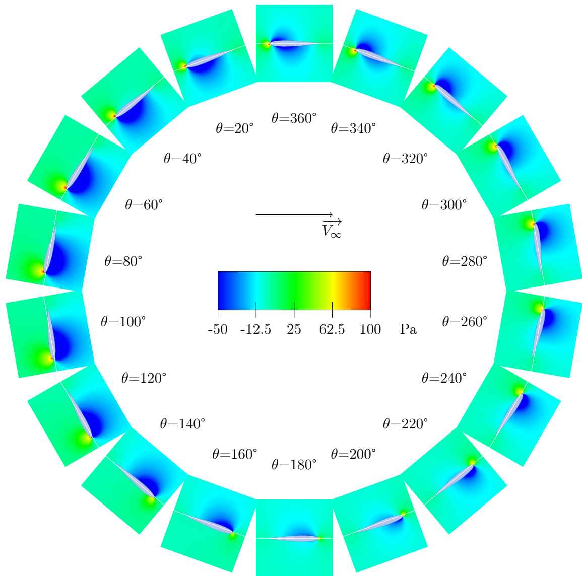
FIGURE 5.64 – champs de pression autour du foil dans le cas f2a2, \lambda = 5
