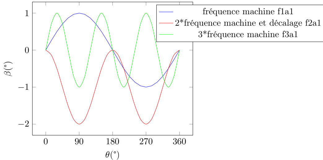
FIGURE 5.30 – Représentation des différentes fonctions de pas utilisées
