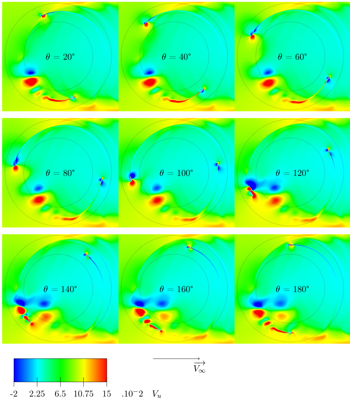
FIGURE 5.36 – Vitesse du fluide selon l'axe x pour le cas f1a3, \lambda = 5
