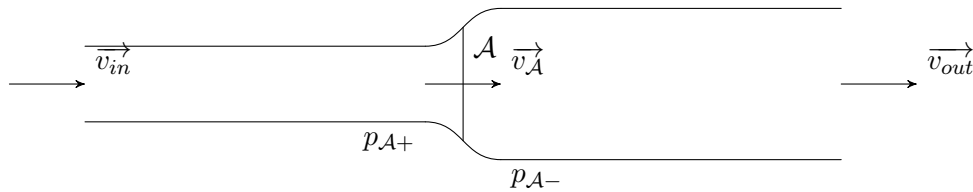
FIGURE 4.3 – Les différentes notations au sein d’un tube
