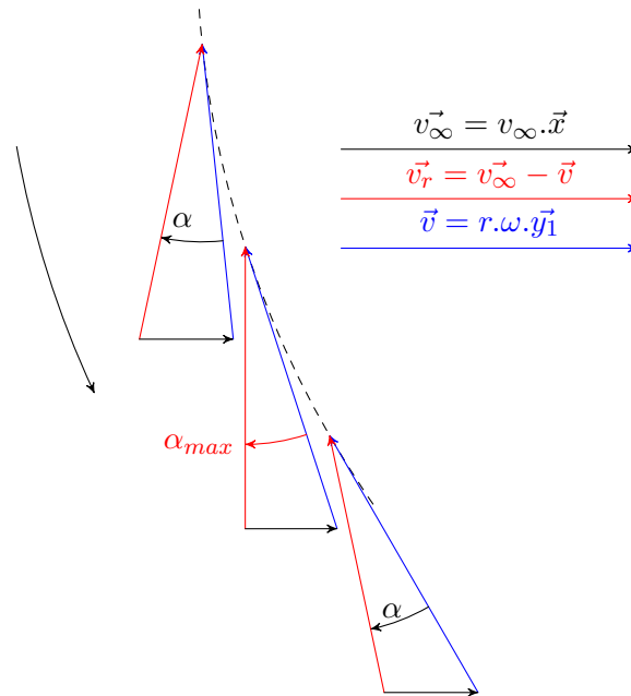
FIGURE 2.19 – Angle d'incidence géométrique à proximité de sa valeur maximale
