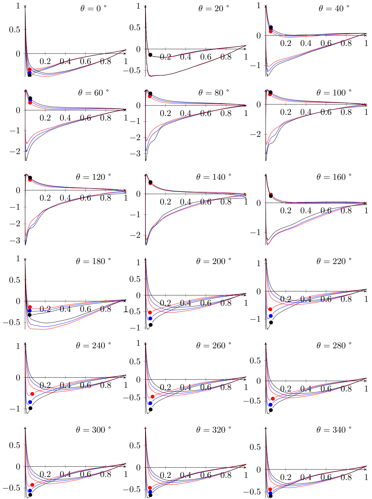
FIGURE C.4 – Coefficient de pression pour les cas f1a-2 et f1a-4
