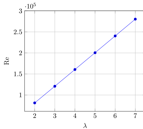
FIGURE 4.18 – Influence de \lambda sur le Reynolds dans le cas Re = 2 \cdot 10^5
