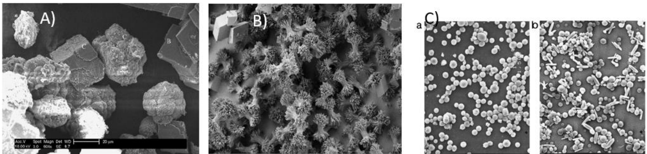
Figure 37. A) Transition solide-solide framboïdale de la vaterite en calcite (Nehrke, Van Cappellen et al. 2006). B) Recristallisation par sphérules de la vaterite en calcite (Beck and Andreassen 2010). C) Deux exemples de l'état métastable de l'aragonite en solution (Wang, Sondi et al. 1999)
