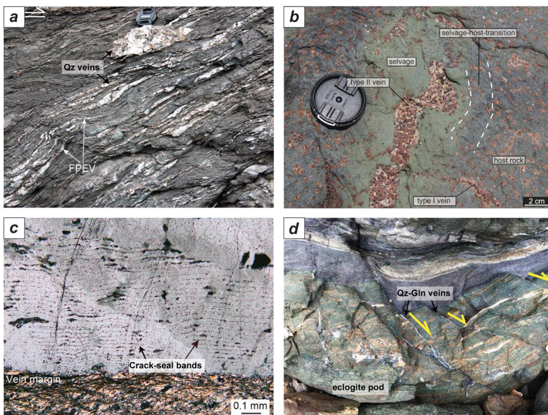
Figure 1.9 : Veines métamorphiques de roches HP-BT. A) Grandes quantités de veines de quartz dans les méta-sédiments du prisme de Shimanto (Japon). FPEV = foliation-parallel extension veins. Modifié d'après Ujiie et al. (2018). B) Veines à grenat-quartz-phengite dans un bloc éclogitique du Pouébo Eclogite Mélange (Nouvelle-Calédonie). D'après Taetz et al. (2018). C) Bandes d'inclusions dans une veine de type « crack-seal » du prisme de Shimanto (Japon). Ce type de veine se forme par des cycles successifs de fracturation, d'infiltration de fluide et de cristallisation. Chaque bande est interprétée comme un incrément de déplacement sur une surface de glissement. Modifié d'après Ujiie et al. (2018). D) Veines de cisaillement à quartz-glaucophane recoupant un boudin d'éclogite, Syros (Grèce). Modifié d'après Kotowski et Behr (2019).
