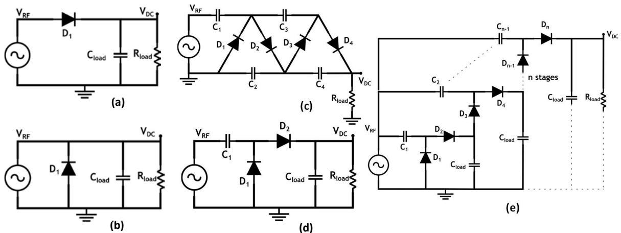
Figure 1.7. Rectifier topologies: (a) Series diode rectifier, (b) Shunt diode rectifier, (c) single stage Greinacher rectifier; (d) Cockcroft-Walton rectifier, (e) N-stage Dickson rectifier.
