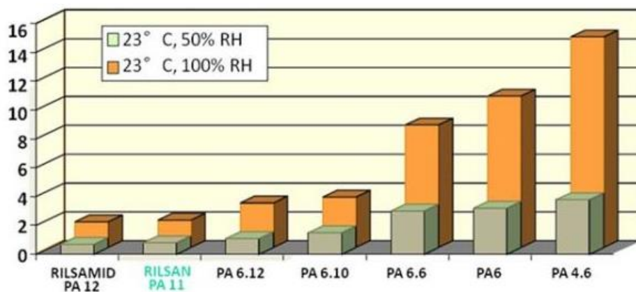
Figure 16 Histogramme comparatif de la résistance à l'humidité des PA
