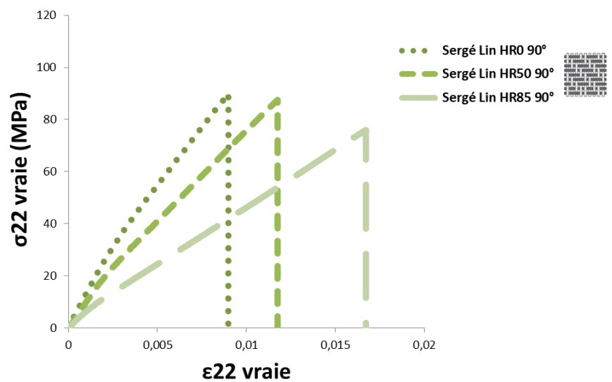
Figure 52 Essais de traction \sigma \text{ vraie} = f(\epsilon \text{ vraie}) dans le système de coordonnées locales pour le composites lin/PA11 pour 0°, 45° et 90° à HR0, HR50 et HR85 à T23°C
