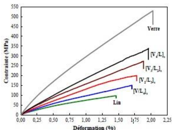
Figure 20 Courbe contrainte-déformation des matériaux composites non-hybrides et hybrides [2]
