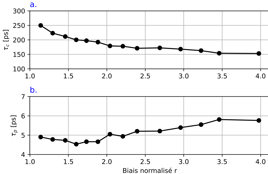
FIGURE 2.2 – Temps de vie caractéristiques du laser : a. temps de vie des porteurs, b. temps de vie des photons.
