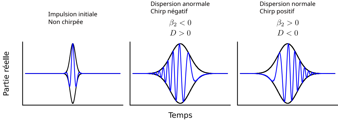
FIGURE 4.1 – Représentation d'impulsions en champs : état initial, après dispersion anormale, après dispersion normale.
