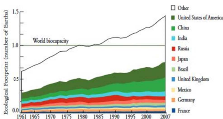
Figure 1: Évolution de l'empreinte écologique mondiale de 1961 à 2007 (Source : Global Footprint Network)
