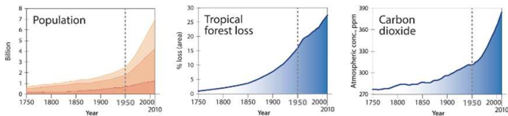
Figure 3: Tendances entre 1750 et 2010 pour trois indicateurs parmi d'autres (Source : Steffen et al, 2005)
