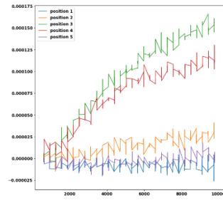
15% TMOS
