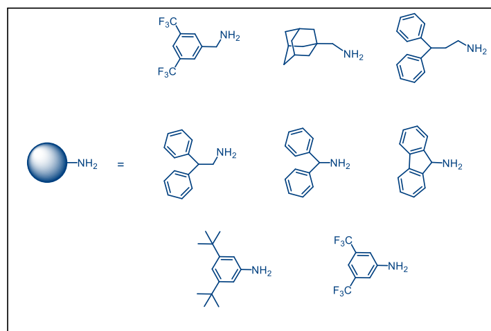
Figure 8. Préparation de [2]rotaxanes par réaction d'échanges de bouchons avec des amines primaires à partir d'un synthon activé à bouchons échangeables dinitrophénol.
