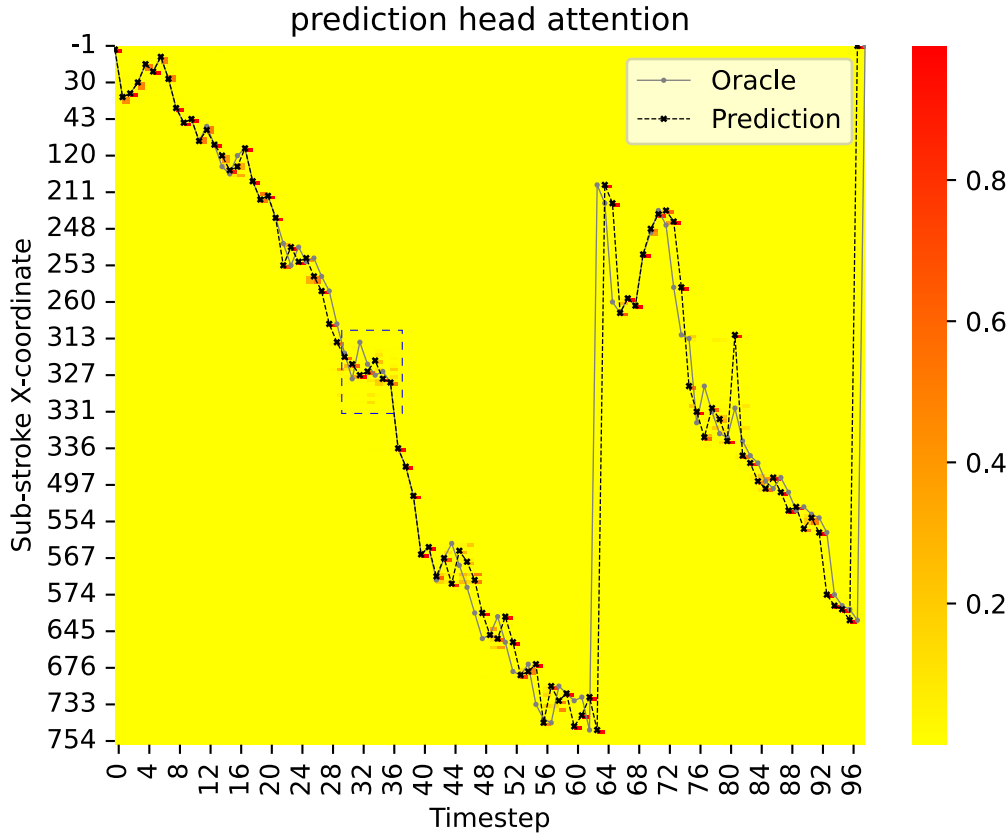
(a) Carte d'attention obtenue lors de l'inférence.
