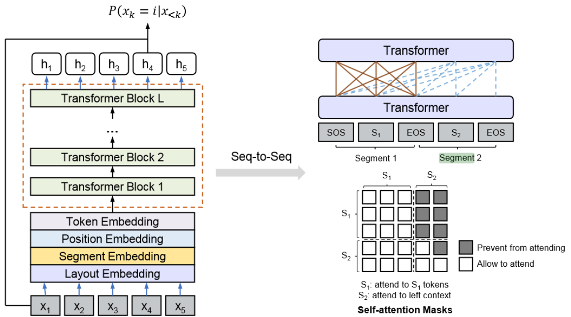
FIGURE 2.15 – Architecture du réseau LayoutReader. Le modèle prend en entrée la séquence de mots et leur mise en page (en segment) obtenu d'un système OCR. Le décodage s'effectue par segment de texte (ligne), ici segment 1 désigne la ligne source produite par un système d'OCR et segment 2 la ligne cible ré-ordonné. Les masques d'attentions habituellement sont employés pour assurer une auto-régressivité.
