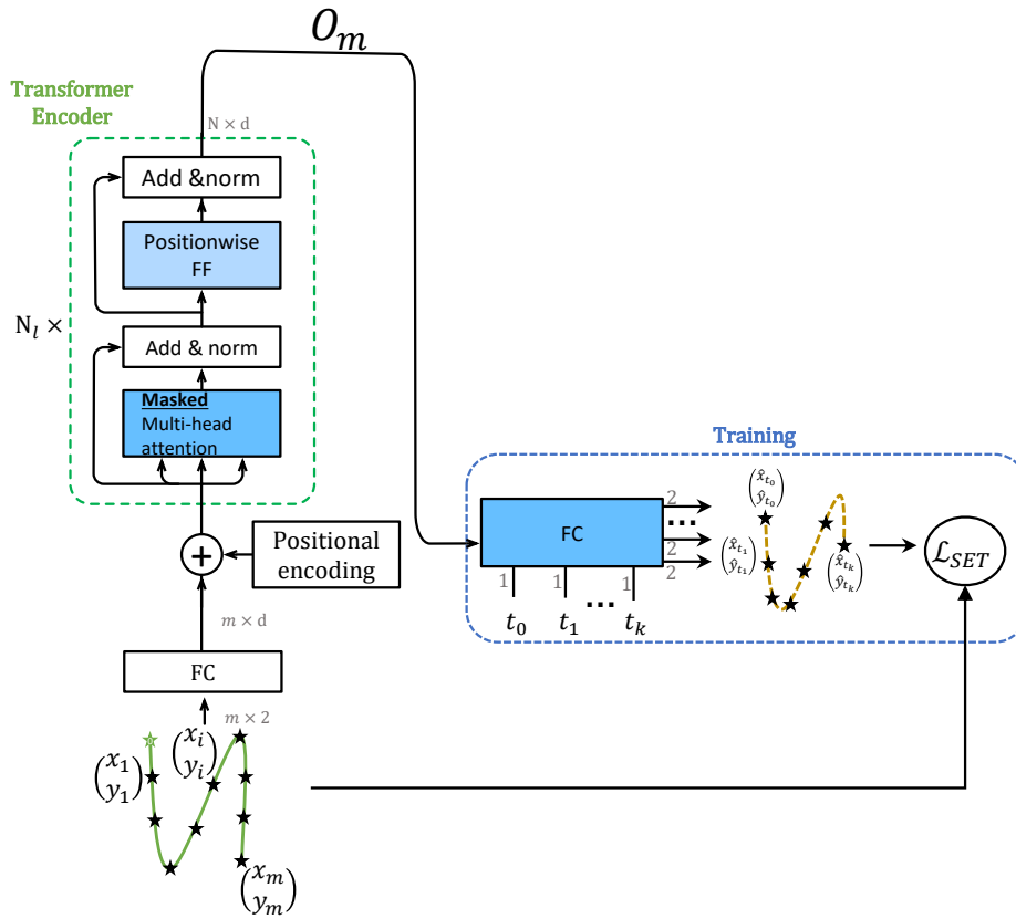
FIGURE 3.10 – Architecture du réseau SET.
