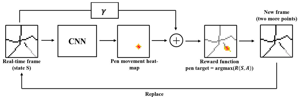
FIGURE 2.20 – Modèle CNN et algorithme d'inférence itérative.
