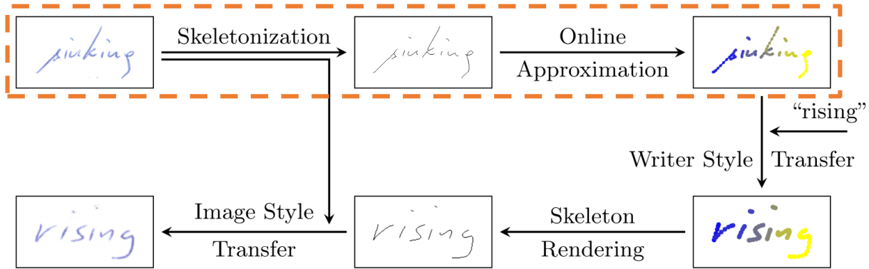
FIGURE 2.1 – Pipeline de Transfert de style d’écriture hors-ligne à hors-ligne (illustration de [May+20]). L’image est convertie d’abord en signal en-ligne (encadré en pointillé orange), puis le transfert de style est effectué dans le domaine en-ligne avant d’être rastériser en une image d’écriture hors-ligne.
