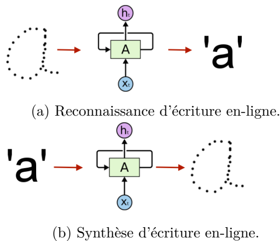
FIGURE 2.9 – Modèle LSTM pour la reconnaissance en-ligne et le problème inverse de synthèse d'écriture en-ligne. Illustration de Greydanus.
