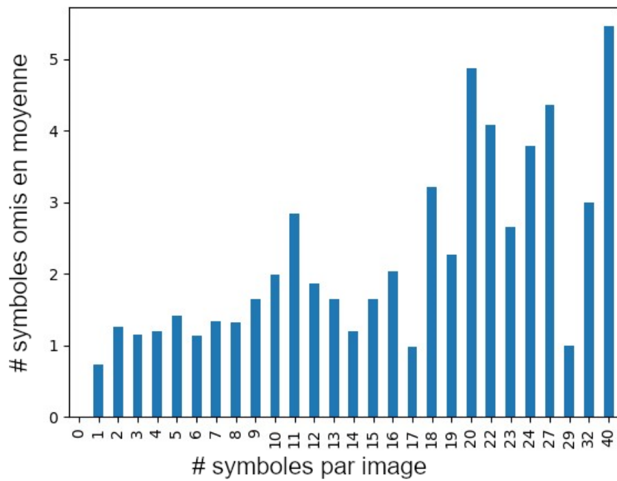
FIGURE 3.18 – Nombre moyen de symboles omis en moyenne en fonction du nombre de symboles par image des 142 expressions erronées mentionnées précédemment.
