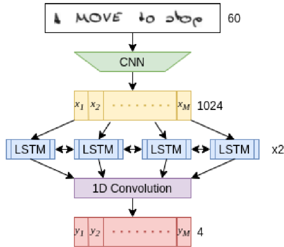
FIGURE 2.21 – Modèle CNN-BiLSTM
