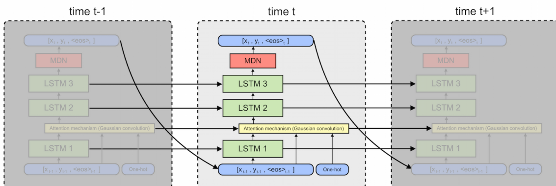
FIGURE 2.10 – Modèle LSTM de synthèses d'écriture en-ligne de [Gra14]. Illustration de Greydanus.
