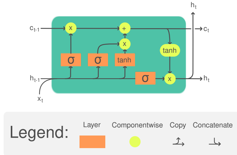
FIGURE 2.8 – Illustration des portes du LSTM. Source de l'image : Wikipédia.
