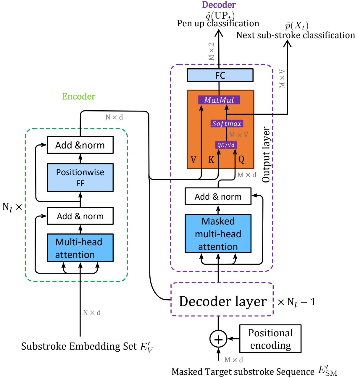
FIGURE 3.11 – Architecture du réseau SORT. La couche de sortie exprimée par l’expression 3.10 est ici représentée. Les dimensions des tenseurs en sortie des couches sont indiquées en gris. Illustration inspirée de [Zha+23].
