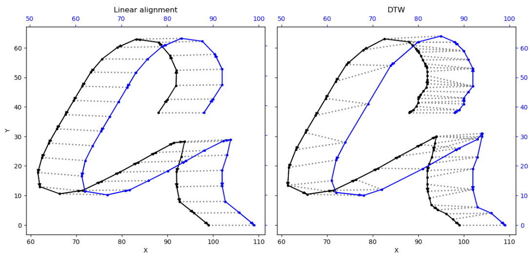
(b) À gauche, l’alignement linéaire RMSE qui nécessite un rééchantillonnage des deux signaux, et à droite, alignement par DTW.
