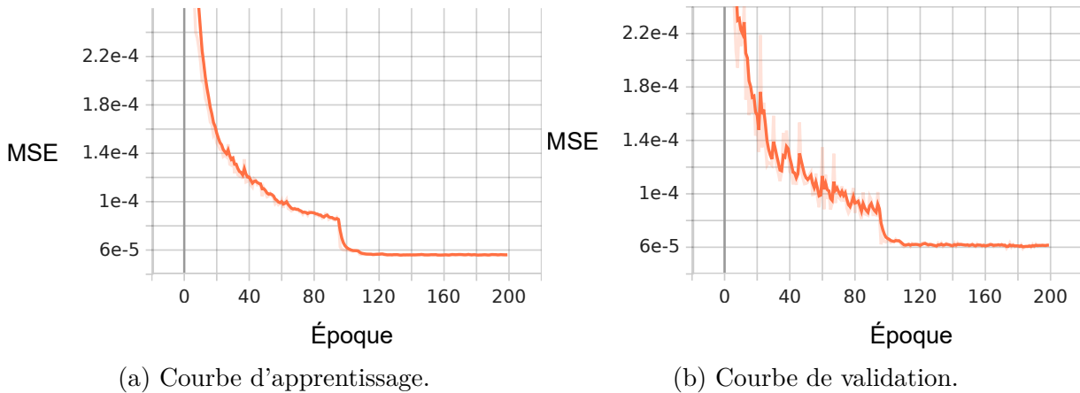
FIGURE 3.12 – Courbes d'apprentissages et de validation du modèle SET sur la base IRONOFF. On rappelle que la fonction de coût \mathcal{L}_{SET} employée ici est une MSE.
