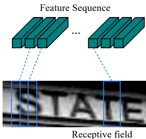
FIGURE 2.19 – Zone de l’image associée au champ récepteur d’un vecteur de la séquence de caractéristiques.
