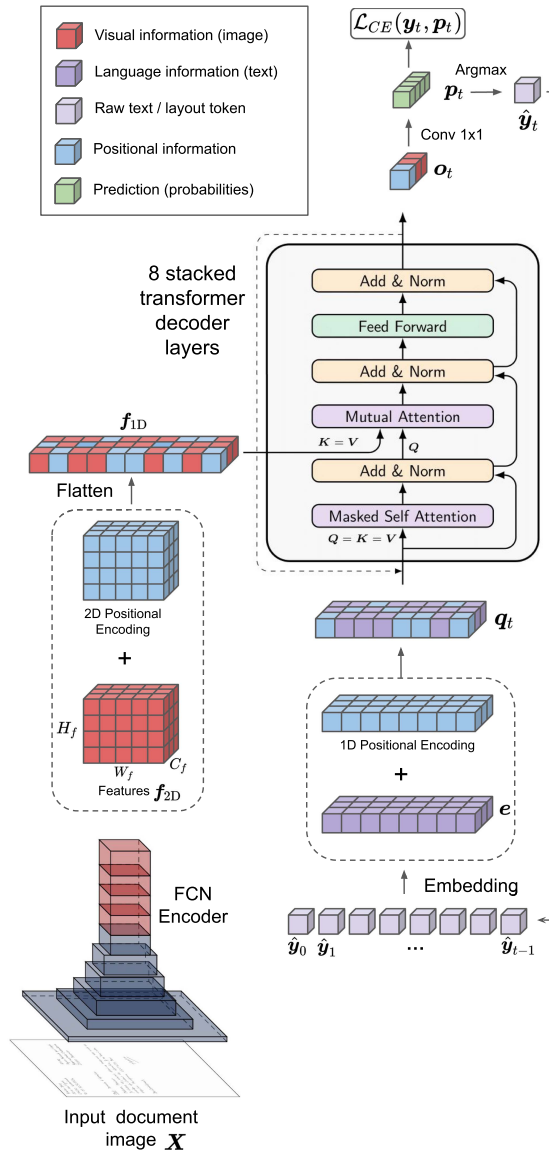
FIGURE 2.13 – Architecture CNN-Transformer pour la reconnaissance de texte manuscrit à l'échelle document. Illustration par [CCP23].
