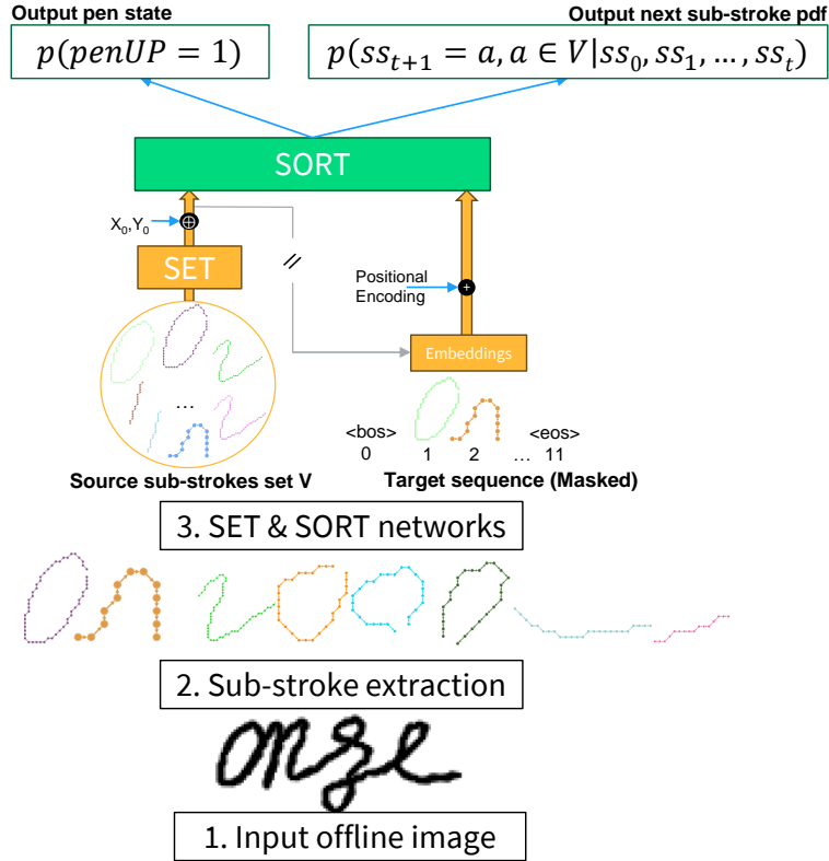
FIGURE 3.7 – Aperçu de l’approche proposée. Après l’extraction des sous-trait à partir du squelette du hors-ligne, le réseau SET permet d’obtenir un vecteur descripteur de sous-trait. Le réseau SORT utilise l’ensemble des vecteurs descripteurs V et l’historique pour prédire le prochain sous-trait ss_{t+1} et l’état du stylo.
