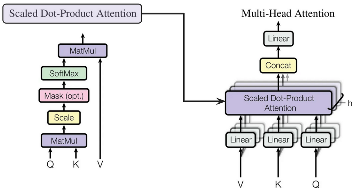
FIGURE 2.12 – (Gauche) Attention avec un produit scalaire normalisé. Un masque est appliqué aux scores d'attentions dans le décodeur pour garantir l'auto-régressivité. (Droite) Un module d'attention multitête consiste en un ensemble de têtes d'attention calculées indépendamment puis agrégées ensemble pour produire une sortie cachée. Illustration par [Vas+17].
