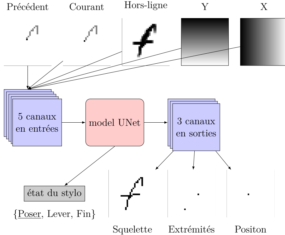
FIGURE 3.4 – Entrées et sorties de notre modèle CNN.
