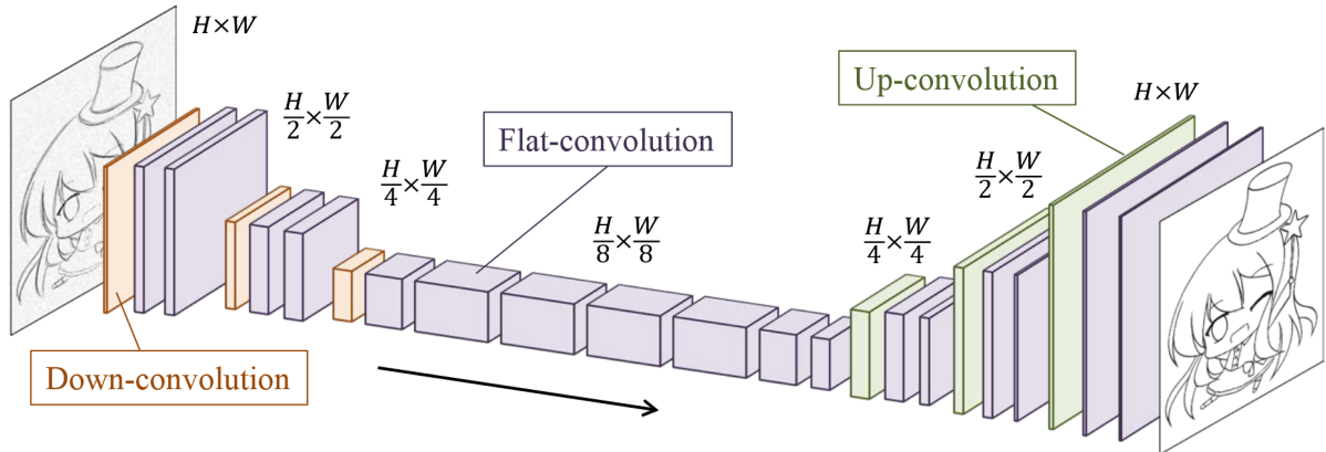
FIGURE 2.6 – Architecture FCNN encodeur-décodeur de [SS+16].
