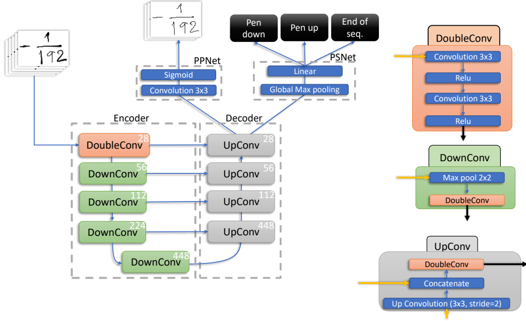
FIGURE 3.5 – Architecture du réseau. Le nombre de filtres utilisés dans chaque convolution est indiqué sur chaque bloc. L’encodeur et le décodeur sont partagés par PSNet et PPNet.
