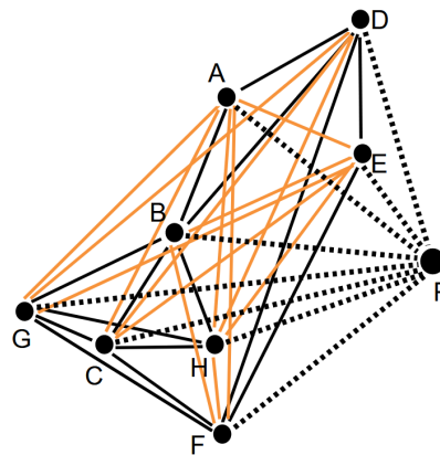
(b) Graphe complet G_K .
