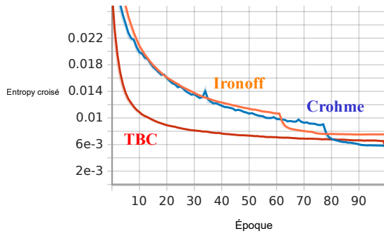
(a) Courbe d'apprentissage de l'ordonnement des sous-traits \mathcal{L}_{\Pi_t} .
