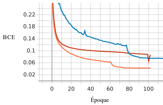
(c) Courbe d'apprentissage de la classification des levers de stylo \mathcal{L}_{UP_t} .
