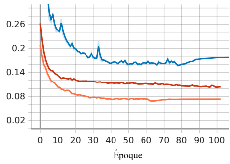
(d) Courbe de validation de la classification des levers de stylo \mathcal{L}_{UP_t} .
