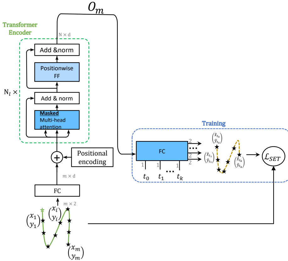
FIGURE 3.10 – Architecture du réseau SET.
