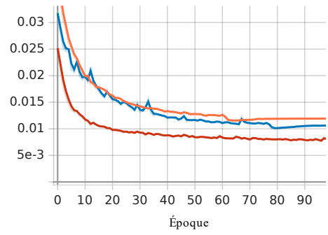
(b) Courbe de validation de l'ordonnement des sous-traits \mathcal{L}_{\Pi_t} .
