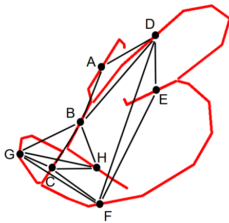
(a) Graphe adjoint G associé au squelette d'une lettre "B".
