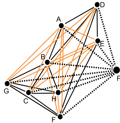
(b) Graphe complet G_K .
