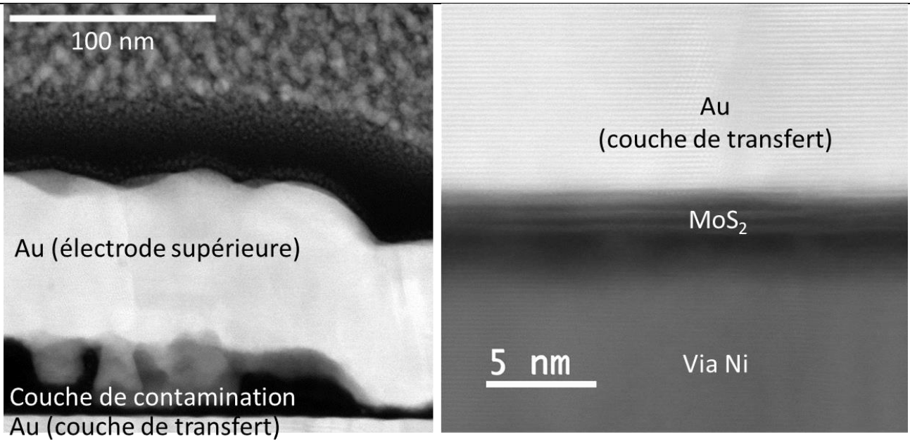
Figure III-20 : Observations TEM en coupe des nouveaux circuits. a : couches supérieures du dispositif, au-dessus du MoS 2 , b : observation à fort grossissement de la couche de MoS 2 et de ses interfaces. Pour des questions de propriété intellectuelle, l'empilement complet ne peut être montré.
