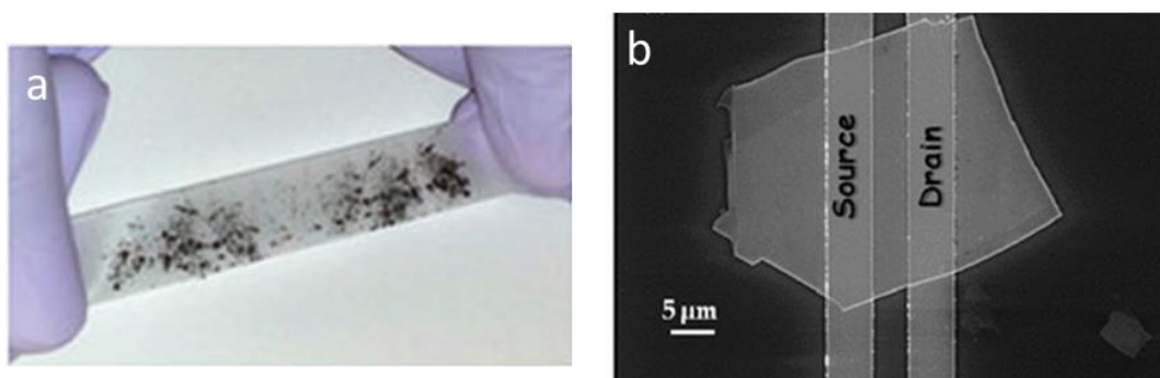
Figure I-8 : Feuillets de MoS 2 exfoliés sur ruban adhésif (a) ou intégrés dans un dispositif (b) [19], [20].
