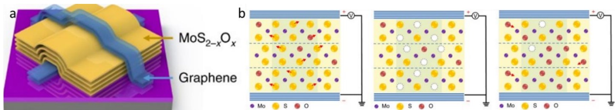
Figure I-21 : a : Schéma des dispositifs étudiés , b : schéma du mécanisme de commutation [43].
