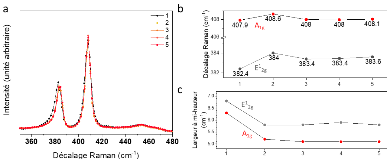
Figure III-14 : Analyses Raman à différentes étapes du procédé. Superposition des différents spectres acquis (a) et évolution de la position (b) et de la largeur à mi-hauteur (c) des deux modes E_{2g}^1 et A_{1g} .
