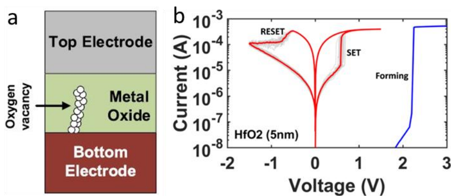
Figure I-14 : OxRAM, à gauche : schéma du dispositif (a) , cycle de SET et RESET typique d'une mémoire résistive de type OxRAM à base de HfO 2 (b) avec tracé du premier cycle ou forming en bleu et des suivants avec les commutations OFF vers ON : set et ON vers OFF : reset [[32], [33]].
