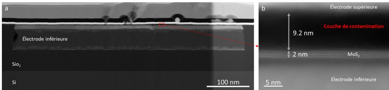
Figure III-9 : Image obtenue en TEM des premiers circuits réalisés. (a) Image de l'empilement complet, (b) Image à plus fort grossissement montrant le film de MoS 2 et ses interfaces avec les électrodes inférieure et supérieure.
