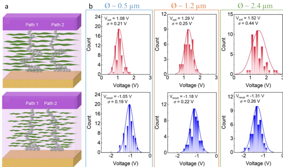
Figure IV-10 : Schémas et graphiques issus de [44]. a : schématisation des filaments conducteurs formés pour des nanofeuillets de différentes tailles, b : distribution des tensions de commutation pour différents diamètres de nanofeuillets.
