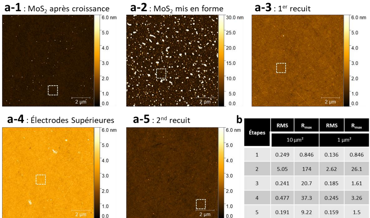
Figure III-16 : Scans AFM réalisés sur une zone propre de MoS 2 à différentes étapes de l'intégration (a-1 à a-5). b : rugosité moyenne (RMS) et maximale (R max ) des différents scans AFM, sur une zone de 10 μm 2 (scan entier) ou 1 μm 2 (zone propre délimitée par les encadrés blancs en pointillés).
