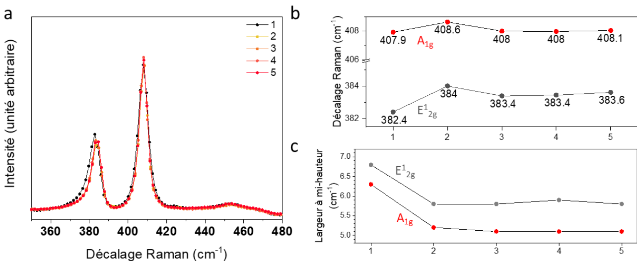
Figure III-14 : Analyses Raman à différentes étapes du procédé. Superposition des différents spectres acquis (a) et évolution de la position (b) et de la largeur à mi-hauteur (c) des deux modes E 2g 1 et A 1g .
