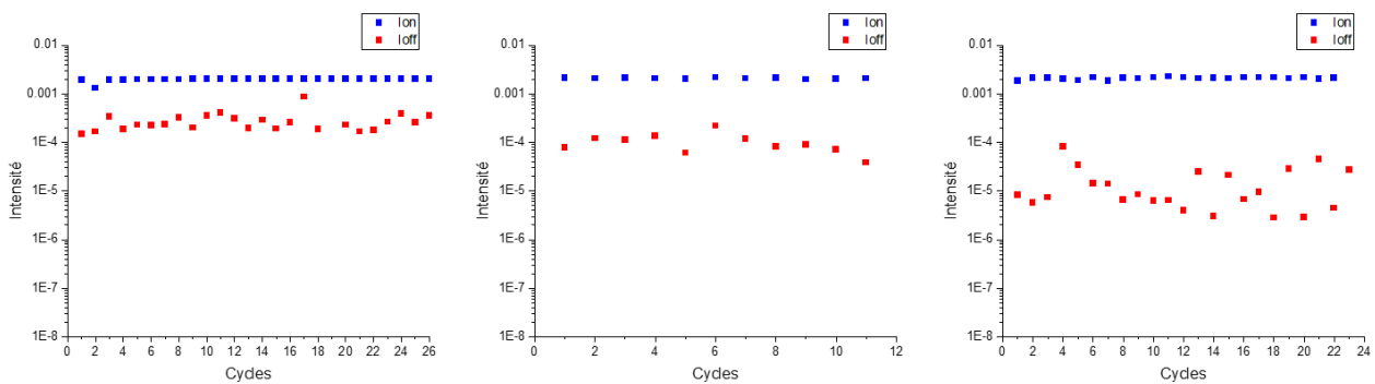
Figure IV-27 : Variation du courant mesuré (pour une tension de 100 mV) dans chacun des états ON et OFF au cours des cycles pour trois dispositifs de l'échantillon n°2 (CVD multicouches).
