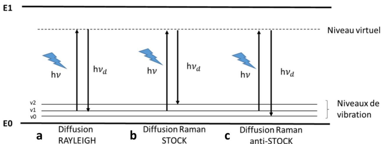
Figure II-1 : Schéma des trois types de désexcitation de l'énergie photonique, issu de la référence [27].
