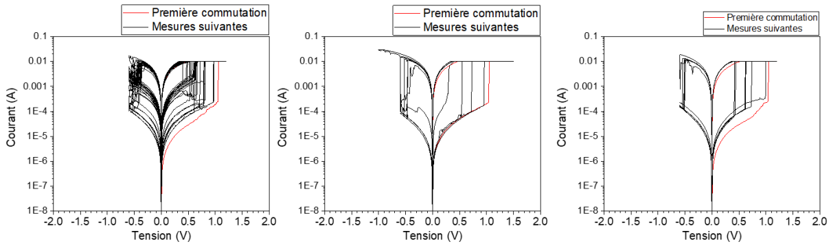
Figure IV-23 : Caractéristiques courant-tension de trois dispositifs de l'échantillon n°3.
