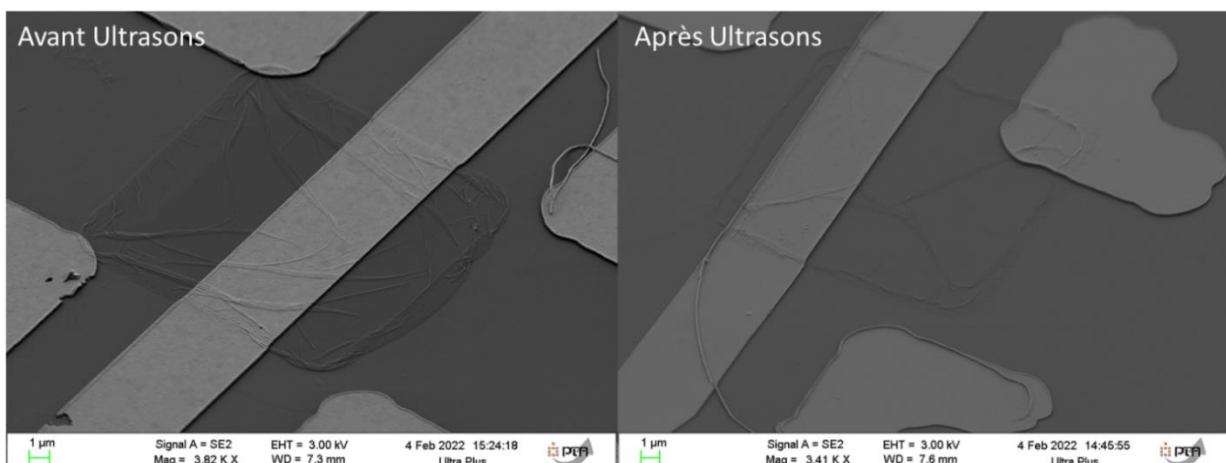
Figure III-23 : image MEB de dispositifs type mémoire avant puis après l'utilisation d'ultrasons.
