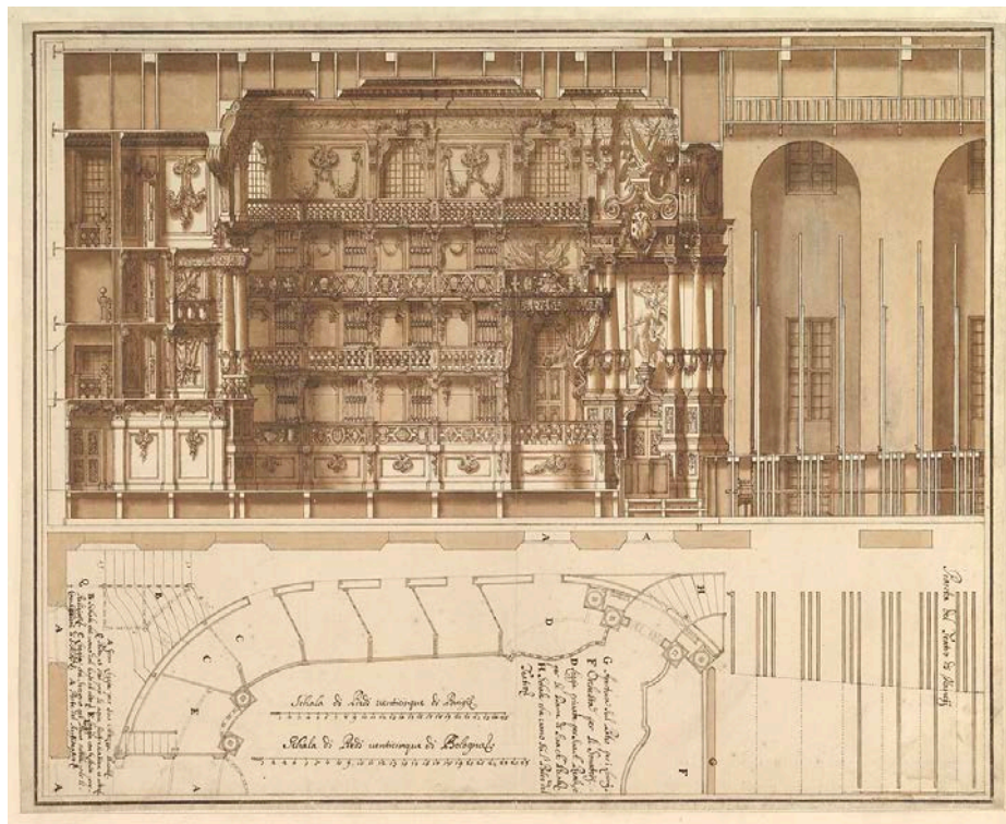
Fig. 55 : Francesco Bibiena, Coupe longitudinale et demi-plan pour le projet de l'opéra de Nancy, crayon et encre brune avec lavis, 413 x 513 mm, 1709, New-York, MET, c°1972.713.61 © MET
