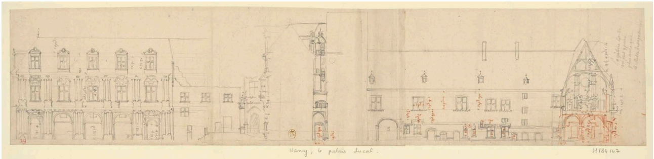
Fig. 24 : Anonyme (probablement agence Hardouin-Mansart), Le palais ducal de Nancy, élévation septentrionale de l'aile sud de la cour d'honneur et de l'aile sud donnant sur le jardin, 157 x 730 mm, crayon noir et sanguine sur papier, 1700, BnF, département des estampes et photographie, c°HA-18 (A, 9)-FT 4 © BnF
