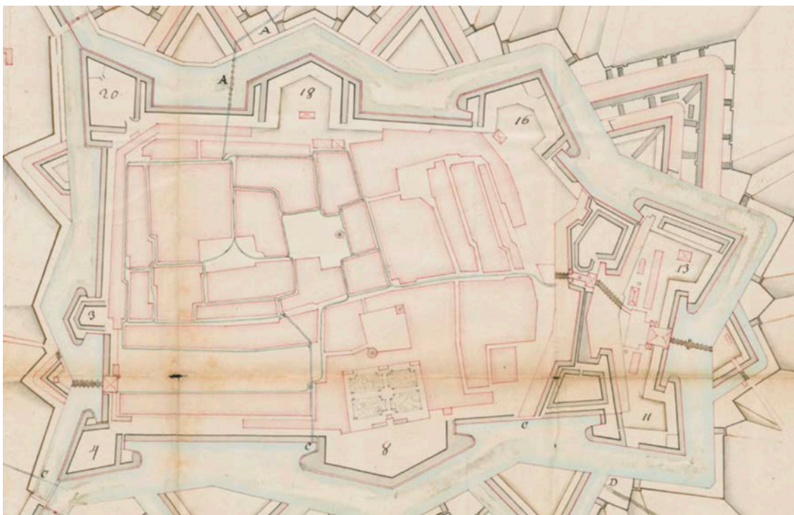
Fig. 20 : Anonyme, Plan des Villes et Citadelle de Nancy , détail de la ville vieille, 1696, Vincennes, SHD 1 VH 1238, Art 8, Sect. 1 carton 1, n° 3 © SHD.
