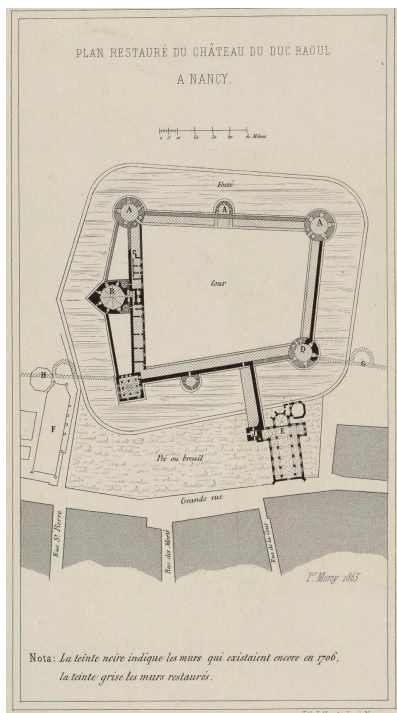
Fig. 51-52 : Reconstitution en plan et en élévation du château médiéval des ducs de Lorraine à Nancy sous le règne du duc Raoul, Prosper Morey et Louis Christophe, lithographie, d'après Prosper Morey 1865, p. 175-176
