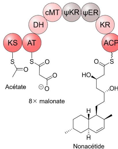
Figure 24: Voies de biosynthèse de l'aflatoxine B 1 , de la 6-MSA et de la lovastatine impliquant une NR-, PR- et HR-iPKS, respectivement (d'après Weissman, 2010 160 et Wang et al., 2021 162 ). Les réactions de cyclisation sont indiquées par une flèche de la couleur des domaines qui les catalysent. Les domaines colorés en gris sont inactifs (ΨKR, ΨER) ou leur rôle est inconnu (C).
