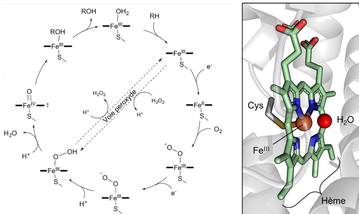
Figure 51 : Cycle catalytique des CYP lors de l'hydroxylation du substrat (à gauche) et structure de l'hème (à droite). La voie peroxyde permet la formation de l'intermédiaire hydroperoxy-ferrique à partir de \text{Fe}^{\text{III}} en présence de l'enzyme et en réagissant avec une molécule de peroxyde d'hydrogène (figure reproduite de Rudolf et al. , 2017 296 ). La structure cristallographique de la CYP AbyV impliquée dans la biosynthèse de l'abyssomicine C
