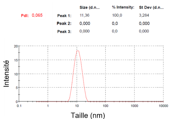
Figure 74 : Résultats de DLS de OocM (à gauche) et de LbmA-Ox-ACP (à droite) permettant la comparaison des paramètres calculés. La détection d'un seul pic responsable de 100 % de l'intensité diffusée atteste de la pureté de l'échantillon. De plus, l'indice de polydispersité (Pdl) est inférieur à 10 %, ce qui indique une bonne homogénéité de l'échantillon. Les deux constructions présentent un diamètre hydrodynamique de taille comparable, bien que le didomaine monomérique LbmA-Ox-ACP soit 60 % plus massif qu'OocM. Cela témoigne de l'homodimérisation d'OocM en solution.
