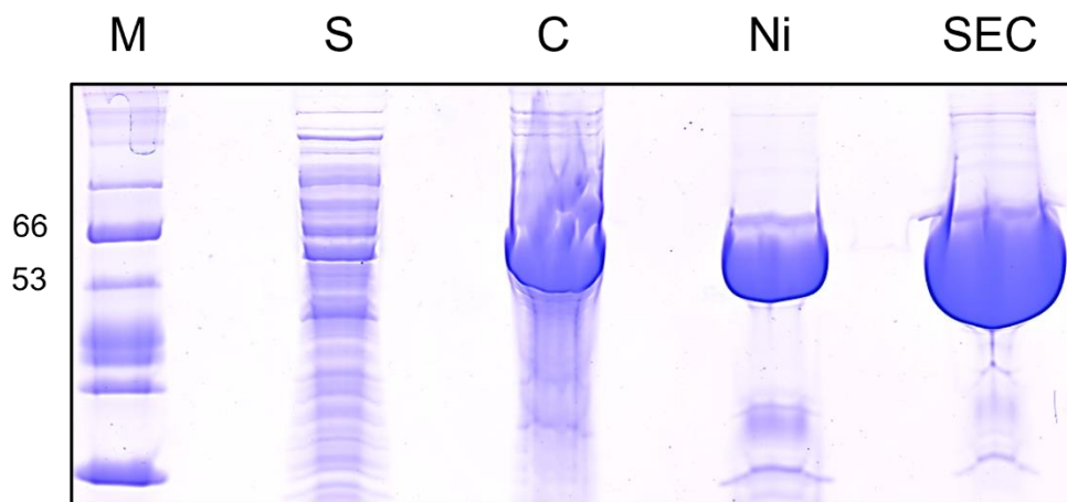
Figure 66: SDS-PAGE bilan de purification de SUMO-SbnP. La pureté de l'échantillon a été évaluée dans le surnageant (S) et le culot (C) de centrifugation après lyse des cellules et dans l'éluat des colonnes de chromatographie d'affinité nickel (Ni) et d'exclusion de taille (SEC). Le protocole mis en place a permis la purification de la BVMO, bien que des impuretés subsistent. Les rendements obtenus sont de 11,61 mg de BVMO par litre de culture. Les bandes du marqueur de taille (M) correspondant aux masses de 53 et 66 kDa sont indiquées. SUMO-SbnP possède une masse moléculaire de 63 kDa.
